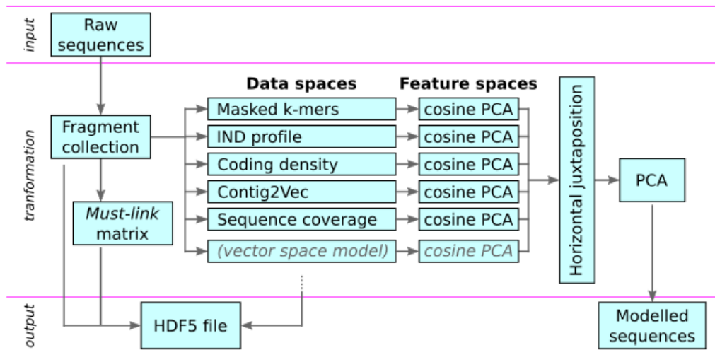
FIGURE 4.1 | Worklow général de fennec pour la modélisation non supervisée de séquences métagénomiques.
