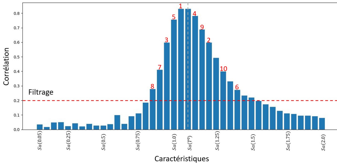
Figure 3.20 - [Coulomb] Application de la méthode hybride
