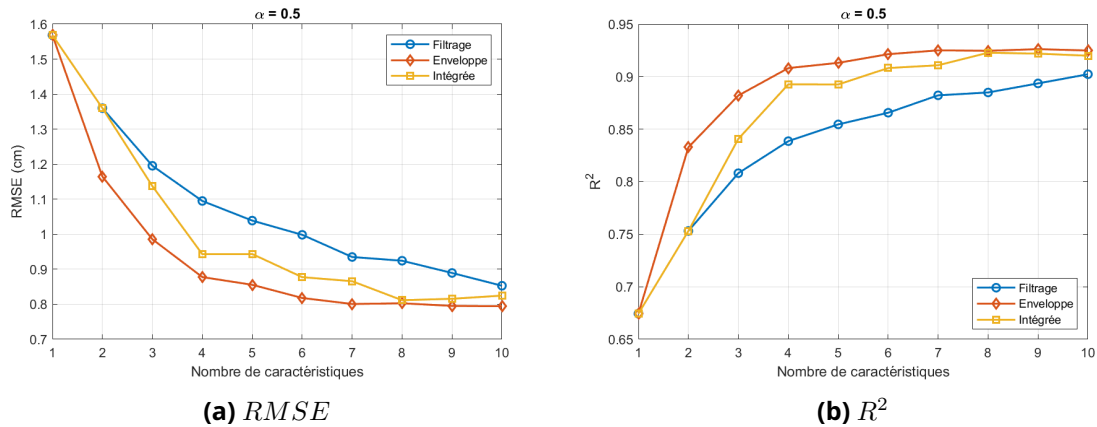
Figure 3.15 – [ \alpha = 0.5 ] Évolution de RMSE et R^2 des méthodes de sélection
