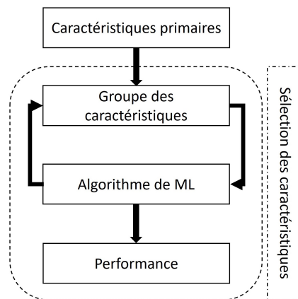
Figure 3.9 – Procédure de sélection des caractéristiques par la méthode intégrée
