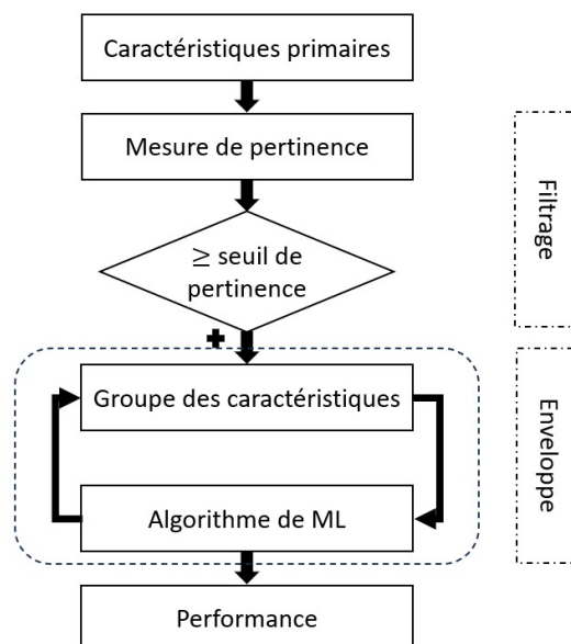
Figure 3.18 – Procédure de sélection des caractéristiques par la méthode hybride
