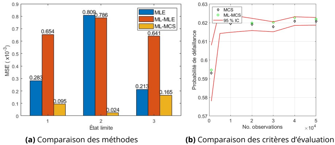
Figure 3.27 – [Bouc-Wen] Comparaisons des méthodes de construction de la courbe
