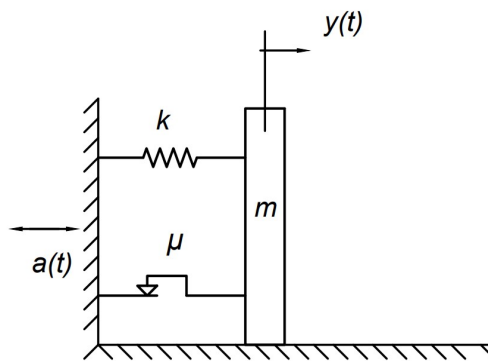
Figure 3.1 – Oscillateur non-linéaire de Coulomb
