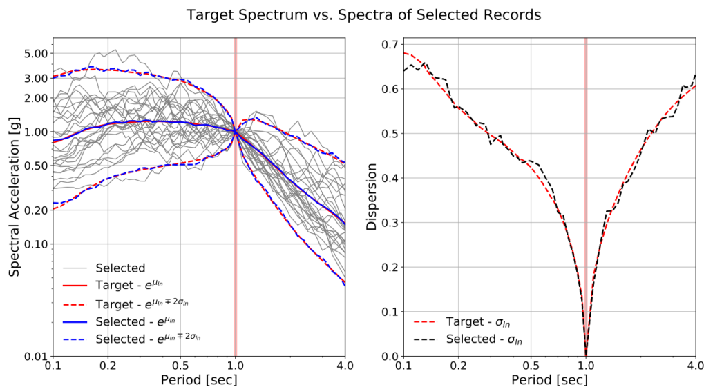
Figure 4.1 – Spectres des enregistrements sélectionnés par EzGM
