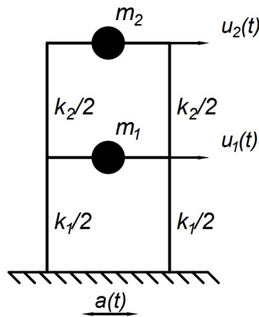
Figure 2.11 – Structure à deux degrés de liberté
