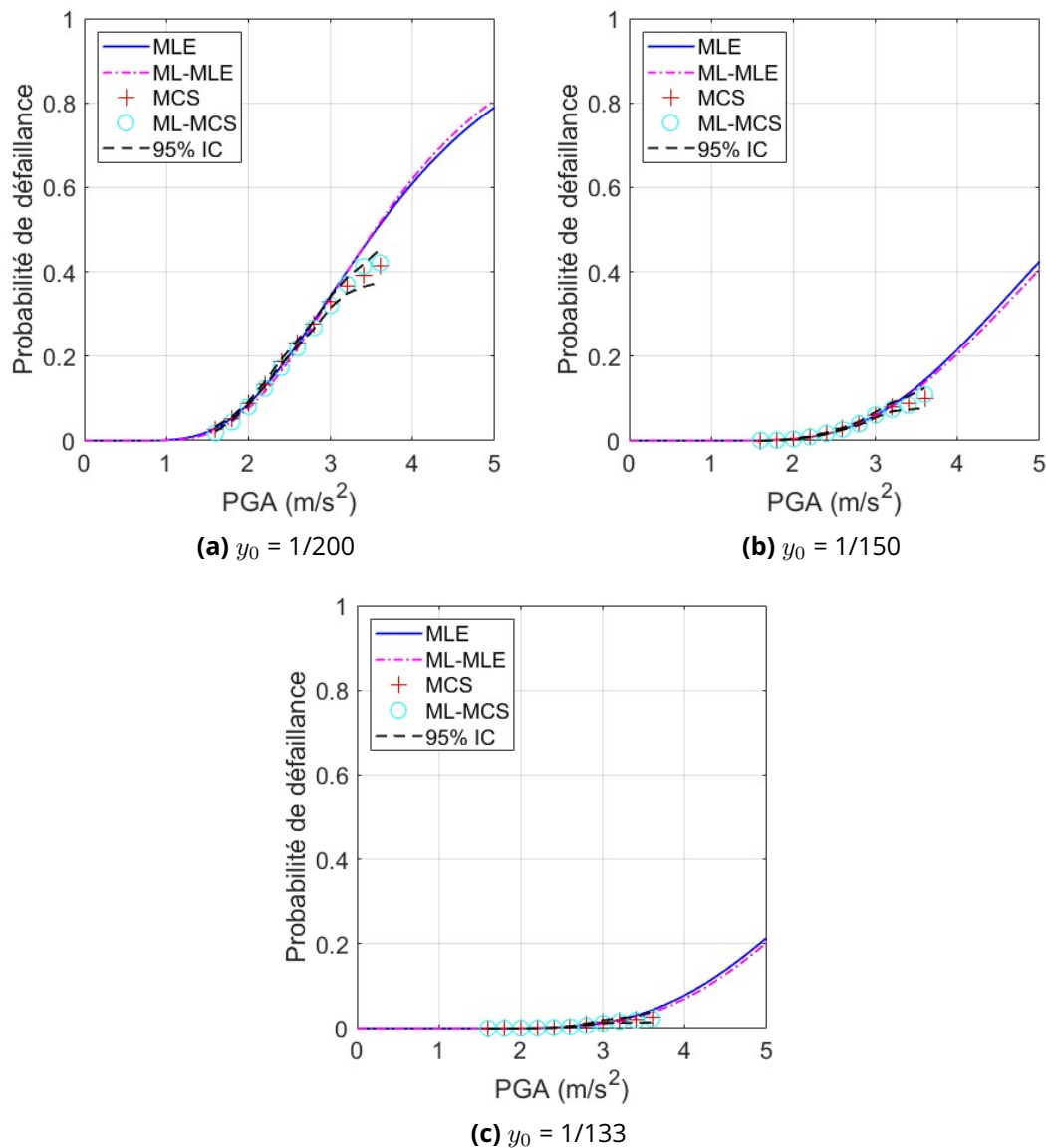
Figure 3.32 – [Bouc-Wen 8ddl] Courbes de fragilité par différentes méthodes
