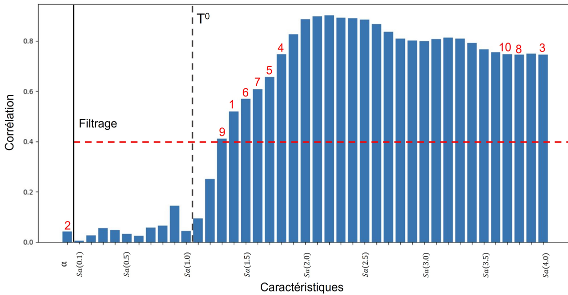
Figure 4.13 – Sélection des caractéristiques par méthode hybride
