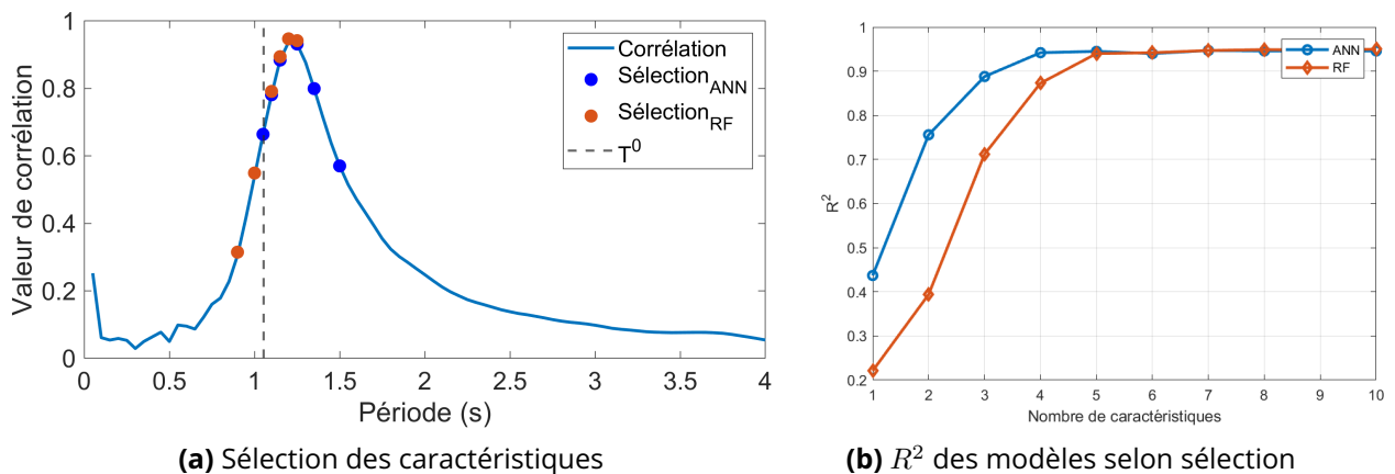
Figure 3.11 – [Enveloppe] Sélection par la méthode de filtrage
