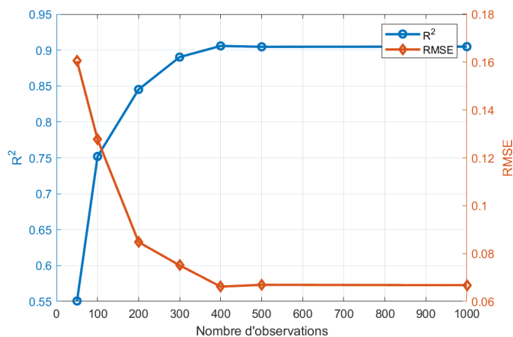
Figure 4.5 – [Coulomb] Évolution des métriques selon le nombre d'observations
