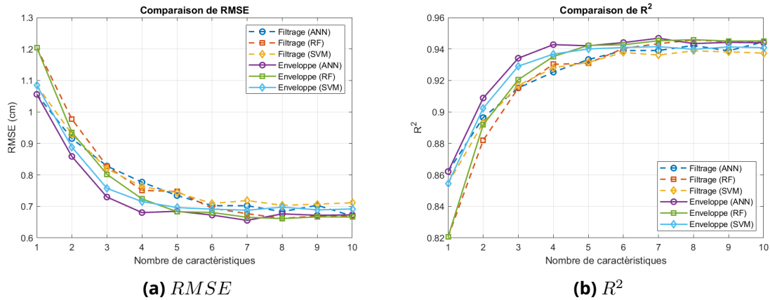
Figure 3.14 – Évolution de RMSE et R^2 selon les méthodes de sélections et les modèles de ML
