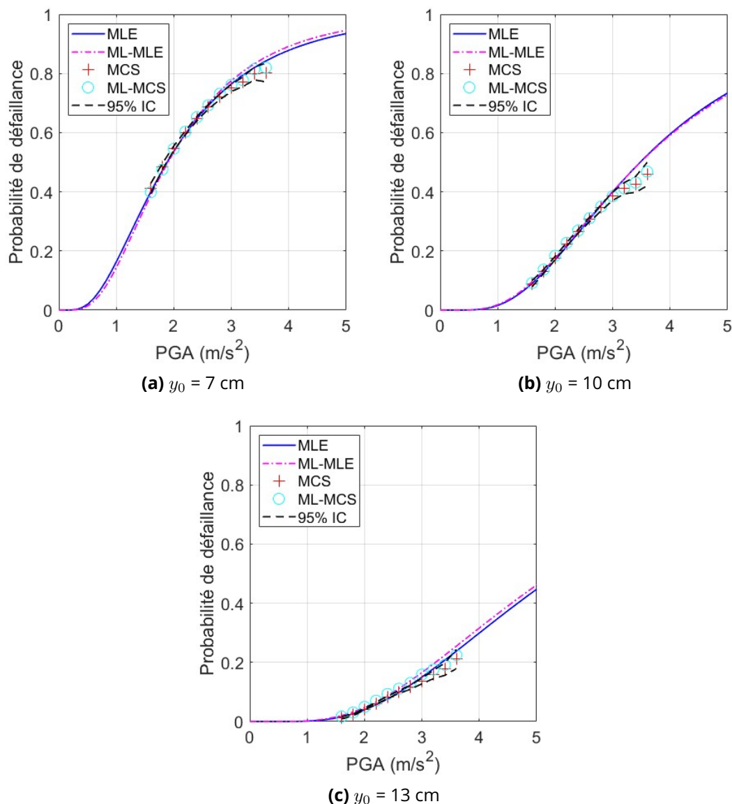
Figure 3.26 - [Bouc-Wen] Courbes de fragilité par différentes méthodes
