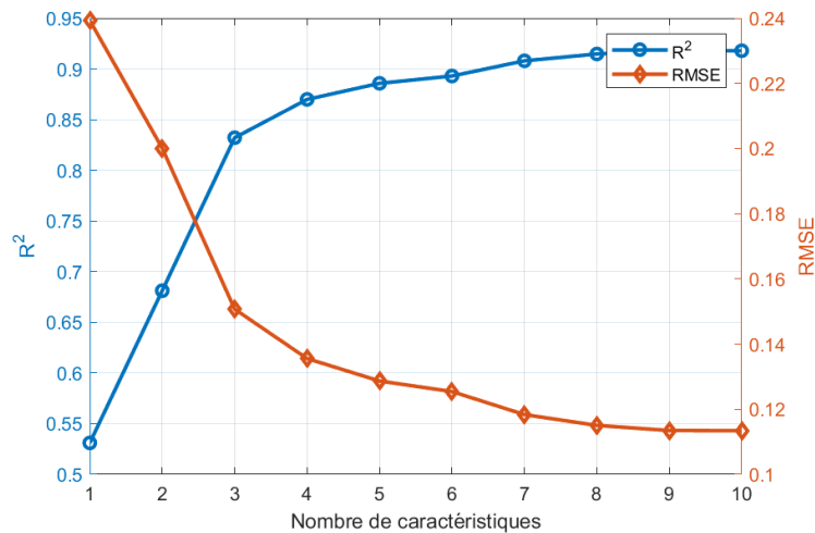
Figure 4.9 – [Bouc-Wen] Évolution des métriques selon le nombre de caractéristiques
