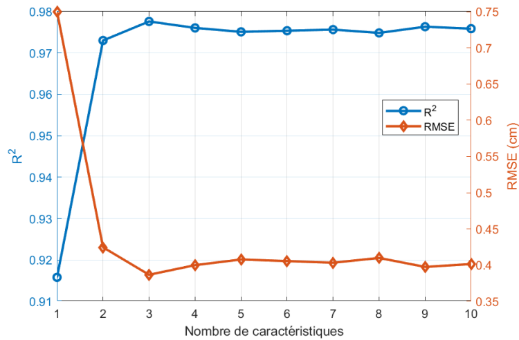
Figure 4.14 – Évolution des métriques selon le nombre de caractéristiques
