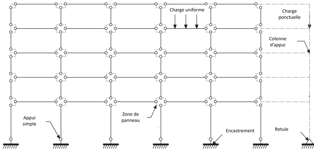
Figure 5.7 - Modèle numérique non-linéaire d'un portique à cinq étages et cinq travées
