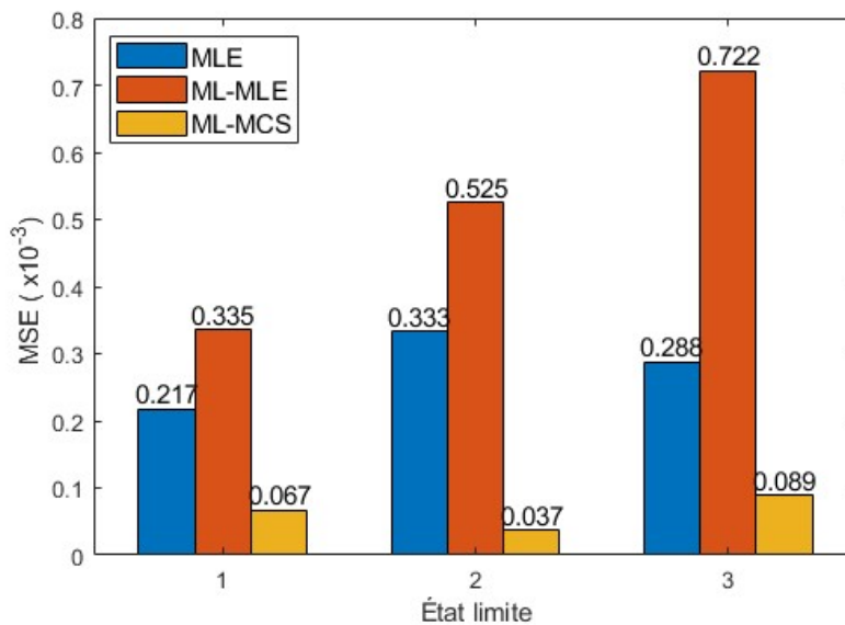
Figure 2.10 – [1ddl] Critère de comparaison pour trois états limites
