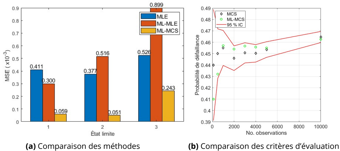
Figure 3.23 – [Coulomb] Comparaisons des méthodes de construction de la courbe
