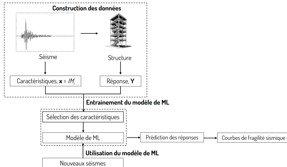
Figure 1.15 – Procédure de construction de la courbe de fragilité basé sur l'apprentissage automatique
