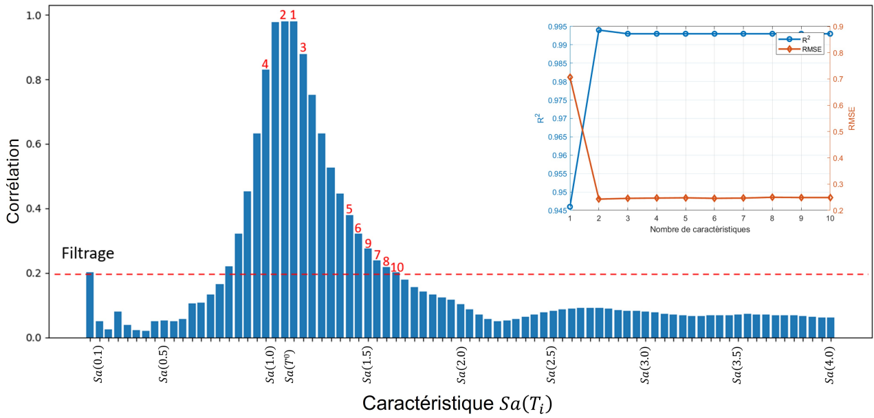
Figure 3.33 – [Bouc-Wen] Sélection pour \alpha = 0.9
