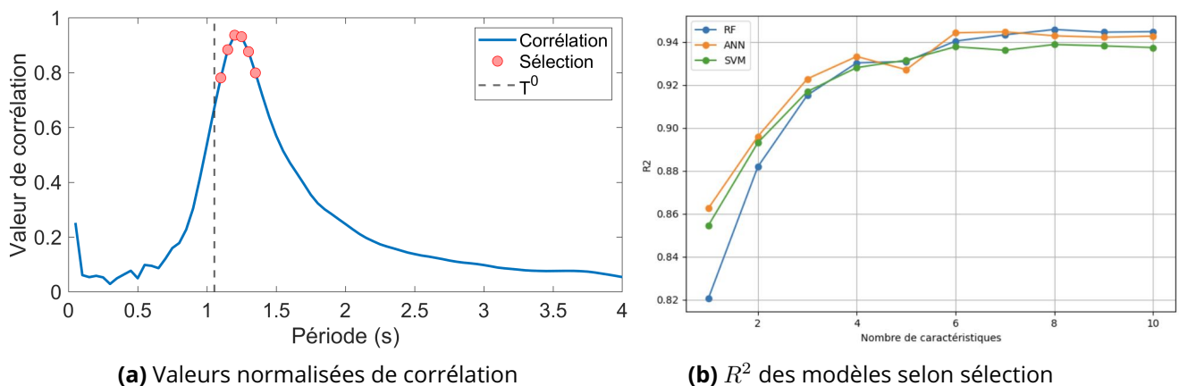
Figure 3.10 – [Filtrage] Sélection par la méthode de filtrage
