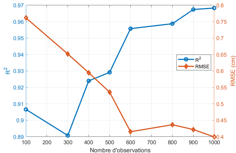
Figure 4.12 – Évolution du modèle selon le nombre d'observations
