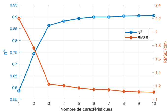
Figure 3.21 - [Coulomb] Évolution des métriques d'évaluation selon le nombre de caractéristiques
