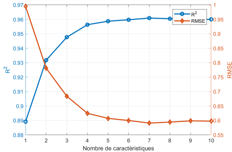
Figure 3.25 – [Bouc-Wen] Évolution des métriques d'évaluation selon le nombre de caractéristiques
