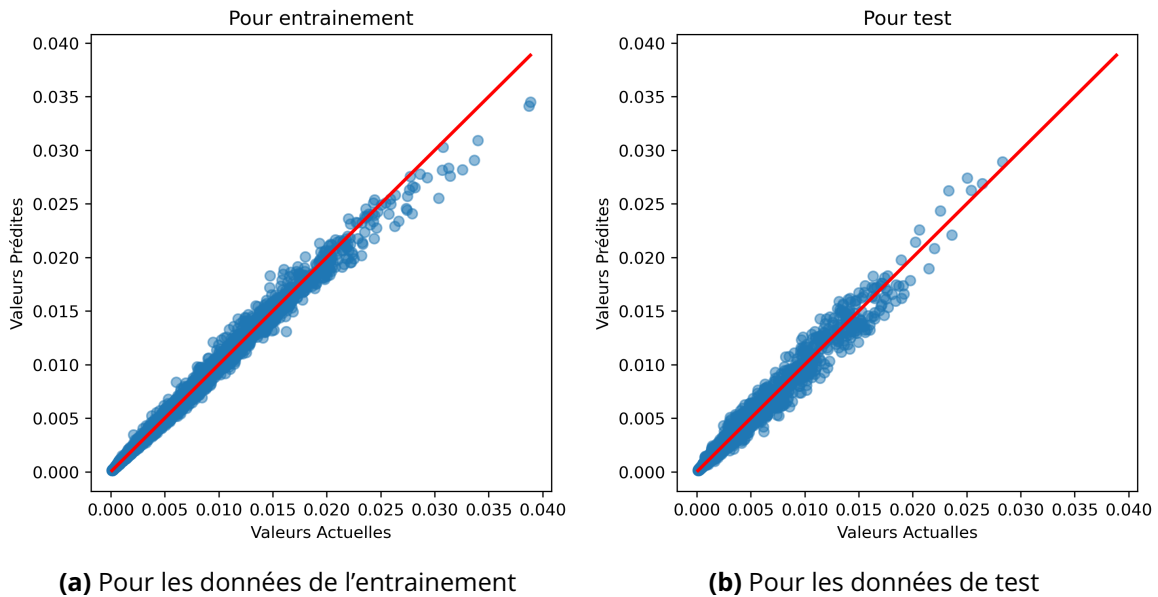
Figure 5.17 – [Plusieurs étages] Comparaison entre les valeurs prédites et les valeurs simulées
