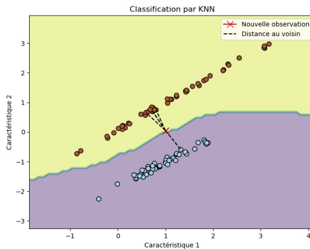
Figure 1.4 – Exemple d'un modèle KNN
