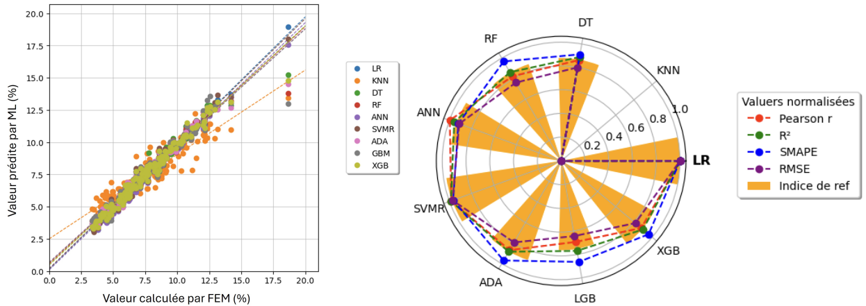
(a) Comparaison des valeurs prédites et actuelles (b) Comparaison des métriques d'évaluation
