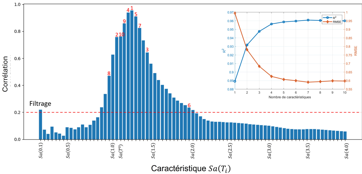
Figure 3.35 - [Bouc-Wen] Sélection pour \alpha = 0.7
