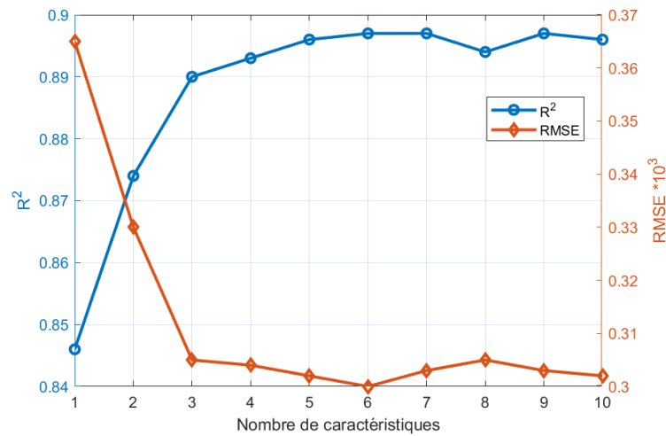
Figure 3.30 – [Bouc-Wen 8ddl] Évolution des métriques d'évaluation selon le nombre de caractéristiques
