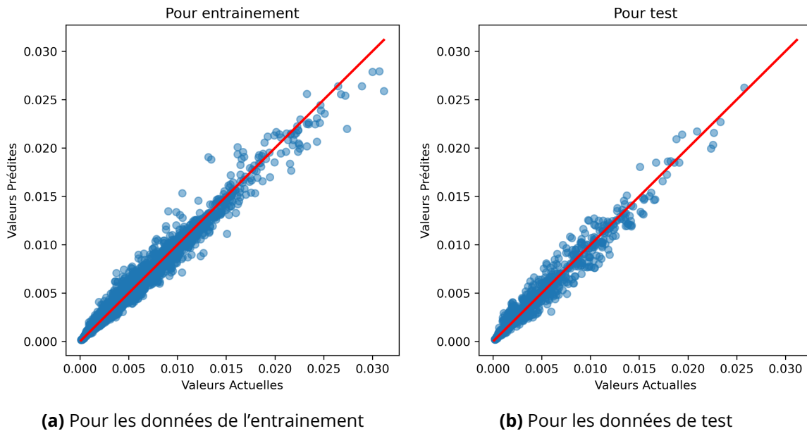
Figure 5.13 – [1 étage] Comparaison entre les valeurs prédites par modèle RF et les valeurs actuelles obtenues par éléments finis
