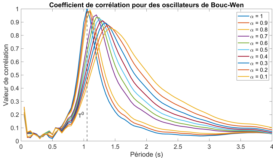
Figure 3.4 – [Bouc-Wen] Coefficient de corrélation par rapport à \alpha
