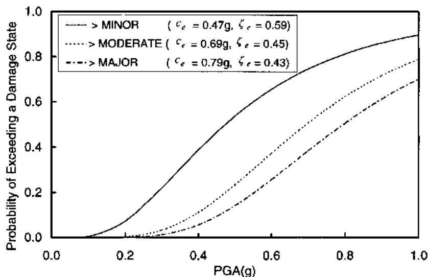
Figure 1.1 – Courbes de fragilité sismique selon PGA [8]
