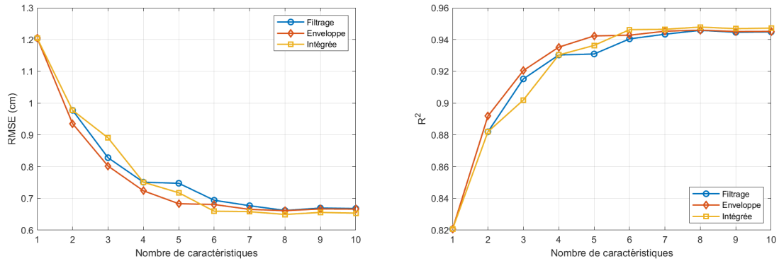
(a) Forêt aléatoire
