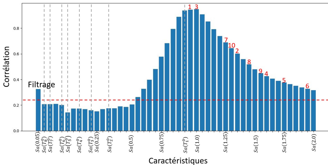
Figure 3.29 – [Bouc-Wen 8ddl] Application de la méthode hybride
