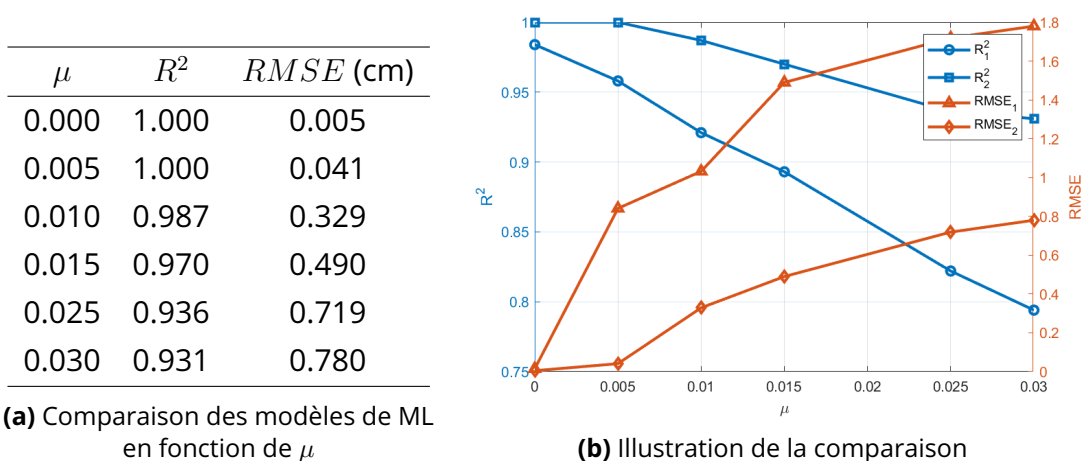
Figure 3.5 – [Coulomb] Influence de \mu et du nombre de caractéristiques
