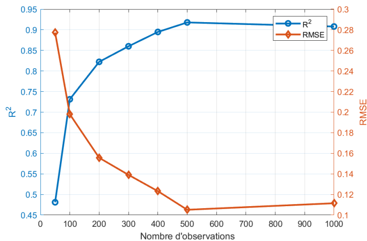
Figure 4.8 – [Bouc-Wen] Évolution des métriques selon le nombre d'observations
