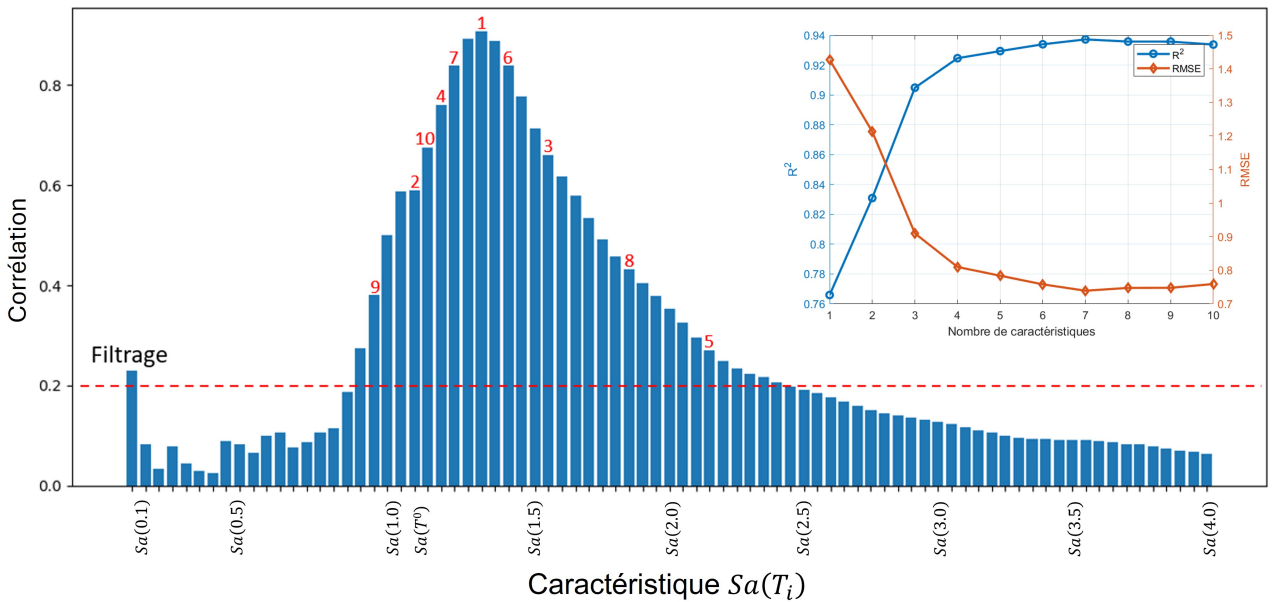
Figure 3.38 – [Bouc-Wen] Sélection pour \alpha = 0.4
