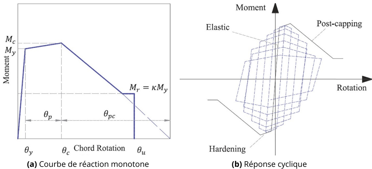
Figure 5.8 - Modèle de matériaux IMK modifié [127]
