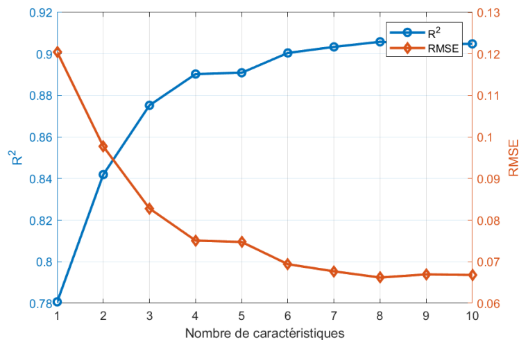
Figure 4.6 – [Coulomb] Évolution des métriques selon le nombre de caractéristiques
