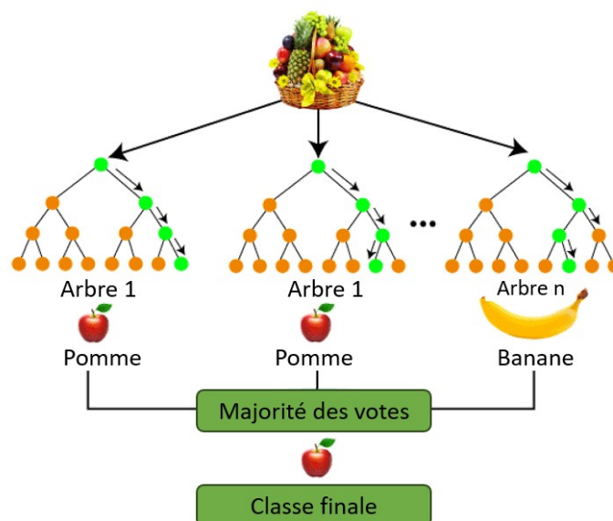
Figure 1.8 – Exemple d’une forêt aléatoire
