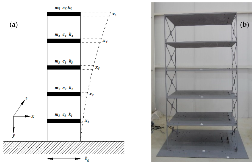
Figure 5.2 – (a) Modèle mécanique de la structure et (b) sa maquette
