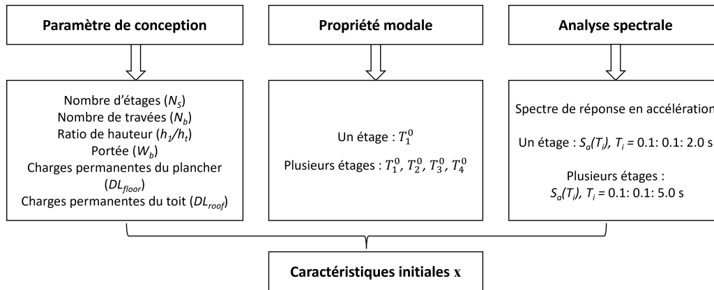
Figure 5.10 – Description de l’ensemble des caractéristiques x
