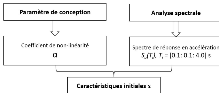
Figure 4.11 – Caractéristiques initiales \mathbf{x} pour les oscillateurs de Bouc-Wen
