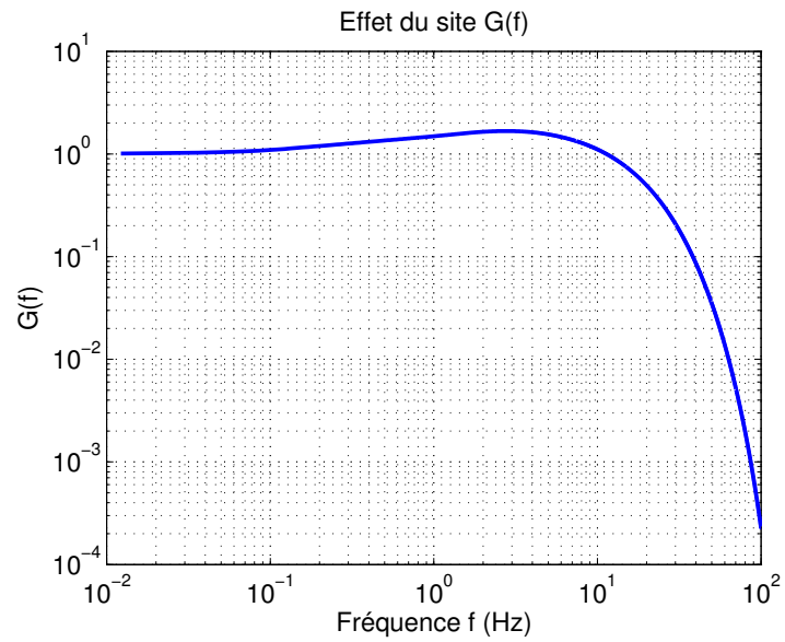
Figure A.3 - Influence de l'effet du site
