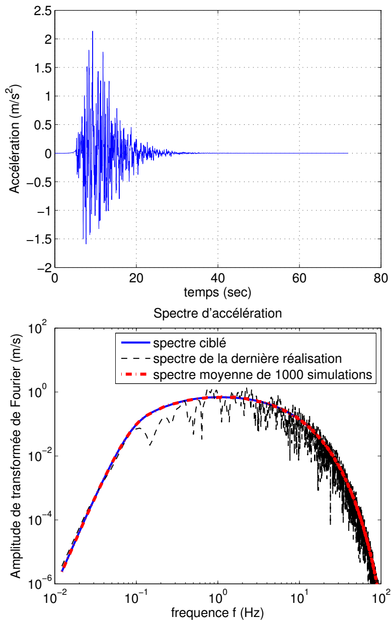
Figure 1.18 – Une simulation de séisme par le modèle de Boore
