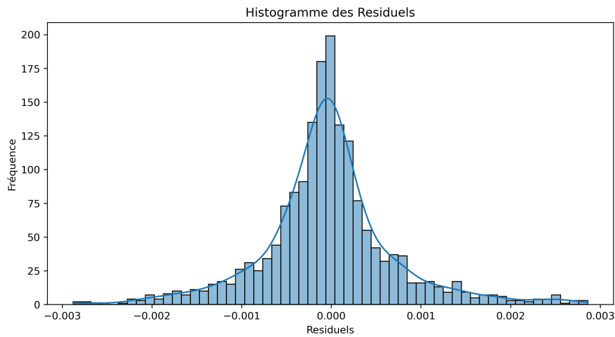
Figure 5.18 – [Plusieurs étages] Histogramme des écarts
