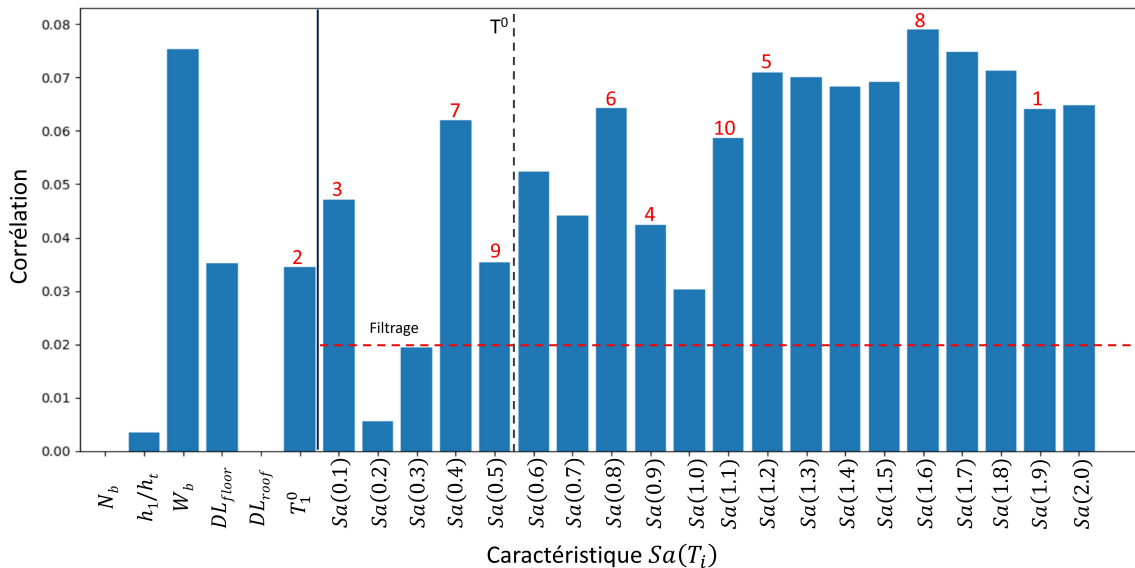
Figure 5.11 – [1 étage] Ordre de sélection des caractéristiques S_a(T_i)
