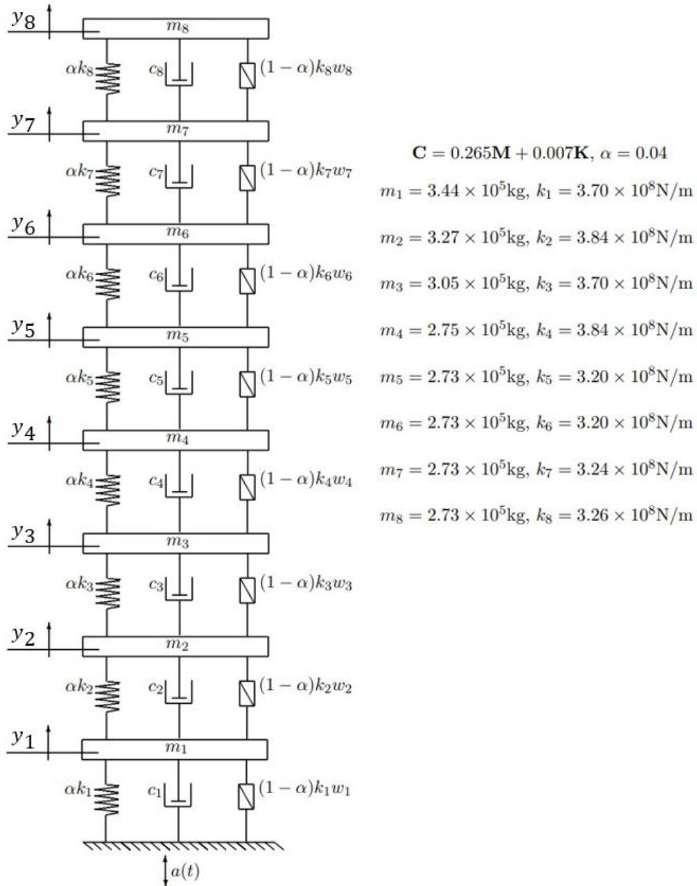
Figure 3.28 – Structure à huit degrés de liberté non-linéaire de Bouc-Wen
