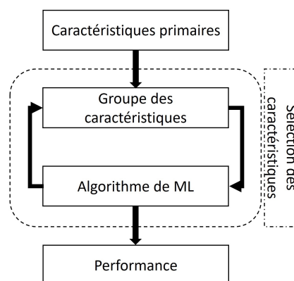
Figure 3.8 – Procédure de sélection des caractéristiques par la méthode d'enveloppe
