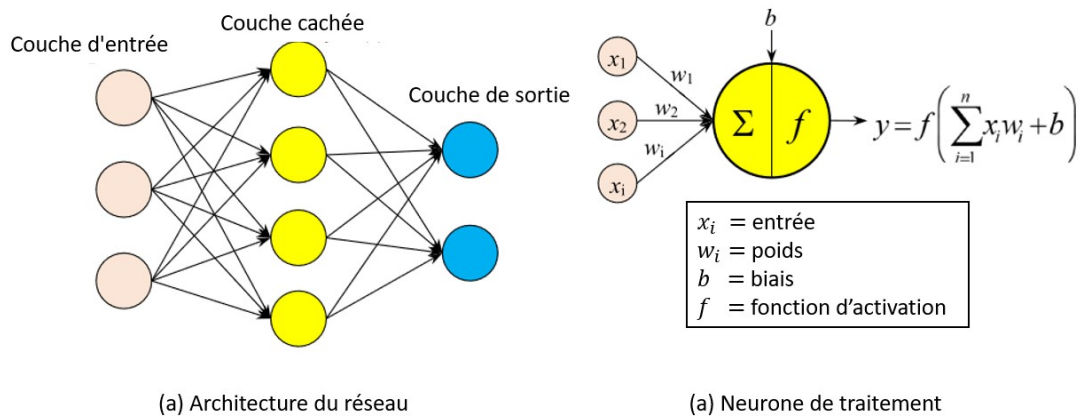
Figure 1.9 – Exemple d'un réseau de neurones
