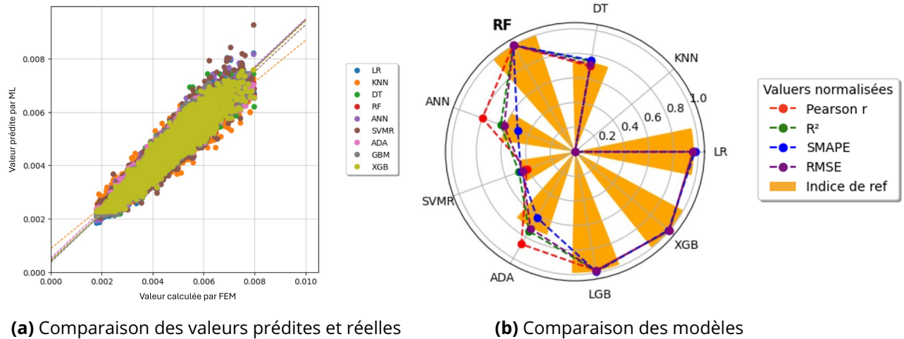
Figure 3.31 – [Bouc-Wen 8ddl] Comparaisons des modèles de machine learning
