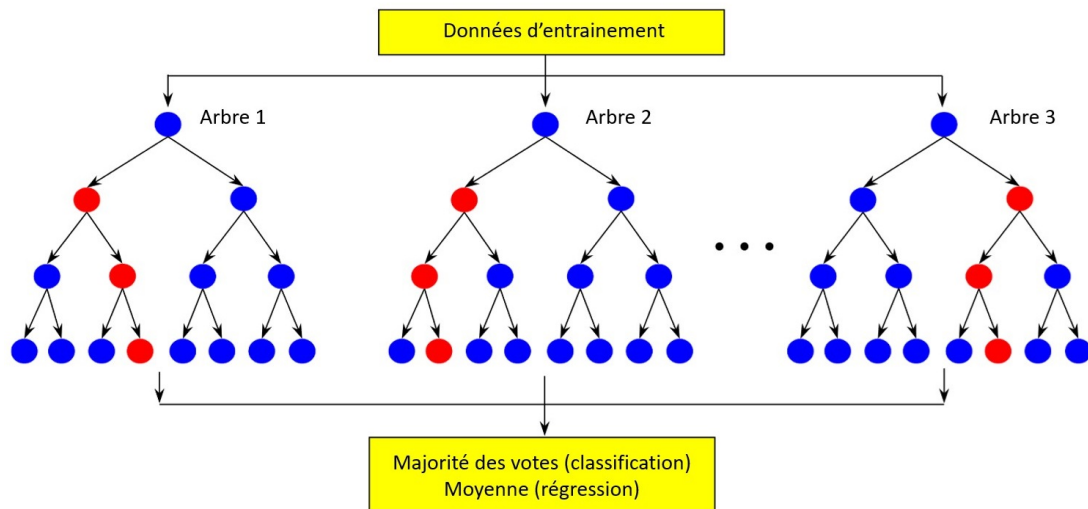
Figure 1.7 – Illustration d’algorithme d’une forêt aléatoire
