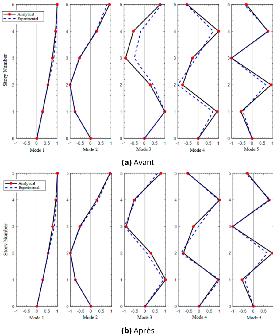
Figure 5.3 – Comparaison de la déformée modale entre le modèle et la maquette [129]
