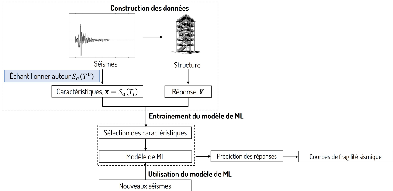
Figure 2.3 – [PRO-LIN] Procédure de l'application de ML pour des structures linéaires
