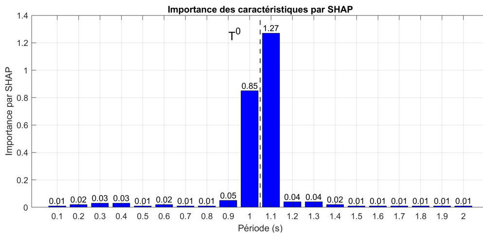
Figure 2.8 – [1ddl] Importance des caractéristiques par une étude de SHAP
