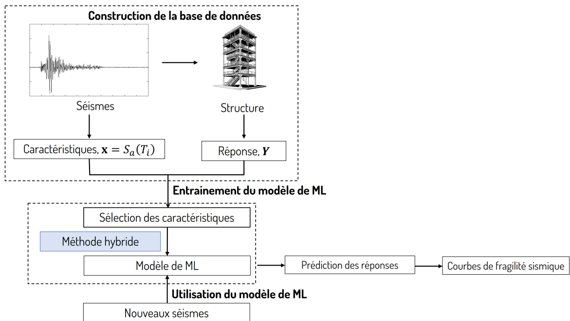
Figure 3.19 – [PRO-NONLIN] Procédure de l'application de ML pour des structures non-linéaires
