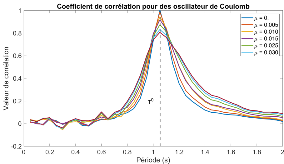
Figure 3.3 – [Coulomb] Coefficient de corrélation par rapport à \mu
