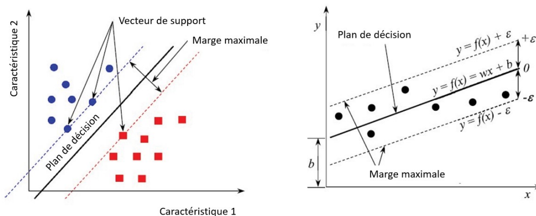
Figure 1.10 – Exemple d'une machine à vecteur de support pour classification et régression
