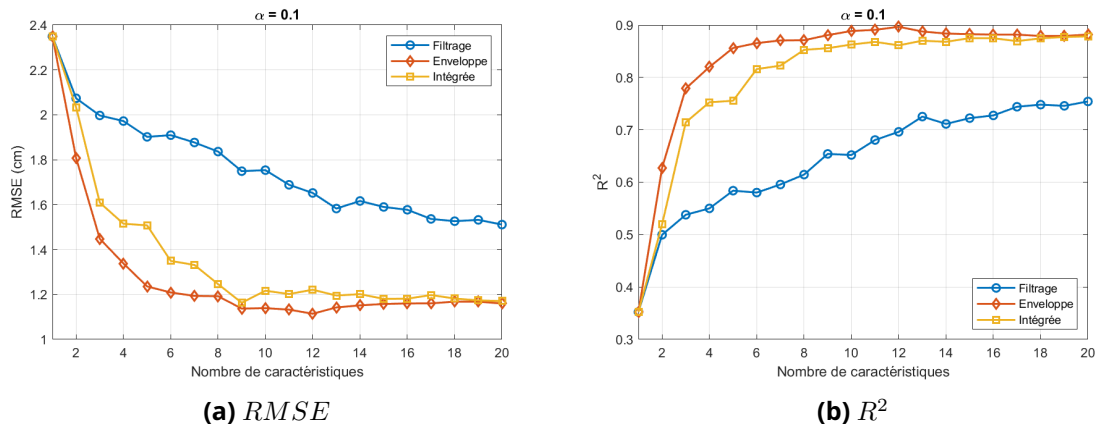
Figure 3.17 – [ \alpha = 0.1 ] Évolution de RMSE et R^2 des méthodes de sélection
