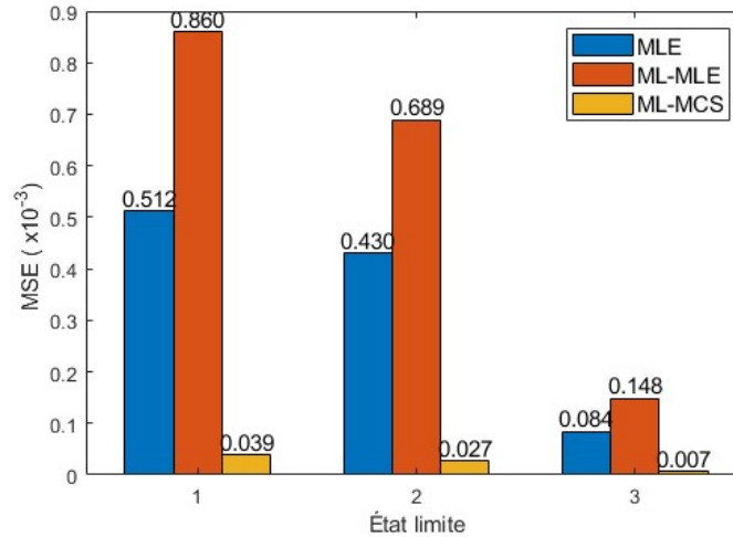
Figure 2.17 – [2ddl] Critère de comparaison pour trois états limites
