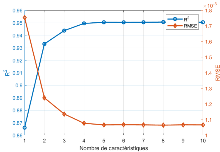
Figure 5.16 – [Plusieurs étages] Évolution des métriques selon le nombre de caractéristiques
