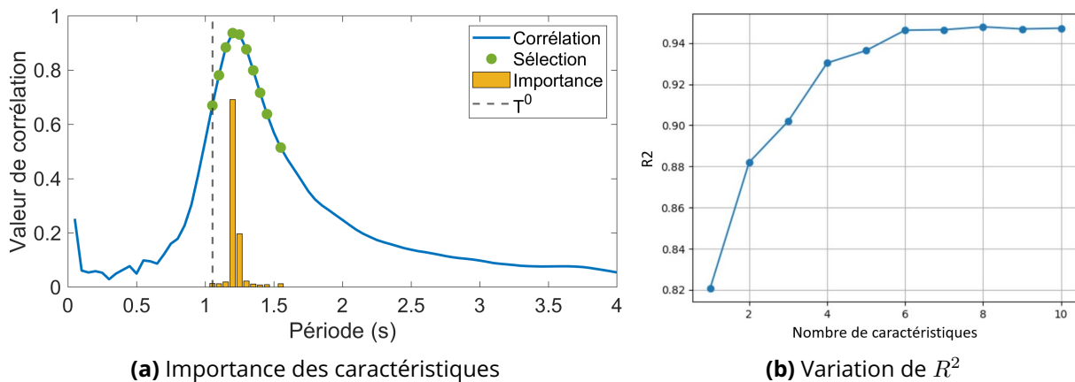
Figure 3.12 - [Intégrée] Résultat de la sélection des caractéristiques récursive
