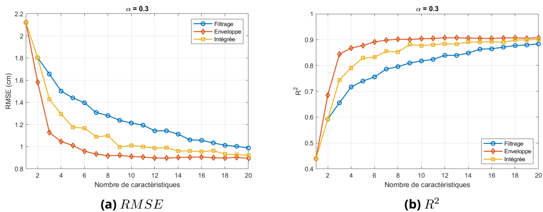
Figure 3.16 – [ \alpha = 0.3 ] Évolution de RMSE et R^2 des méthodes de sélection
