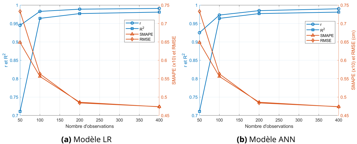
Figure 2.7 – [1ddl] Influence du nombre d'observations
