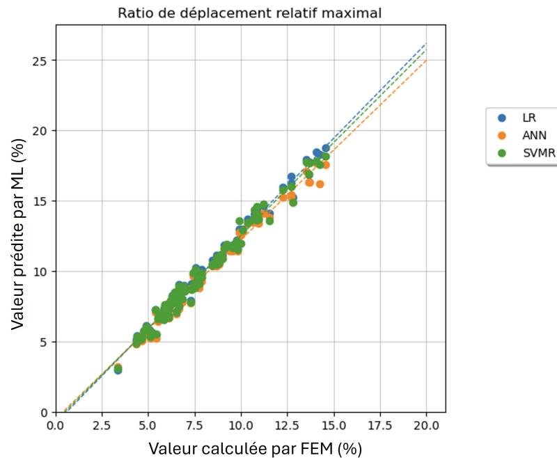
Figure 5.5 - [Maquette] Comparaison des valeurs prédites et actuelles
