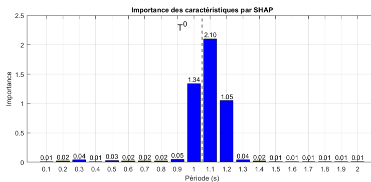
Figure 4.4 – [Linéaire] Contribution des caractéristiques selon l'étude de SHAP
