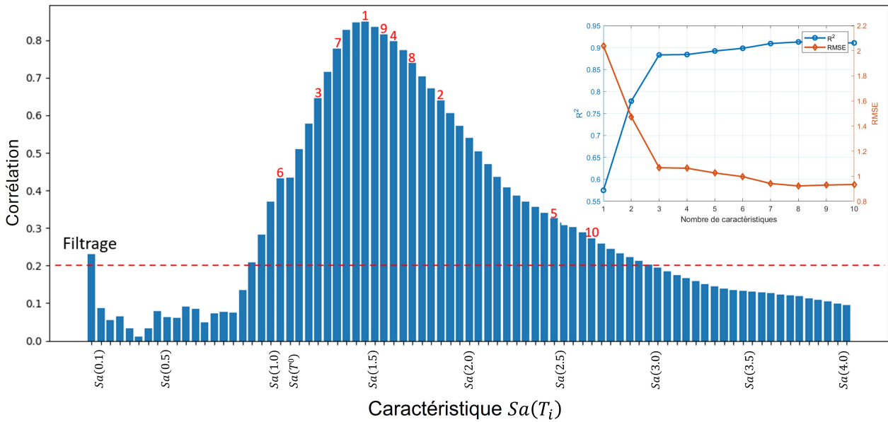
Figure 3.41 – [Bouc-Wen] Sélection pour \alpha = 0.1
