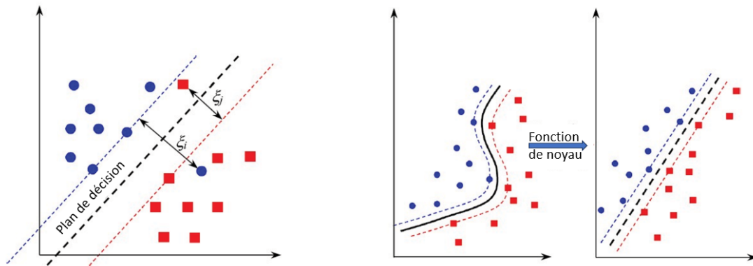
Figure 1.11 – Illustration de paramètre de pénalty \xi et la fonction de noyau
