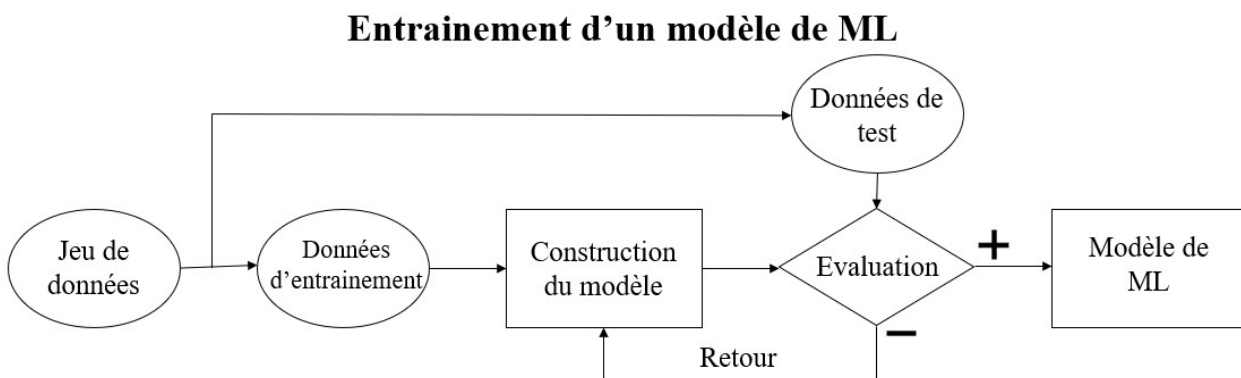
Figure 1.13 – Procédure typique d'entraînement un modèle d'apprentissage automatique
