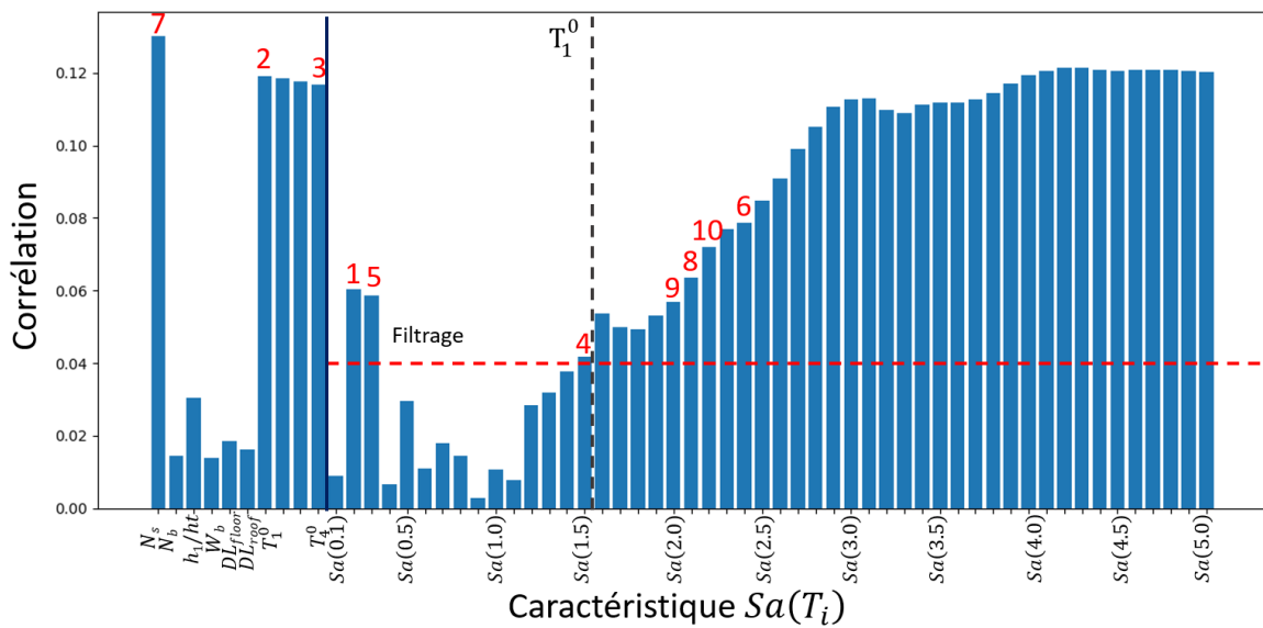
Figure 5.15 – [Plusieurs étages] Ordre de sélection des caractéristiques
