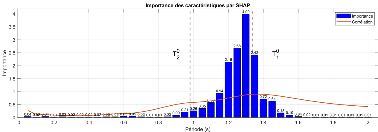
Figure 2.15 – [2ddl] Valeurs SHAP des caractéristiques du spectre de réponse en accélération
