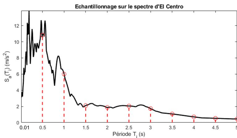
Figure 2.5 – [1ddl] Échantillonnage initiale du spectre de réponse en accélération moyenne
