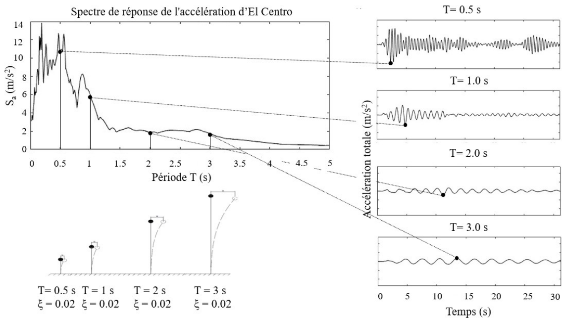
Figure 1.16 – Spectre de réponse d'accélération totale pour le séisme d'El Centro
