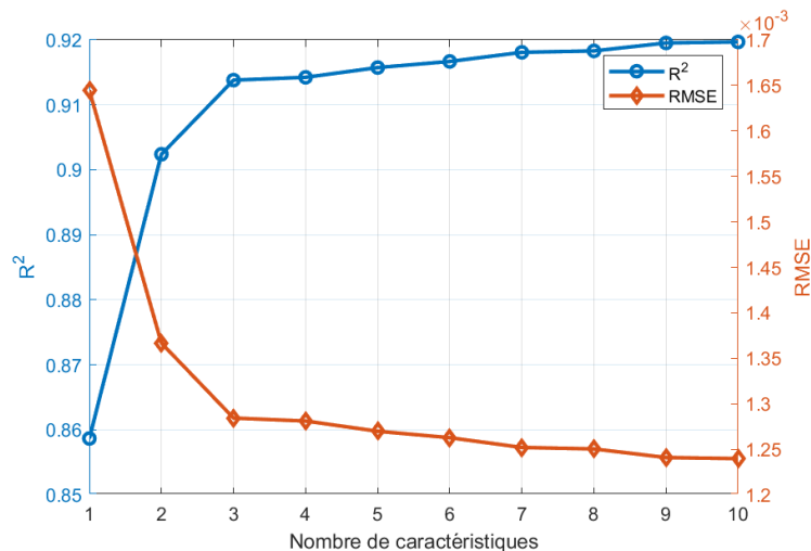
Figure 5.12 – [1 étage] Évolution des métriques d'évaluation selon le nombre de caractéristiques
