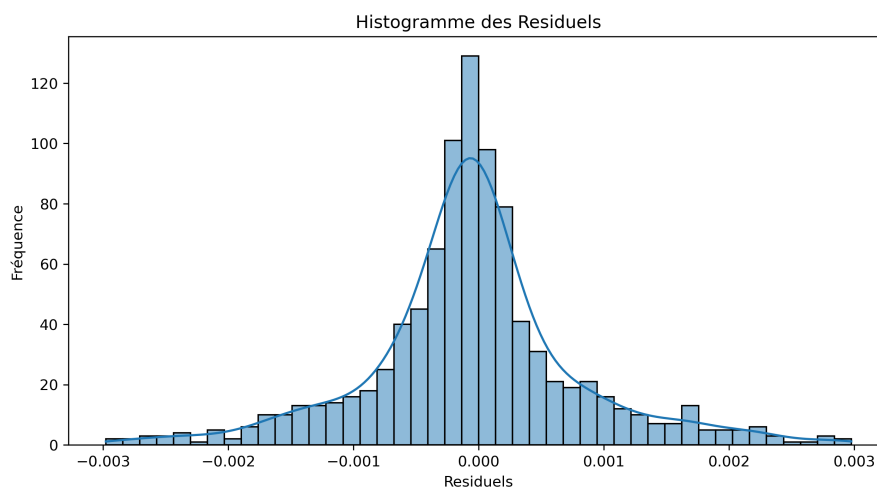
Figure 5.14 – [1 étage] Histogramme de résidus
