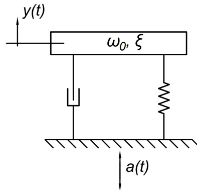
Figure 2.4 – Structure à un degré de liberté
