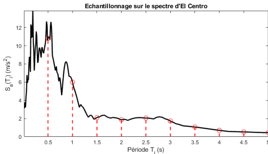
Figure 2.1 – Exemple d'échantillonnage de S_a(T_i)
