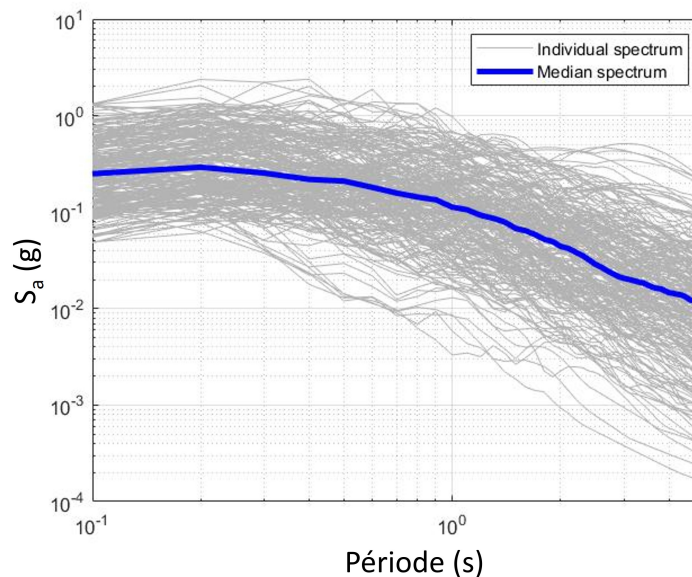
Figure 5.9 – Spectres d'accélération pour les 240 enregistrements de mouvement du sol
