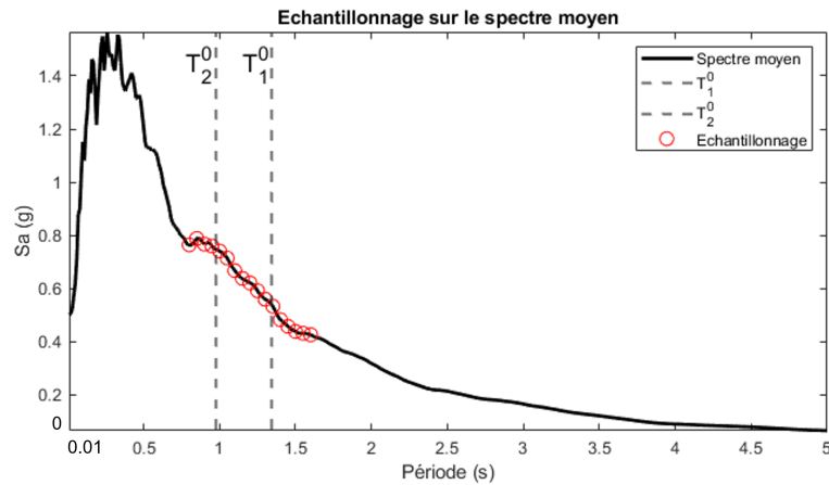
Figure 2.12 - [2ddl] Échantillonnage du spectre de réponse en accélération moyen et périodes propres du système
