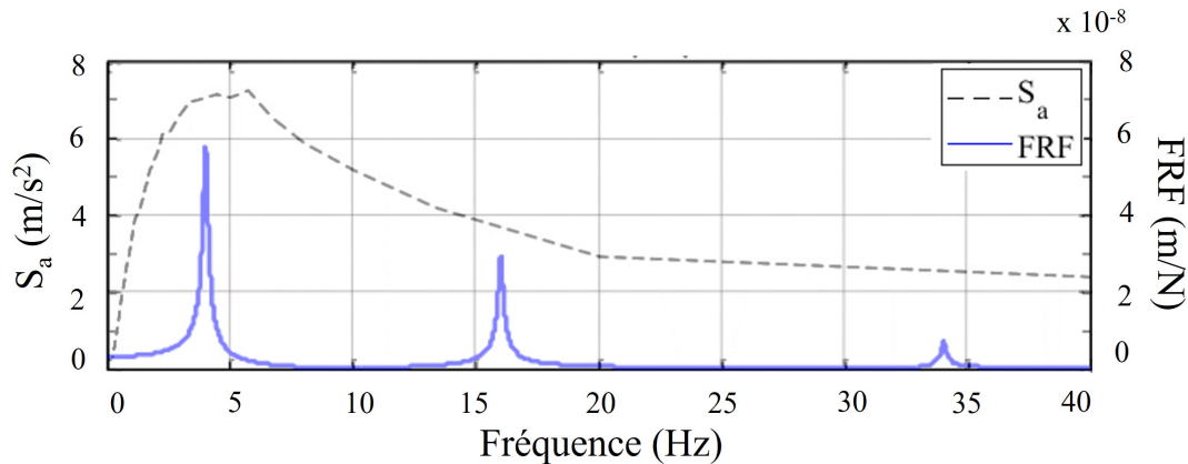
Figure 2.2 – Spectre de réponse en accélération avec la fonction de réponse en fréquence
