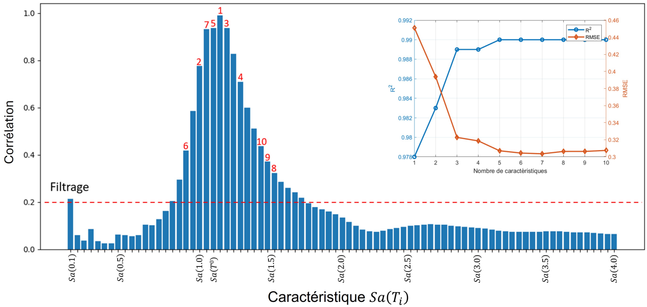
Figure 3.34 – [Bouc-Wen] Sélection pour \alpha = 0.8
