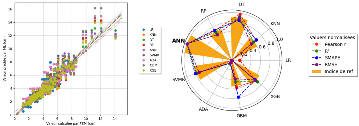
(a) Comparaison des valeurs prédites et actuelles (b) Comparaison des critères d'évaluation
