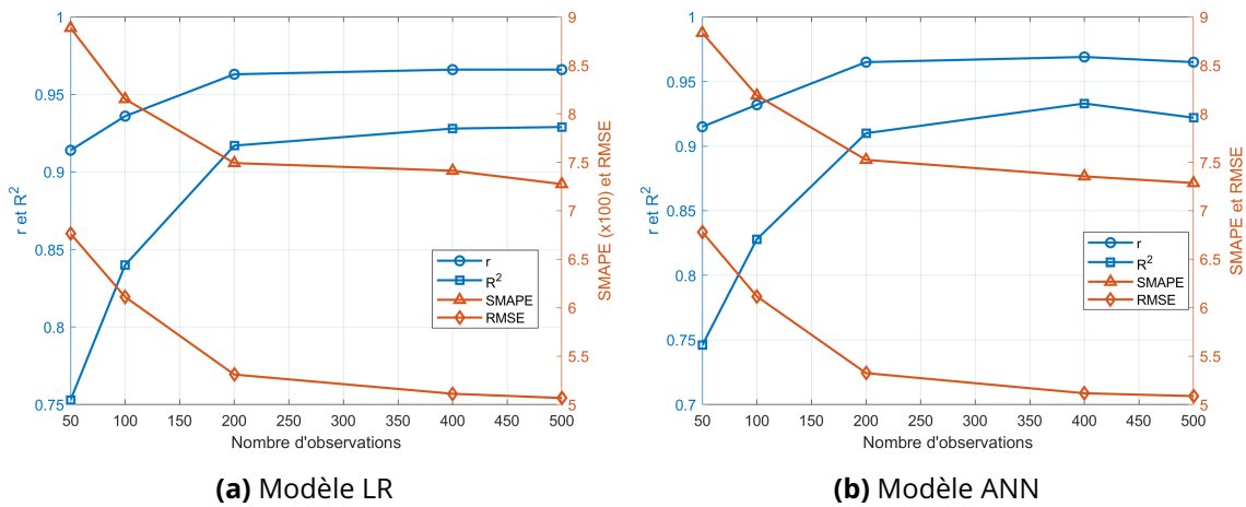
Figure 2.14 – [2ddl] Influence du nombre d'observations
