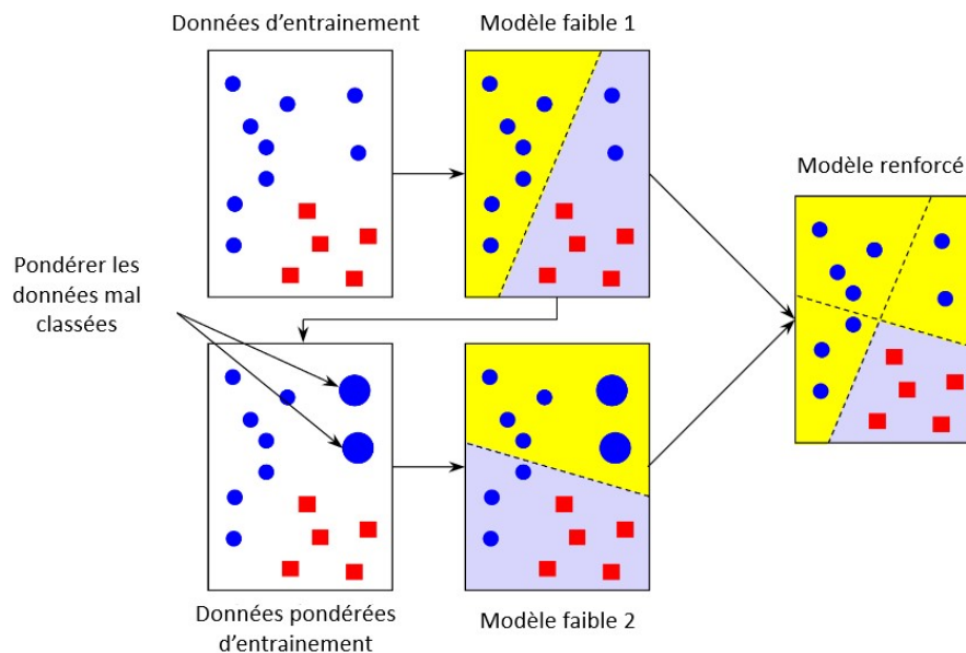
Figure 1.12 – Implémentation de AdaBoost avec deux modèles faibles
