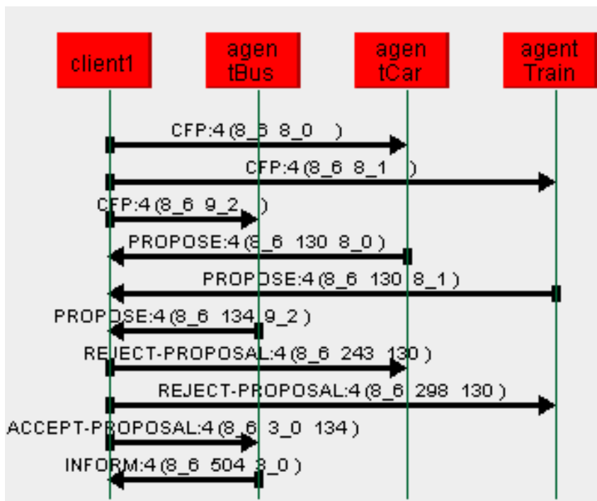
FIGURE C.2 – Vue du Sniffer de l'IHM de JADE : Echanges entre les agents.
