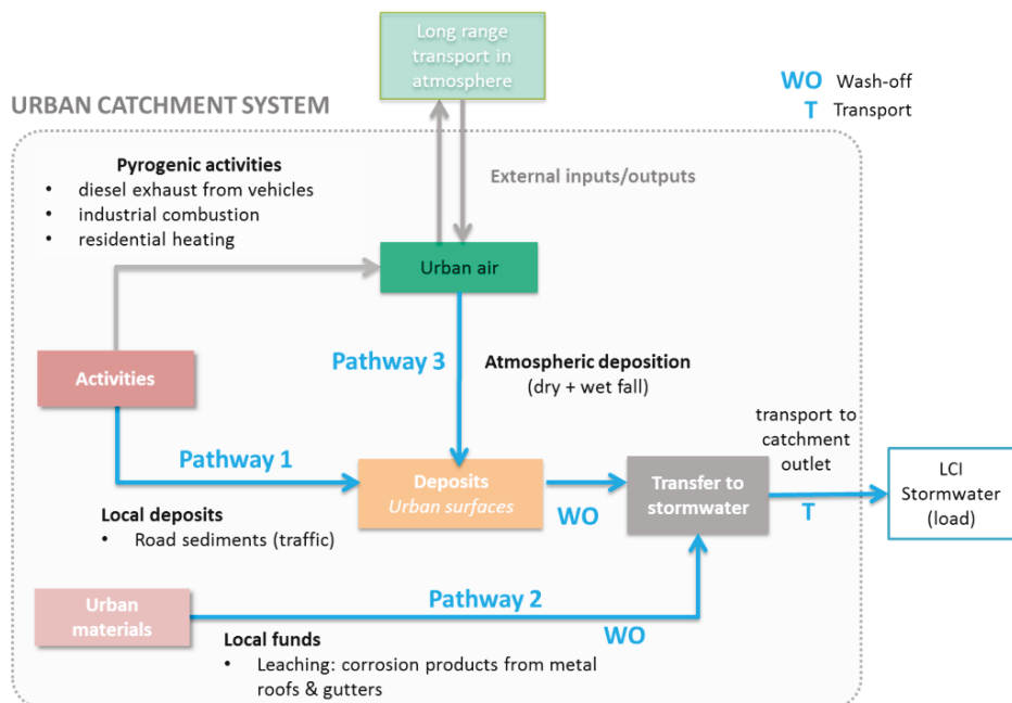
Figure 31. Modélisation des voies d'entrée pour les polluants des eaux pluviales provenant de sources diffuses urbaines (en bleu, voies considérées dans le cadre conceptuel; en gris, voies non incluses)
