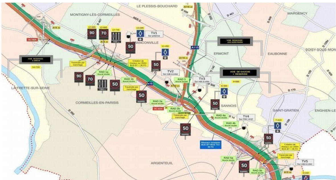
FIGURE B.3 – Synoptique simplifié lié au projet de VR2+ sur l’A15. Source : DiRIF
