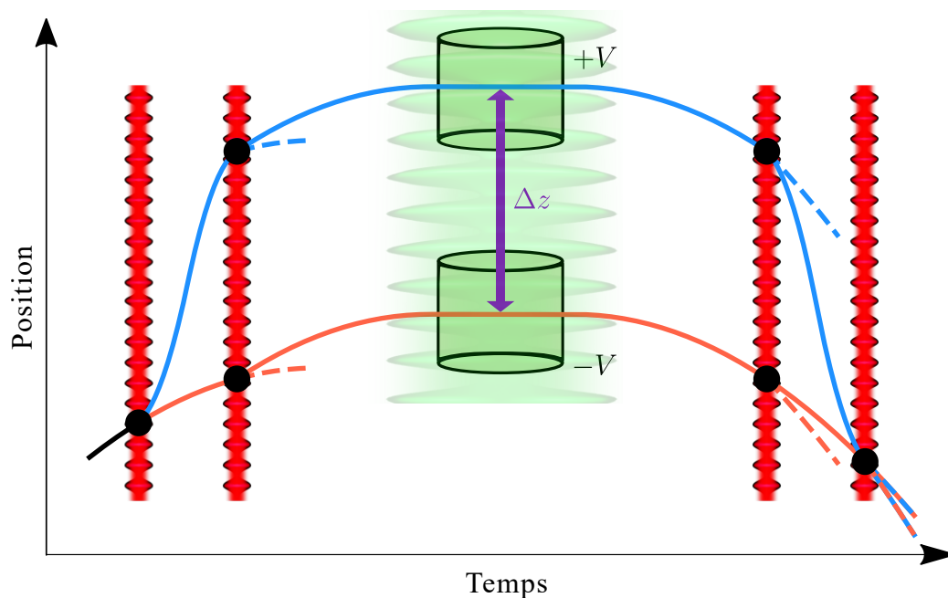
FIGURE 6.1 – Schéma spatio-temporel d'un interféromètre LMT piégé. Après un premier pulse \pi/2 , une accélération et une décelération d'un des bras est réalisé pour augmenter la séparation spatiale \Delta z . Un deuxième pulse \pi/2 ramène les deux bras dans le même état d'impulsion (au prix de pertes d'atomes dans les chemins représentés en traitillés). Ces deux paquets d'ondes sont maintenus contre la gravité par accélération continue pendant un temps suffisamment grand pour appliquer les potentiels électrostatiques. Ensuite, un troisième pulse \pi/2 est appliqué dans la direction opposée, suivi d'une nouvelle séquence d'accélération et de décelération. Enfin, un dernier pulse \pi/2 est effectué pour recombiner les chemins.
