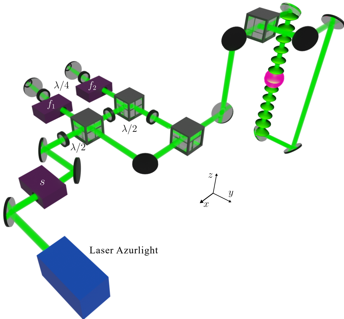
FIGURE 2.15 – Schéma du banc du réseau de lancement. La lumière issue du laser passe à travers un premier modulateur acousto-optique. Le faisceau est séparé en deux chemins passant à travers deux modulateurs en double passage. Enfin, les deux faisceaux sont emmenés en haut et en bas du dispositif principal dans le but de créer le réseau de lancement à la verticale.
