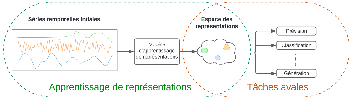
Figure F.1: Visualisation de la pipeline d'apprentissage de représentations pour les séries temporelles. Étape 1 : apprendre la représentation de la série temporelle par apprentissage non supervisé. Étape 2 : application d'un modèle supervisé par dessus la représentation apprise pour traiter une tâche en aval. Ce graphique est inspiré de Trirat et al. (2024) .
