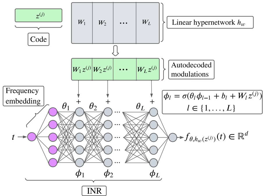
Figure F.4: Vue d'ensemble de l'architecture TimeFlow. Forward pass pour approximer la série temporelle \mathbf{x}^{(j)} au pas de temps t . \mathbf{z}^{(j)} représente la représentation apprise, \sigma la fonction d'activation ReLU, \phi les couches de l'INR et les autres symboles non définis sont des paramètres apprenables.
