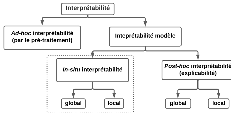
Figure F.3: Taxonomie des modèles de séries temporelles interprétables introduite dans Wang (2021).
