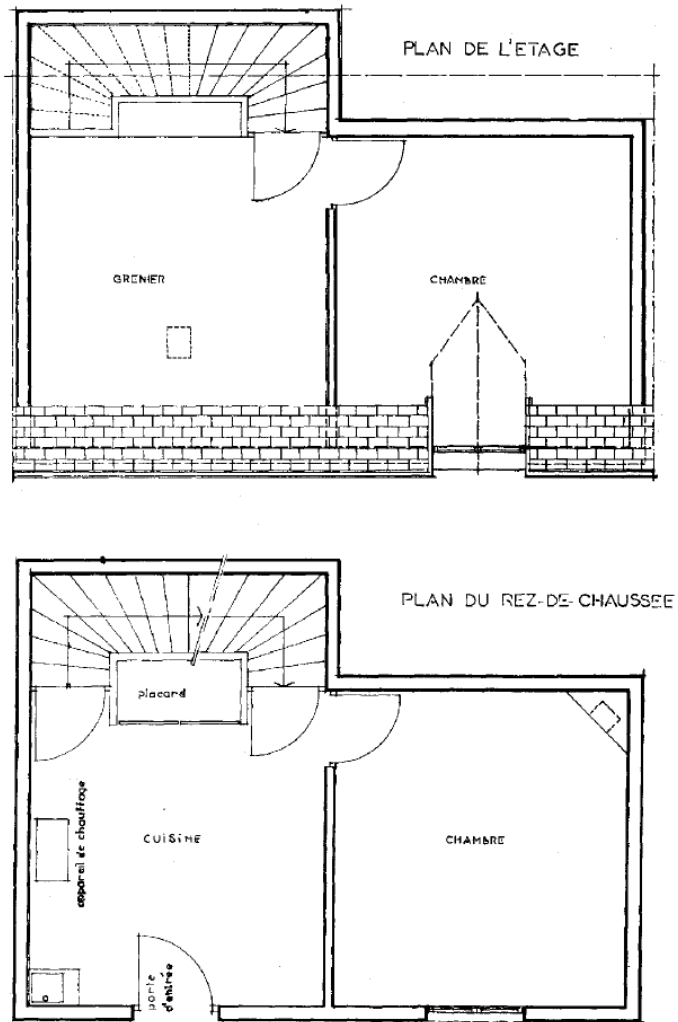
Illustration 7. Une maison des corons : plan de coupe
