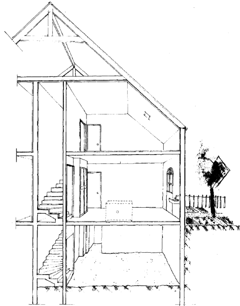
Illustration 8. Schéma d'un logement des corons
