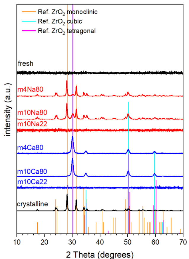
Figure 1 : Diagrammes DRX des échantillons de ZrO 2 (s): rouge: phases solides vieilles dans des solutions de NaOH; bleu: phases solides vieilles dans des solutions de CaCl 2 ; noir: phases de ZrO 2 (s) fraîchement précipitées et cristallines. Les lignes verticales indiquent les données de référence rapportées pour ZrO 2 (cr) dans la base de données COD.
