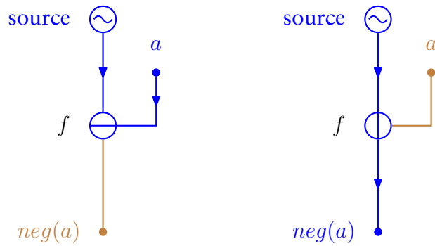
FIGURE 11.2 – La fonction neg(a) , pour e(a) = \text{vrai} , et e(a) = \text{faux}
