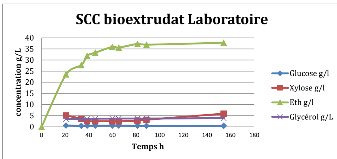
Figure 88. Concentrations de glucose, xylose, éthanol et glycérol en g/L au cours du temps de fermentation de SCC à 25% en conduite SSCF. Substrat similaire à l'expérience précédente mais fermentation en bioréacteur de 5L dans nos locaux.
