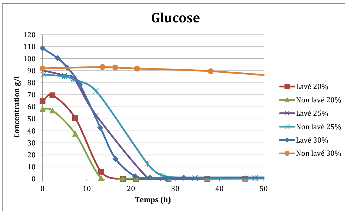
Figure 62. Consommation du glucose par CelluX 4 en SHF à partir SCC prétraité lavé ou non à différents taux de matières sèches
