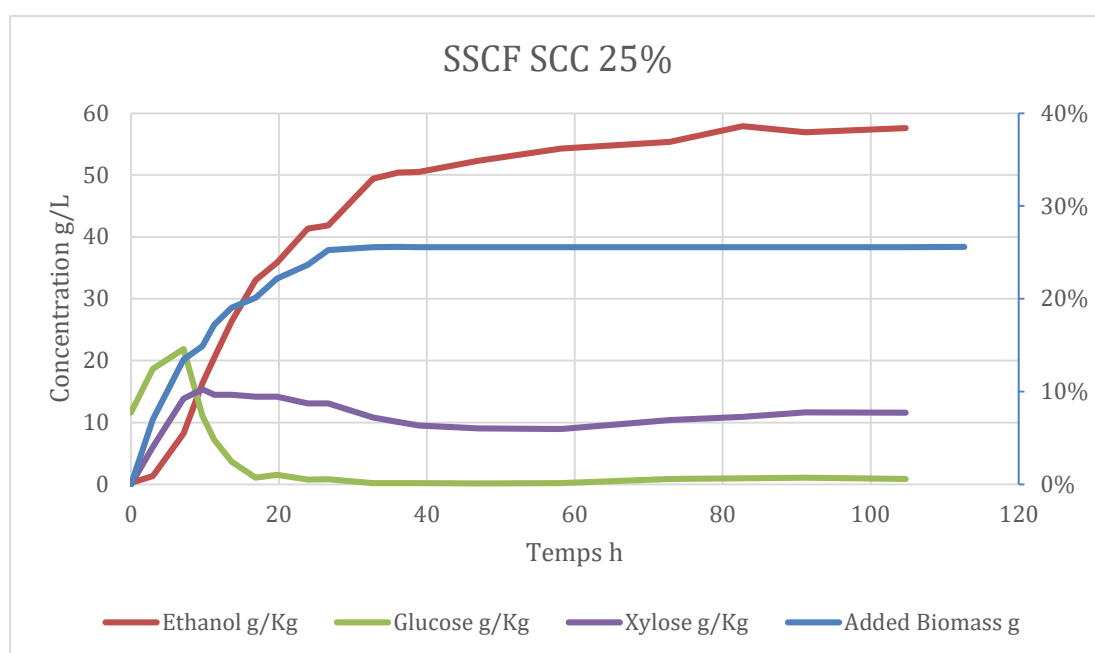
Figure 73. Concentration résiduelle de glucose, de xylose et d'éthanol au cours d'une expérience en Fed batch. La courbe bleue représente le taux de matières sèches cumulé au cours du temps
