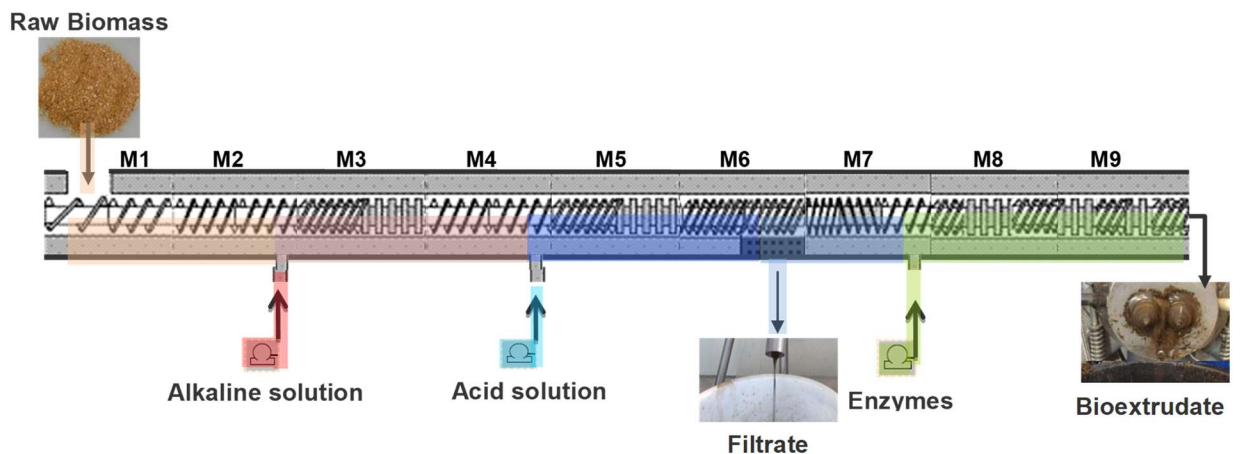
Figure 45. Schéma récapitulatif du prétraitement par extrusion bi-vis du projet BABETREAL-5
