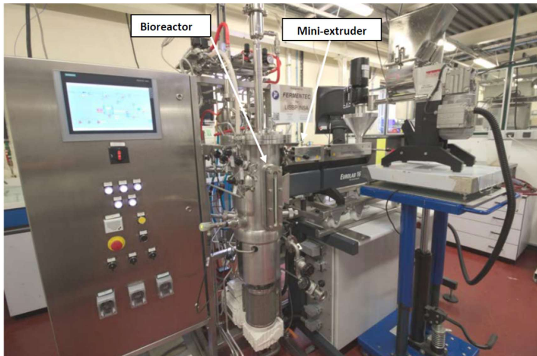
Figure 38. Photographie du matériel utilisé lors des expériences de Fedbatch
