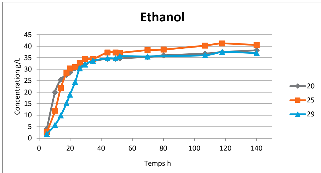
Figure 53. Concentration résiduelle d'éthanol au cours d'une expérience en SSF de SCC à différents taux de matière sèches (20%, 25%, 29%)
