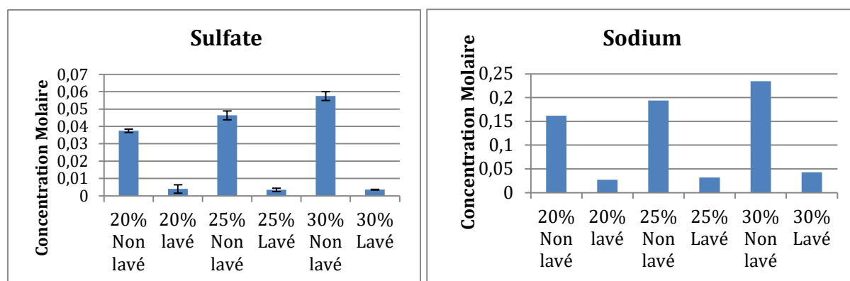
Figure 58. Comparaison des concentrations de sel de sulfate et de sodium dans les extrudats de Sweet Corn Cob prétraité et lavé ou non à différents taux de matière sèches
