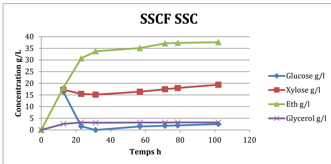
Figure 78. Concentrations du glucose, xylose et éthanol lors d'expériences de SSCF à partir de SCC à 22%
