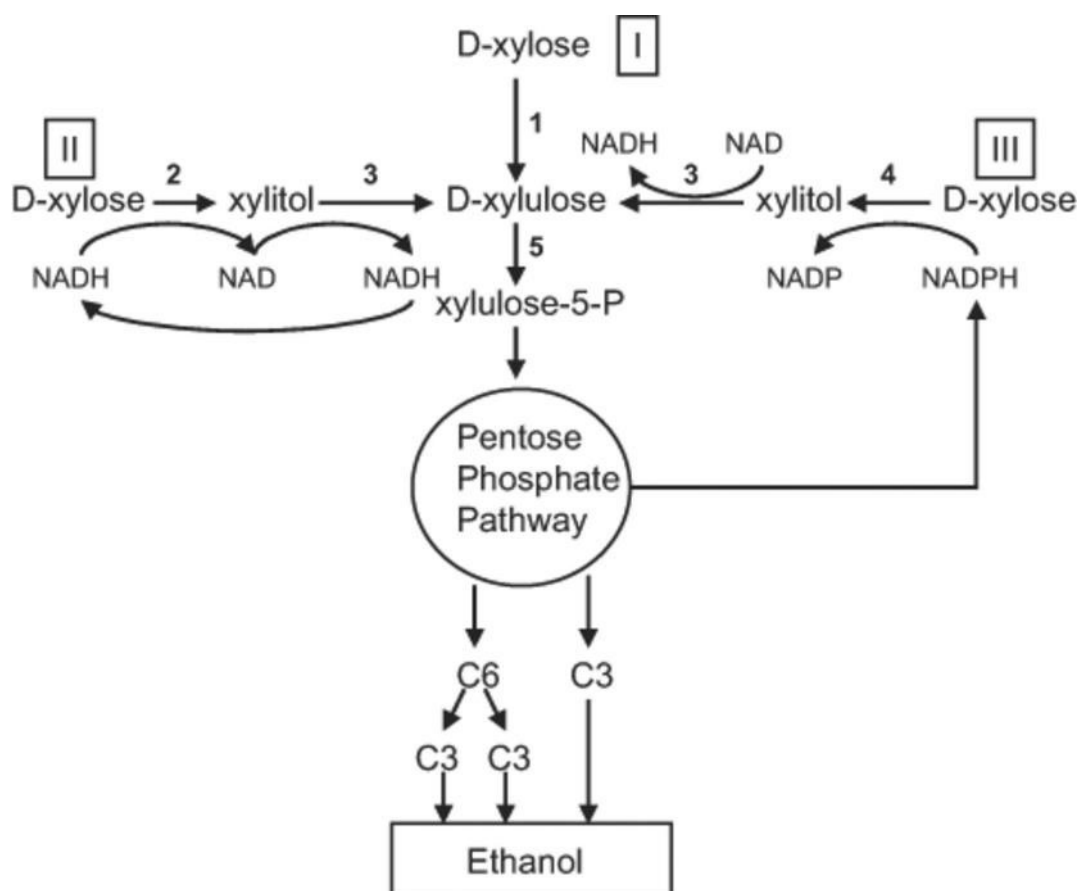
Figure 32. Conversion du xylose en éthanol via des voies métabolique dépendante(III) ou indépendante de cofacteurs (I-II) (Kuyper et al., 2003)
