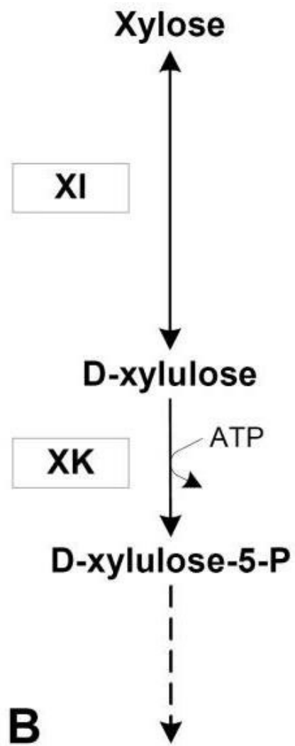
Figure 34. La voie métabolique Xylose Isomérase (XI) (Karhumaa et al., 2007)
