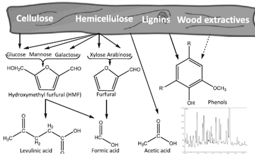
Figure 30. Formation des inhibiteurs lignocellulosiques (Jönsson et al., 2013)
