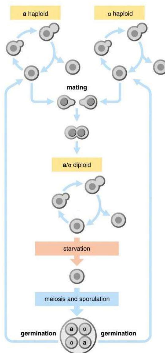
Figure 25. Cycle de vie de S. Cerevisiae (Sun & Heitman, 2011)
