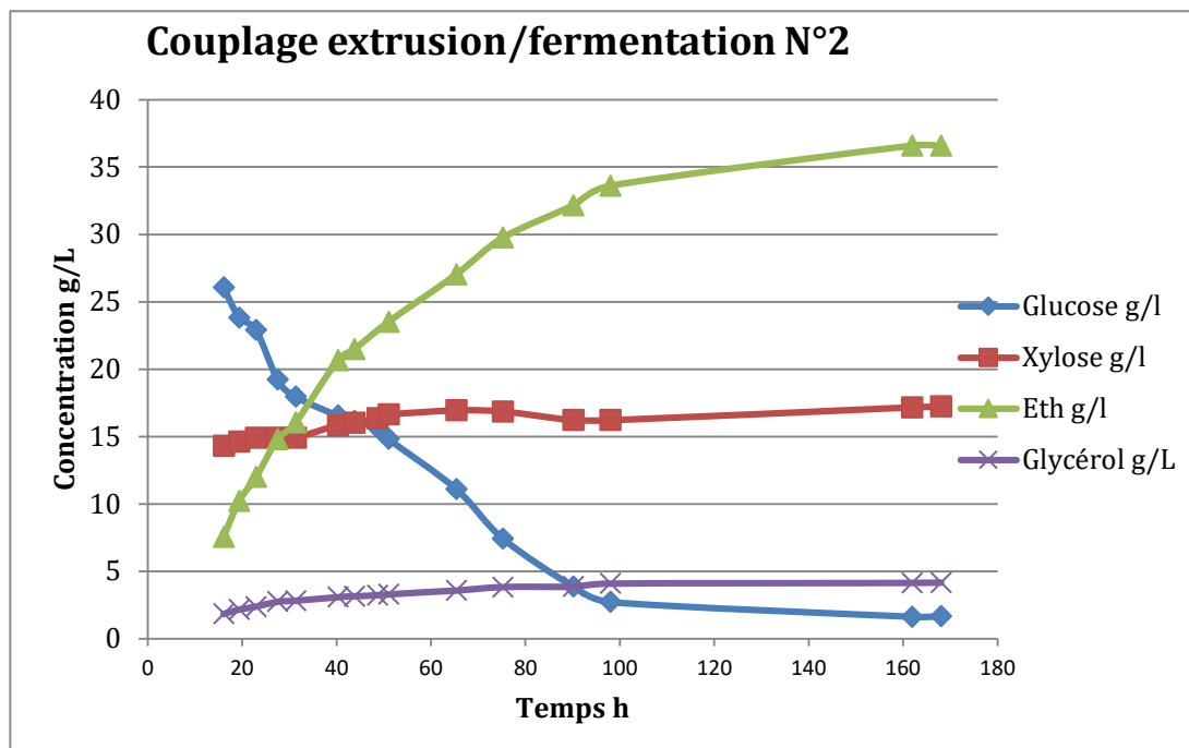
Figure 87. Concentrations de glucose, xylose, éthanol et glycérol en g/L au cours du temps de fermentation de SCC à 25% en conduite SSCF lors d'un coulage extrudeur, bioréacteur.
