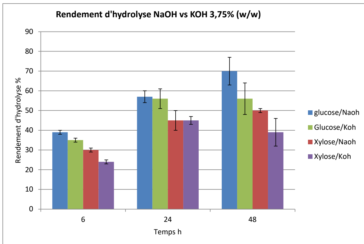
Figure 46. Performances du NaOH comparé au KOH sur le rendement d'hydrolyses du glucose et du xylose. Pré-traitement à 150°C, solution alcaline à 3.75% (w/w). Données produite par INPT et UNAM
