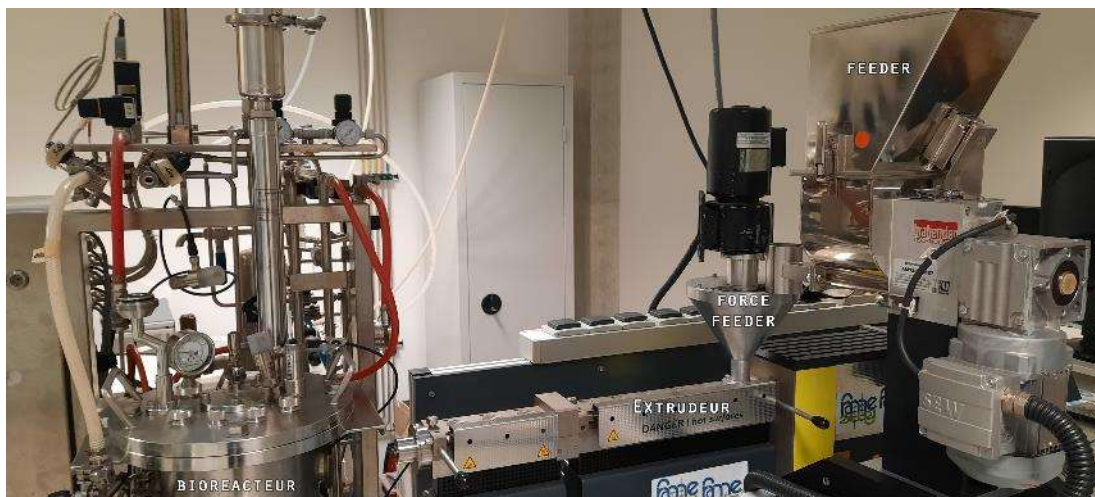
Figure 69. Plan rapproché de l'équipement utilisé pour les expériences en Fed Batch. Un feeder posé sur une balance est utilisé pour mesurer les quantités d'extrudat qui sont envoyées dans l'extrudeur. Ce substrat passe ensuite dans un force feeder à vis qui permet de remplir efficacement l'extrudeur bi-vis pour avoir un apport de matière continu.
