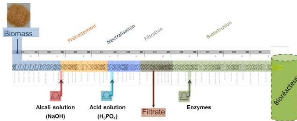
Figure 84. Schéma récapitulatif du couplage extrusion/fermentation
