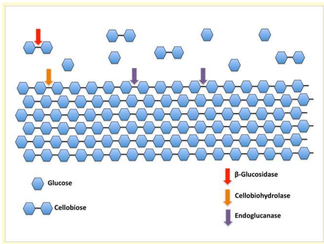
Figure 19. Vue schématique de la dégradation de la cellulose. Les endoglucanases hydrolysent les liaisons de la cellulose en interne, les cellobiohydrolases clivent les unités de cellobiose à l'extrémité des chaînes polysaccharidiques. Finalement les unités de cellobiose libérées sont hydrolysées par les \beta -Glucosidases en glucose.
