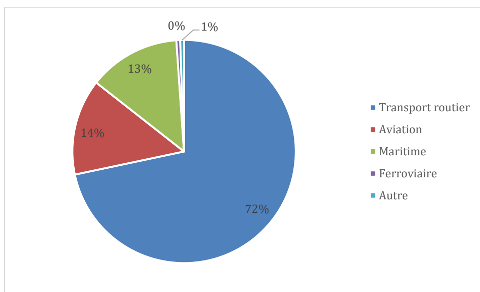
Figure 2. Parts des émissions de gaz à effet de serres par secteur en Europe en 2017. ( https://www.eea.europa.eu/data-and-maps/indicators/transport-emissions-of-greenhouse-gases/transport-emissions-of-greenhouse-gases-12 )
