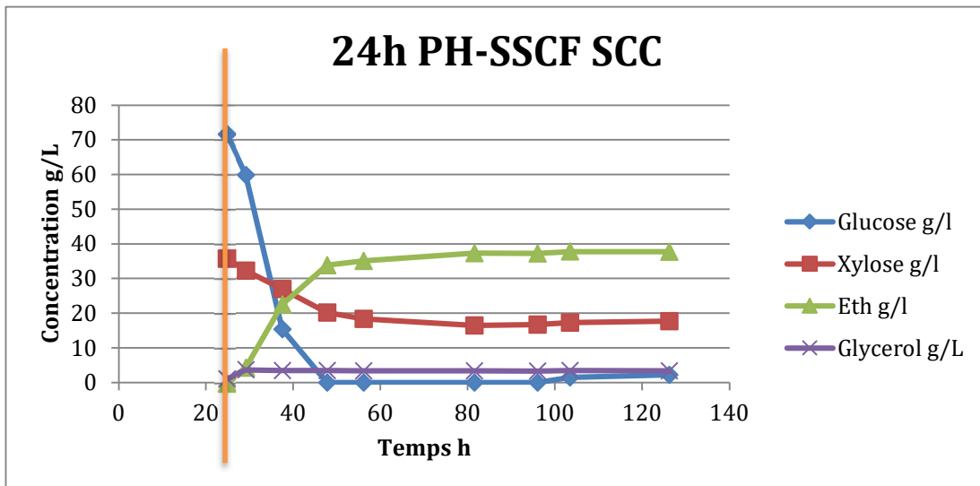
Figure 79. Concentrations du glucose, xylose et éthanol lors d'expériences en Pré-hydrolyse de 24h suivi de la fermentation (SSCF) à partir de SCC à 22%. Le trait orange représente la fin de la pré-hydrolyse et le début de la fermentation
