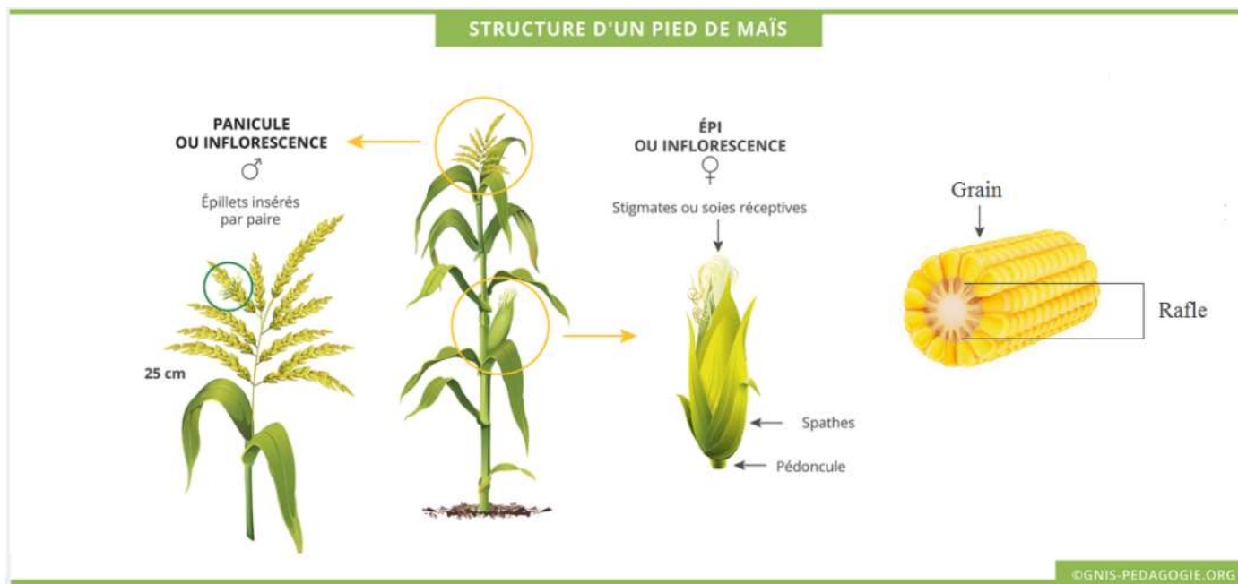
Figure 44. Structure d'un plant de maïs
