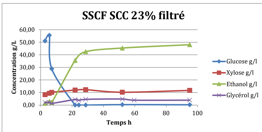
Figure 51. Résultats de SSCF avec du bioextrudat SCC prétraité avec filtration, 23% de matières sèche.
