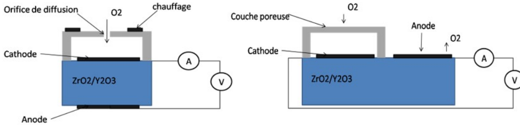
FIGURE 1.12 – Structure d'un capteur d'oxygène ampérométrique avec un orifice de diffusion [40].
