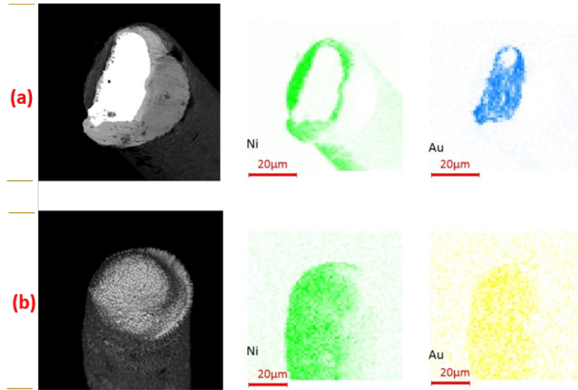
FIGURE 3.10 – Images MEB et EDX pour la surface du fils (a) après recuit à 350°C pendant 500h (b) après recuit à 650°C pendant 500h.
