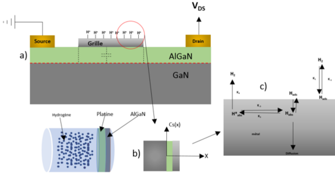
FIGURE 5.19 – Schéma capteur de gaz à grille flottante à base de HEMT AlGaN / GaN. Les gaz cibles sont adsorbés sur la grille et sont couplés capacitivement au canal situé en dessous.
