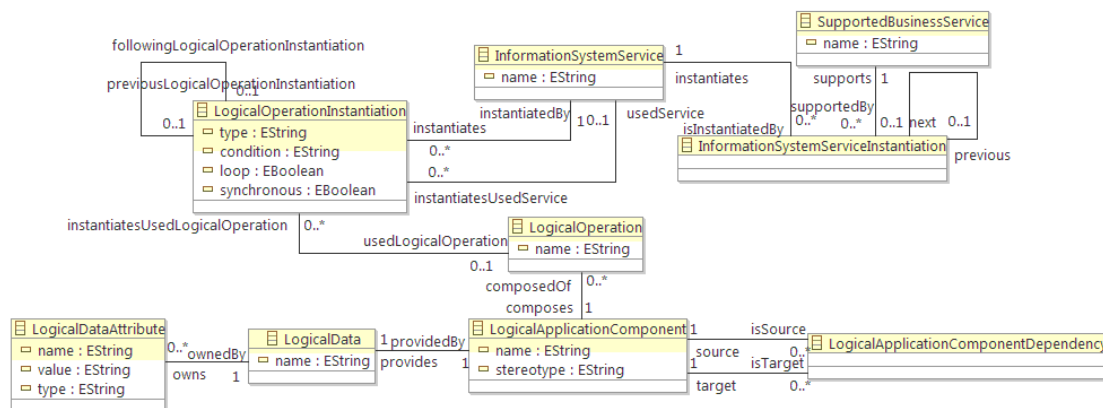
FIGURE 3.8 – PIM : Modèle des composants d'application logiques du SI associé à TCM-LIS (cf. [157])
