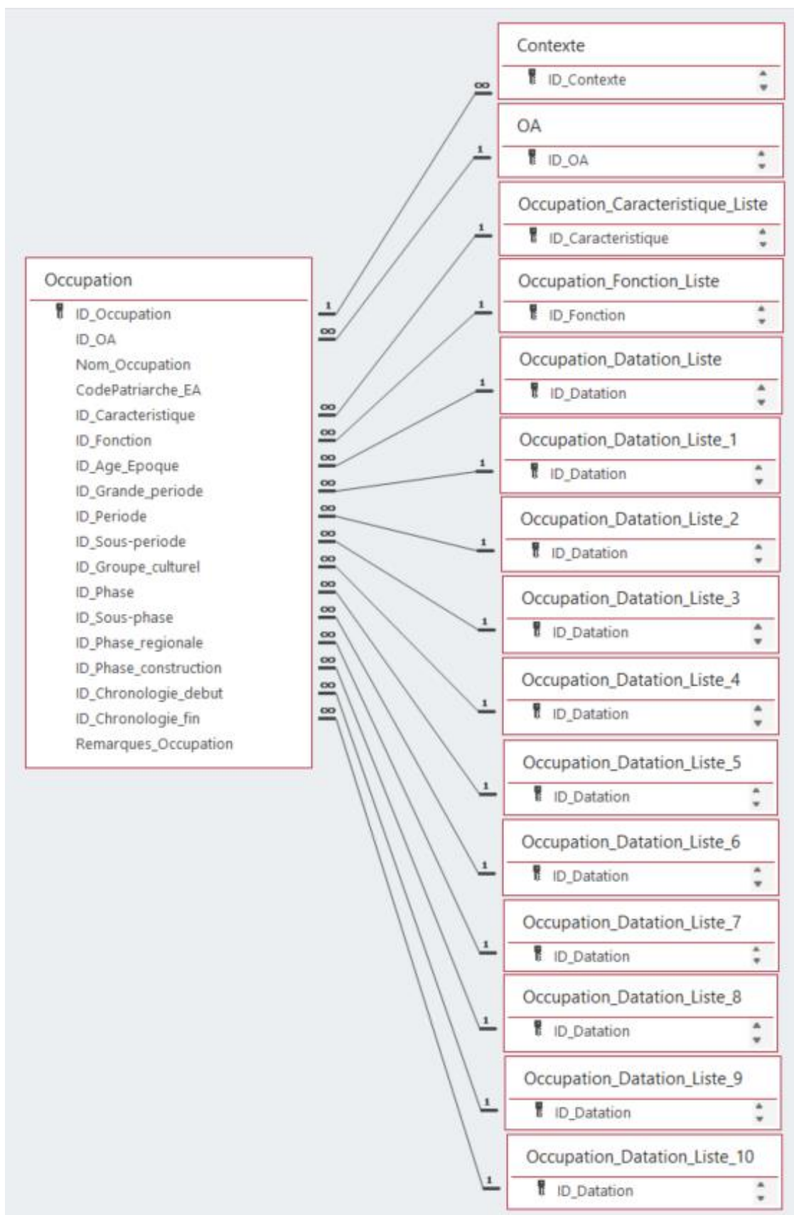
Fig. 3 - Schéma relationnel simplifié de la table « Contexte ». Seules les relations directes sont affichées.
