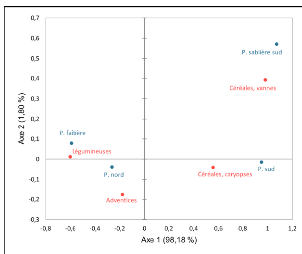
Fig. 136 - Graphique symétrique de l'AFC réalisée sur les données de la maison M2 de Marainville-sur-Madon « sous le Chemin de Naviot ». Axes 1 et 2 (99,99 % de la variance). Rouge : catégories de plantes (colonnes) ; Bleu : ensembles archéologiques (pannes, lignes) ; P : panne ; Valeurs : NMI.
