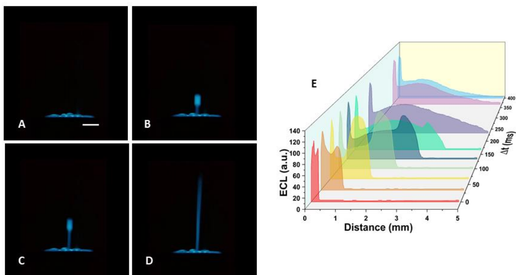
Figure 5. Images ECL ( A-D ) montrant la trajectoire d'une bulle de \text{Cl}_2 générée par électrochimie à différents moments (0 ms, 67 ms, 100 ms et 367 ms, respectivement) après son détachement de la surface de l'électrode de carbone vitreux pendant un balayage en voltampérométrie cyclique de 0 V à 3 V à une vitesse de balayage de 0,1 \text{ V s}^{-1} . Barre d'échelle 1 mm. ( E ) Extension spatiale de l'émission ECL suite au détachement d'une bulle de \text{Cl}_2 de la surface de l'électrode (les images correspondantes sont montrées dans ( A-D )). La propagation de l'ECL jusqu'à 5 mm de l'électrode indique la possibilité d'une formation retardée des espèces radicalaires réactives lors de la dissolution du gaz emprisonné dans la bulle.
