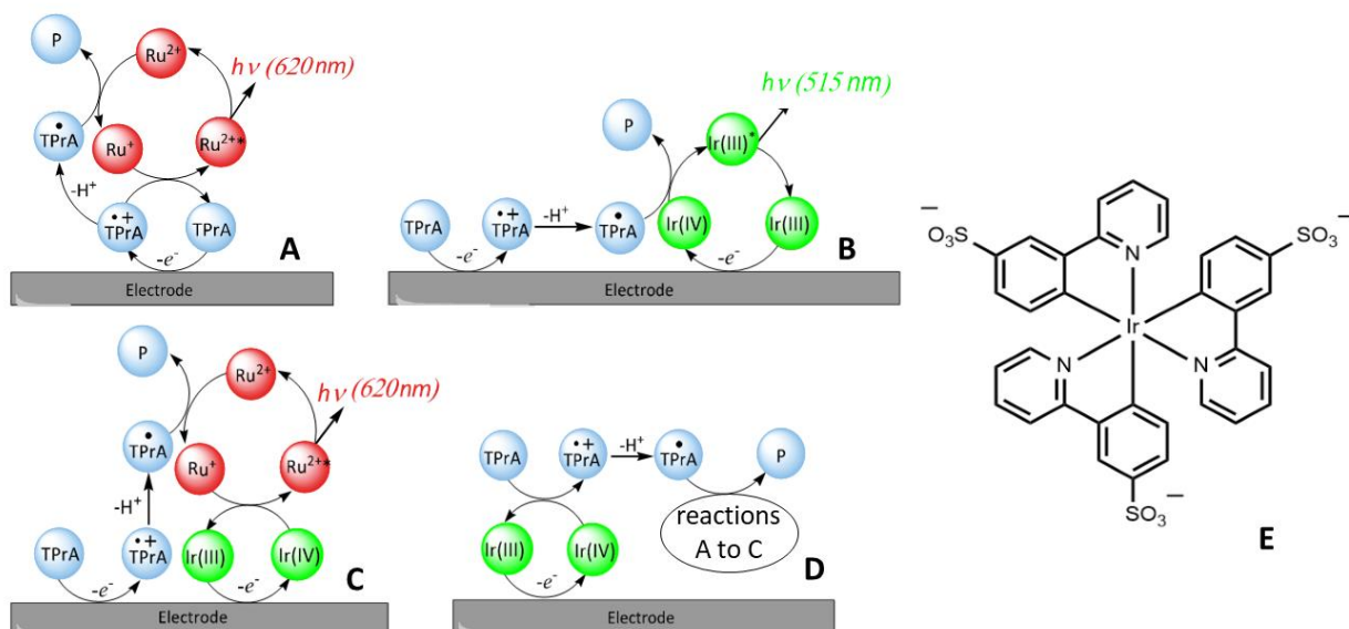
Figure 1. Schémas de la (A) voie ECL conventionnelle "à distance", (B) voie directe vers l'ECL [\text{Ir}^{\text{III}}(\text{sppy})_3]^{3-} , (C) voie ECL améliorée "à médiation redox" et (D) catalyse redox (oxydation catalytique de TPrA par [\text{Ir}^{\text{IV}}(\text{sppy})_3]^{2-} ). \text{Ru}^{2+} , \text{Ir}(\text{III}) et TPrA représentent respectivement le luminophore [\text{Ru}(\text{bpy})_3]^{2+} , le médiateur redox [\text{Ir}^{\text{III}}(\text{sppy})_3]^{3-} et la tri- n -propylamine. (E) Structure chimique du complexe [\text{Ir}(\text{sppy})_3]^{3-} .
