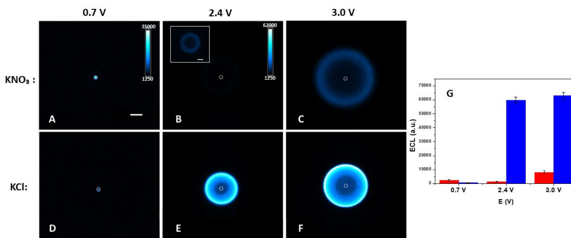
Figure 4. (A-F) et (H-K) Images de l'émission ECL au niveau de la microélectrode d'or dans la solution PBS 0,2 M (pH 8) contenant 0,5 M \text{H}_2\text{O}_2 , 0,42 mM L-012 et 50 mM (A-C) \text{KNO}_3 ou (D-F et H-K) \text{KCl} . Le potentiel de l'électrode a été réglé à (A et D) 0,7 V, (B et E) 2,4 V et (C et F) 3 V vs Ag/AgCl pendant 20 s. Les images ECL en fausses couleurs (A et D) et (B, C, E et F) ont été codées avec les échelles d'intensité lumineuse 1200-35000 (montrées en A) et 1200-62000 (montrées en B), respectivement. L'image en médaillon dans (B) a été codée avec la gamme d'intensité 1200-10000. Le cercle en pointillé matérialise le disque d'or de la microélectrode. Barre d'échelle : 50 \mu\text{m} . (G) L'intensité moyenne de l'ECL en présence de l'électrolyte support \text{KNO}_3 50 mM (en rouge) ou \text{KCl} 50 mM (en bleu) lors de l'application d'impulsions chronoampérométriques de 0,7 V, 2,4 V et 3 V par rapport à Ag/AgCl. Les valeurs de l'histogramme représentent la moyenne des expériences pour chaque condition, comme le montrent les images (A-F), réalisées en trois exemplaires en présence (en bleu) et en l'absence de \text{Cl}^- (en rouge). Les barres d'erreur indiquent \pm 1 écart-type par rapport à la moyenne.
