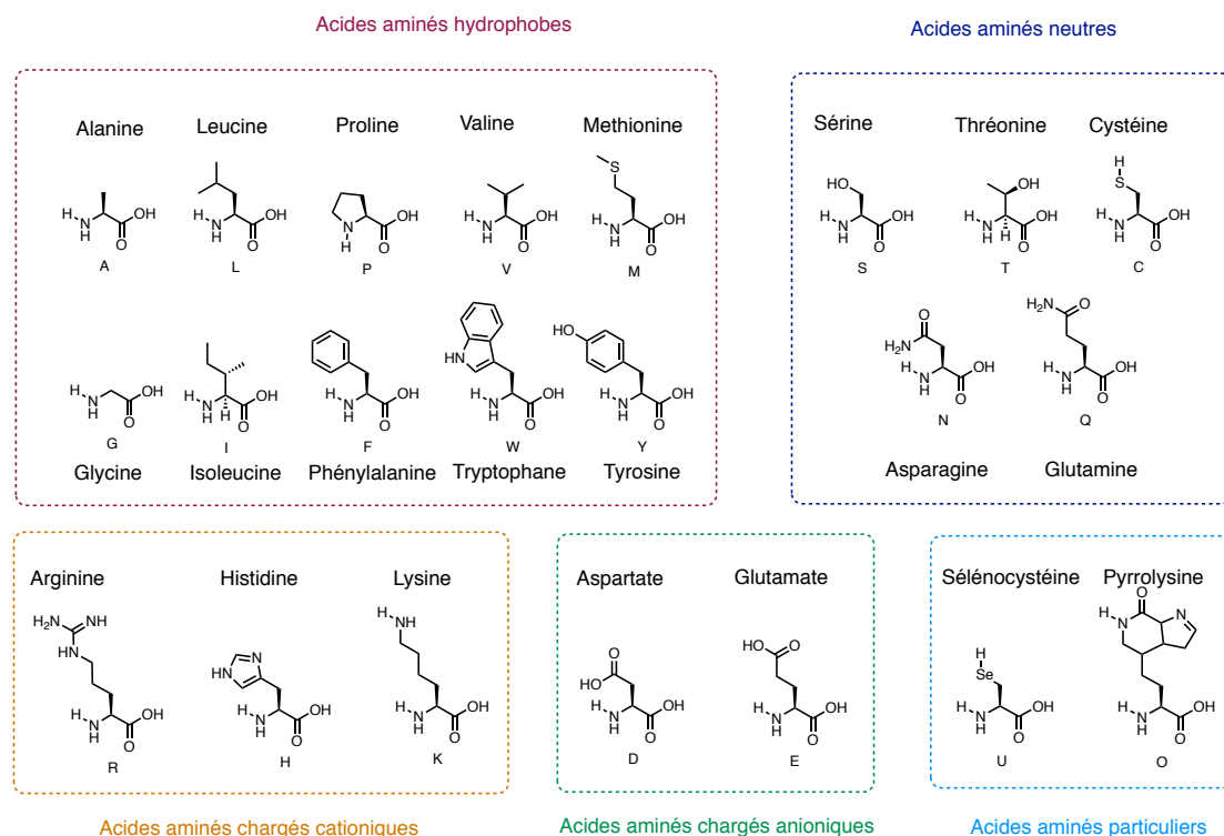
Figure 1 : Structures des acides aminés protéinogènes.
