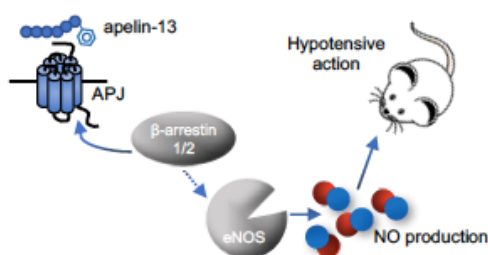
Figure 33 : Mécanisme de l'effet hypotenseur de l'apeline-13 136 .
