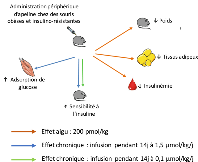
Figure 31 : Implication de l'apeline dans le diabète et l'obésité 126 .
