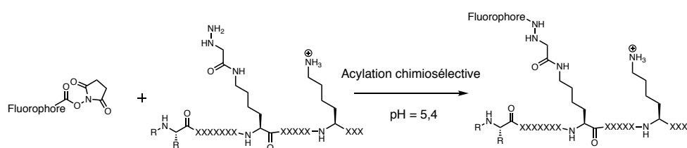
Schéma 4 : Principe de l'acylation chimiosélective pour la synthèse de peptides fluorescents.
