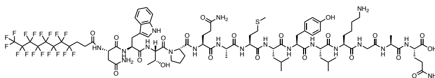
Figure 63 : Structure de la F8-spexine.
