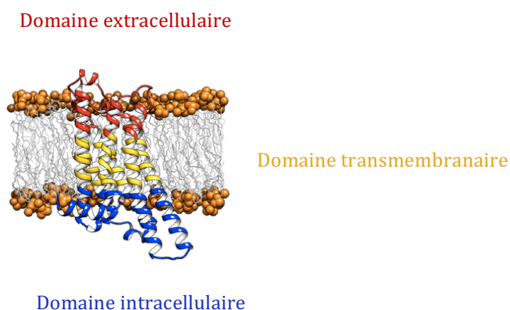
Figure 24 : Structure générale des RCPG de classe A 91 .
