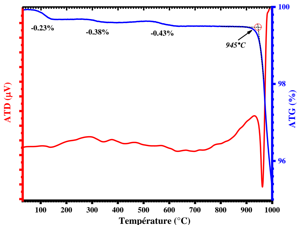
Figure IV. 2 : Analyses ATD/ATG du mélange de précurseurs ( \text{Bi}_2\text{O}_3 + \text{BiOCl} ) non-calciné.
