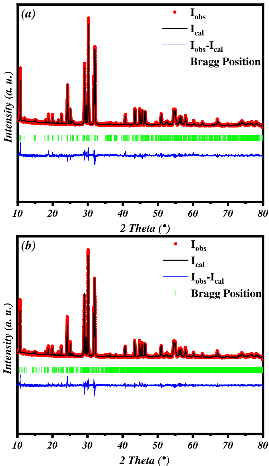
Figure IV. 6 : Profils de diffraction observés et calculés, à partir d'affinements Rietveld DRX de (a) Bi_{24}O_{31}Cl_{10} ( A2/m ) et (b) Bi_{24}O_{31}Cl_{10} ( P2/c ).
