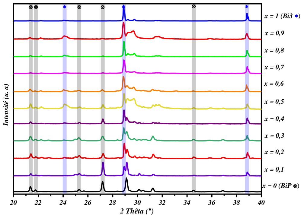
Figure V. 3 : Zoom du diffractogramme DRX des phases mixtes x\text{Bi}_3\text{O}_4\text{Cl}/(1-x)\text{BiPO}_4 dans le domaine angulaire 20 – 40°.
