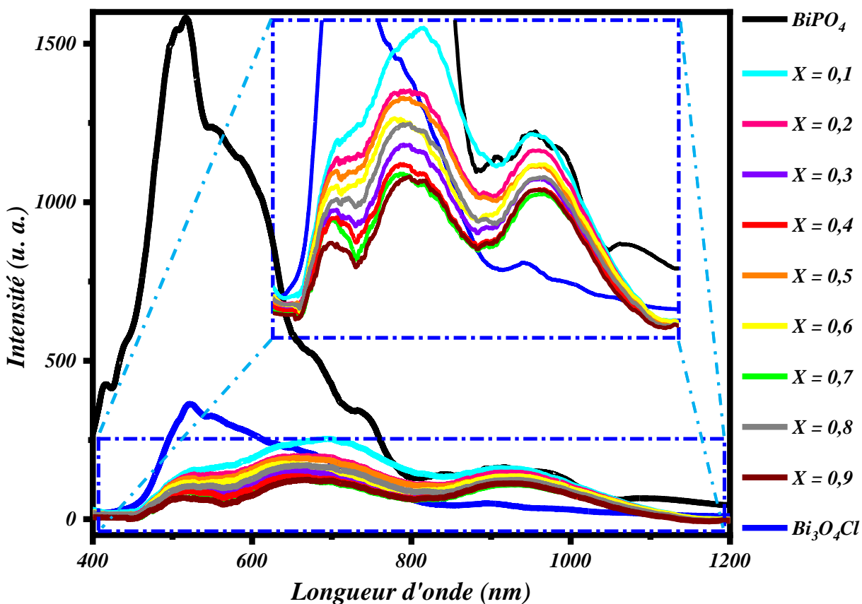
Figure V. 22 : Spectres de photoluminescence avec zoom des systèmes mixtes x\text{Bi}_3\text{O}_4\text{Cl}/(1-x)\text{BiPO}_4 ( \lambda_{exc} = 364 \text{ nm} ).
