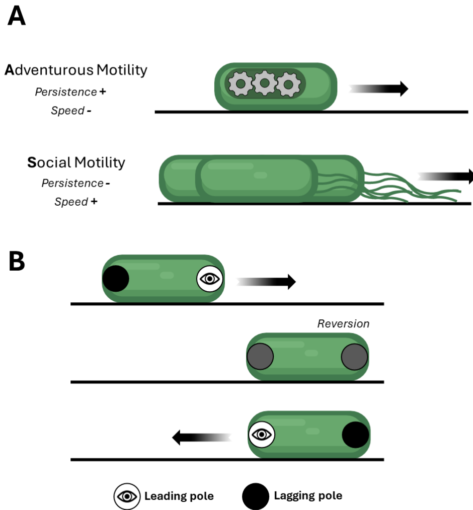
FIGURE III.1 – Schéma de la motilité de la bactérie Myxococcus xanthus . A. La bactérie M. xanthus possède deux systèmes de motilité bien distincts, la motilité aventureuse (A) et la motilité sociale (S). La motilité aventureuse se caractérise par l'activation de moteurs cellulaires latéraux, permettant à des bactéries isolées, généralement situées en périphérie de la colonie, de se déplacer de manière autonome [121]. En revanche, la motilité sociale de Myxococcus xanthus repose sur l'utilisation de pili situés aux pôles des cellules, fonctionnant comme des grappins pour favoriser un déplacement coordonné parmi les groupes de bactéries [120]. Ces deux motilités ont des propriétés de déplacement différentes concernant les caractéristiques de vitesse ou de temps de persistance le long d'une trajectoire. B. Illustration du phénomène de « réversion ». La bactérie possède deux pôles, l'un correspondant à la tête (Leading pole) et l'autre à la queue (Lagging pole). Ces deux pôles peuvent s'inverser, la tête devenant queue et inversement.
