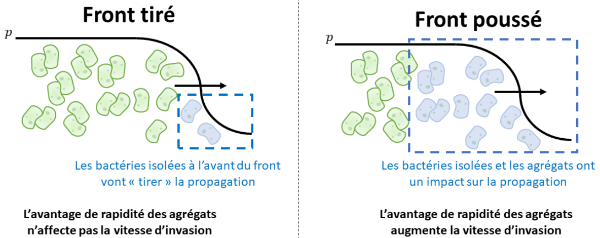
FIGURE III.4 – Illustration du régime de front tiré et de front poussé pour l'invasion de M. xanthus . Quand le front est tiré, seules les bactéries isolées en amont du front vont contribuer à la propagation de la bactérie prédatrice [62]. Ainsi l'avantage de vitesse que possèdent les agrégats n'aura aucun effet sur la vitesse d'invasion. A l'inverse, dans le régime de front poussé, les agrégats ont cette fois-ci également un rôle, ils « poussent » le front. Dans ce cas de figure, l'avantage de vitesse des agrégats permet une invasion plus rapide.
