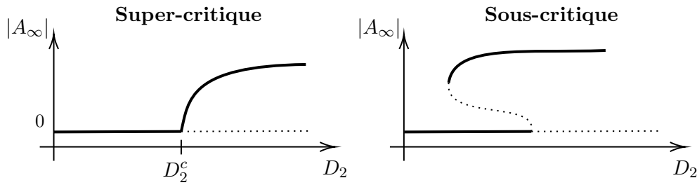
FIGURE I.4 – Illustration de bifurcation de Turing super-critique et sous-critique. Les lignes pleines sont stables tandis que les lignes pointillées sont instables.
