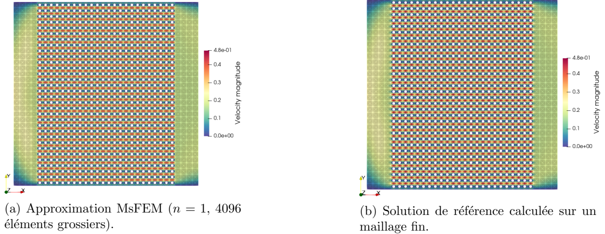
Figure 2.12: Simulation bi-dimensionnelle d'un écoulement de Stokes dans un canal ouvert, \nu = 1 , écoulement de la gauche vers la droite avec une entrée parabolique, une sortie libre, et une vitesse nulle sur les bords haut, bas et sur les obstacles.
