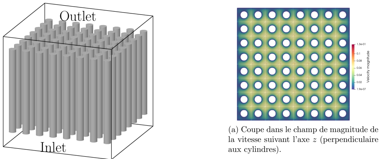
Figure 2.14: Approximation MsFEM d'un écoulement de Stokes dans un canal ouvert tridimensionnel avec une entrée parabolique, une sortie libre et une vitesse nulle sur les autres bords ( n = 2 , 3072 éléments grossiers).
