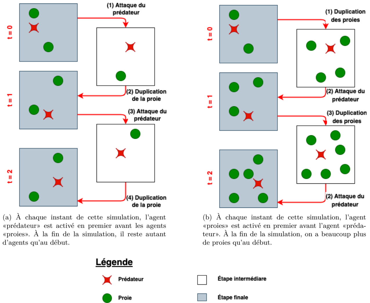
FIGURE 1.14 – Exemple d'issues possibles d'une simulation selon l'ordre d'activation des agents
