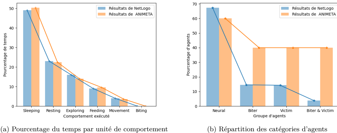
FIGURE 5.17 – Comparaison des résultats de ANIMETA avec ceux de NetLogo
