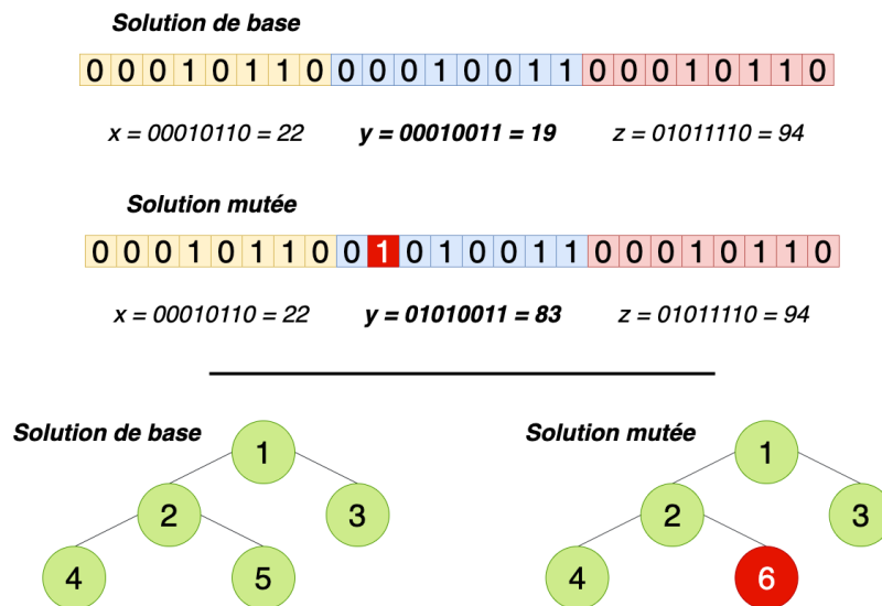
FIGURE 2.13 – Mutations avec les deux représentations de solution (binaire et arbres)
