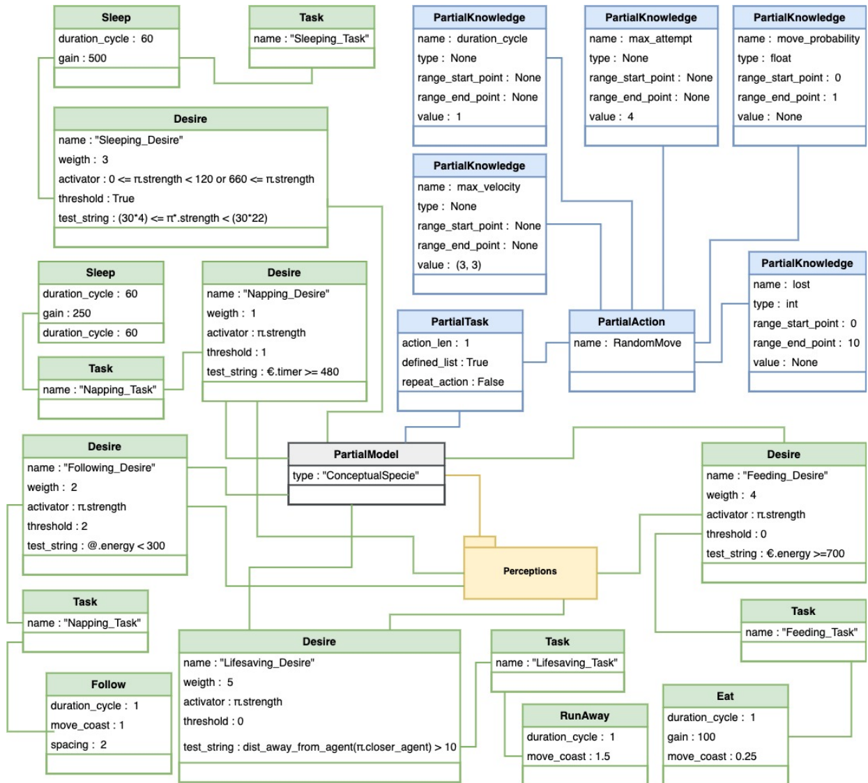
FIGURE 5.27 – Diagramme d'objet du modèle partiel (scénario 1)
