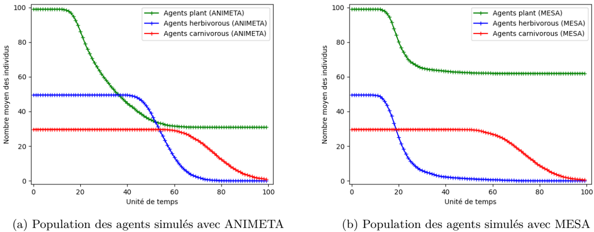
FIGURE 5.13 – Évolution de la population des agents simulés avec ANIMETA et MESA
