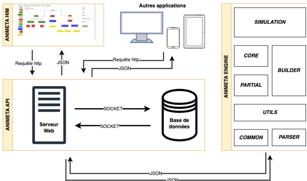
FIGURE 5.3 – Liens et échanges entre ANIMETA-HIM, ANIMETA-API et ANIMETA-ENGINE
