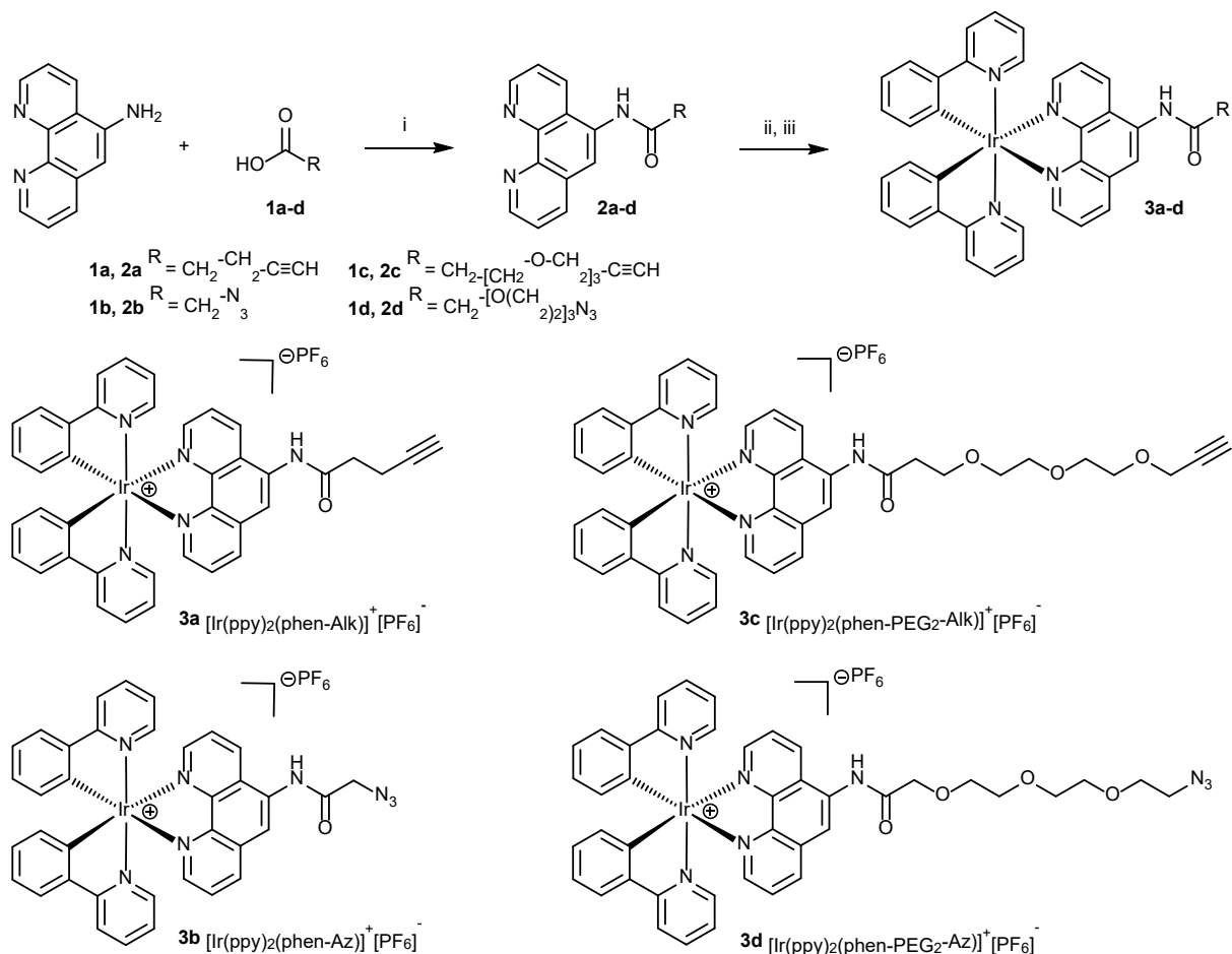
Figure 17 Synthèse et structure des sondes iridium clickables. (i) 1,10-phenanthroline-5-amine, DCC, MeCN, t.a. , 20h – 2a: 95%, 2b: 78%, 2c: 74%, 2d: 72% ; (ii) [\text{IrCl}(\text{ppy})_2] \text{CH}_2\text{Cl}_2\text{-MeOH} , 45 à 55°C, 5 à 15h ; (iii) \text{NH}_4\text{PF}_6 , t.a. , 15mn – 3a: 93%, 3b: 54%, 3c: 88%, 3d: 99%.
