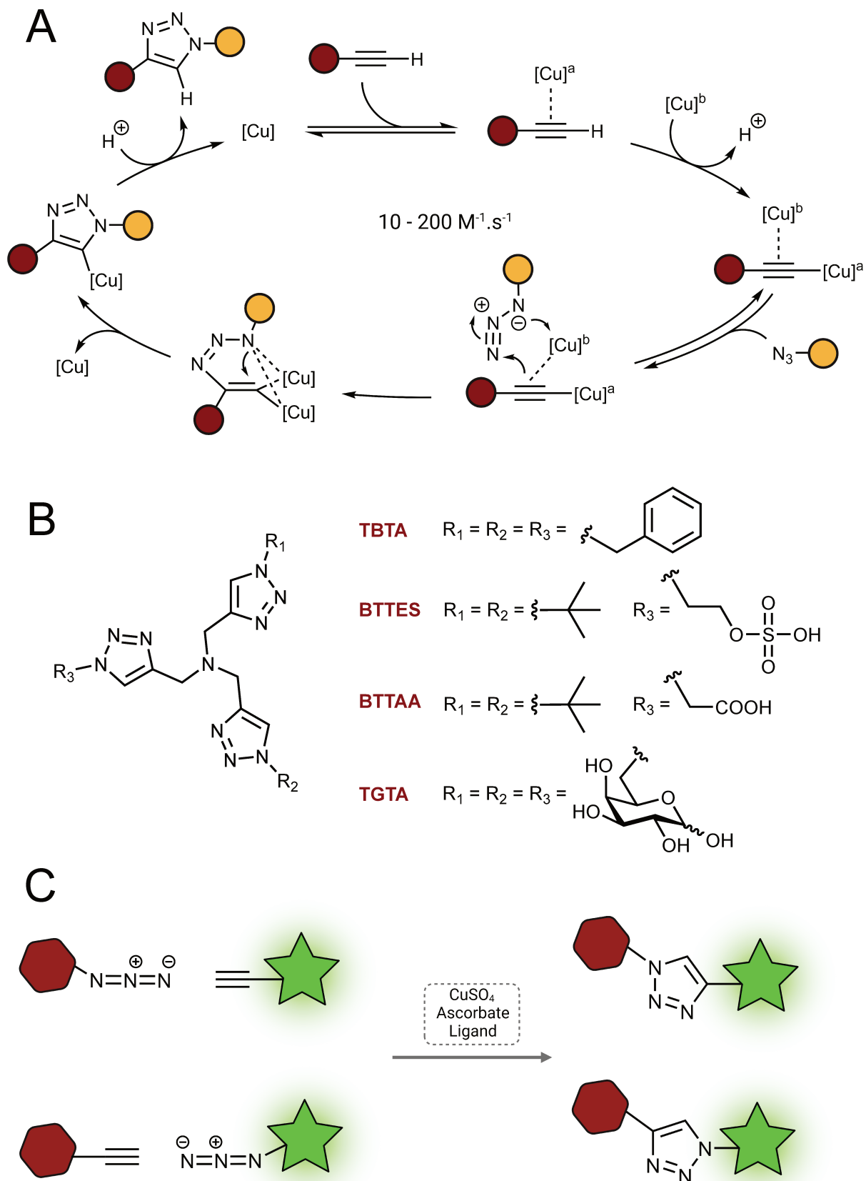
Figure 5 Copper Catalysed Azide Alkyne Cycloaddition (CuAAC). (A) Mécanisme réactionnel. (B) Ligands chélateurs couramment utilisés pour effectuer la réaction. (C) Les groupes azotures et alcynes, de par leur nature discrète et relativement inerte en milieu biologique, peuvent être utilisés aussi bien sur la sonde que sur le rapporteur, de façon interchangeable.
