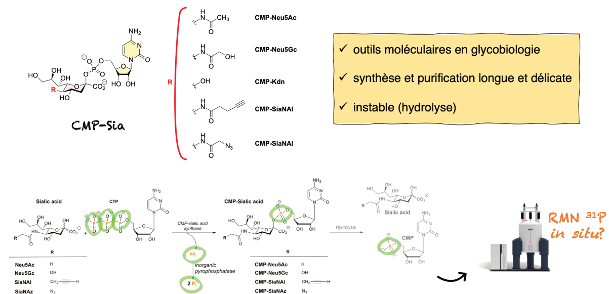
Figure 20 Rapporteurs chimiques de type CMP-acides sialiques utilisés pour l'étude de la biosynthèse des chaînes poly acides sialiques. Ces rapporteurs chimiques ont été synthétisés via une réaction enzymatique in vitro . La RMN du phosphore ^{31}\text{P} permet de suivre la formation du lien phosphodiester et ainsi l'avancée de la réaction.
