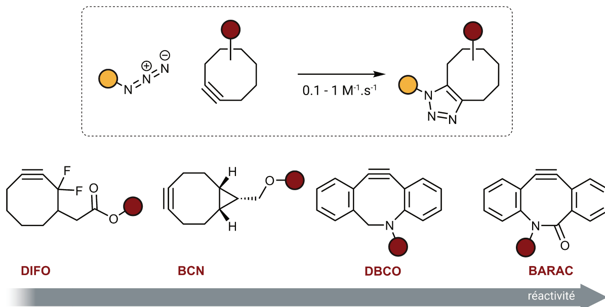
Figure 6 Strain-Promoted Alkyne Azide Cycloaddition (SPAAC). Les alcynes cycliques contraints de type cyclooctyne réagissent spontanément avec les azotures pour former un cycle triazole stable. Différentes générations de cyclooctynes ont été développées pour améliorer la vitesse de la réaction. Pour utiliser cette approche, le rapporteur chimique devra nécessairement porter le groupement azoture car les cyclooctynes sont trop encombrants et perturberaient l'étape d'incorporation métabolique.
