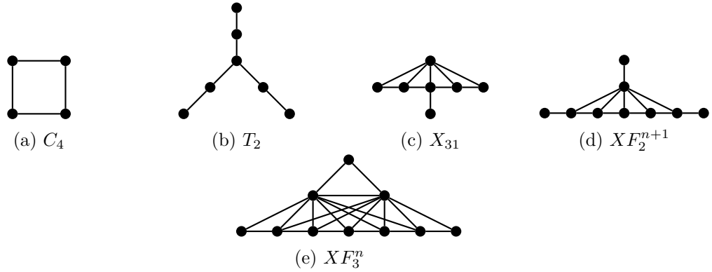
Figure 1.: Sous-graphes induits interdits pour les graphes d'intervalles
