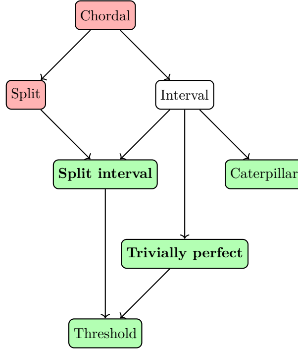
Figure 9.: Complexité de PIG-completion sur différentes sous-classes de graphes chordaux.
