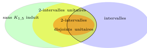
Figure 3.: Les graphes d'intervalles sans K_{1,5} induit ne sont pas contenus dans la classe des graphes de 2-intervalles disjoints unitaires. La classe des graphes de 2-intervalles unitaires est une superclasse des graphes de 2-intervalles disjoints unitaires, et s'étend à toute l'intersection des graphes sans K_{1,5} induit et des graphes d'intervalles.
