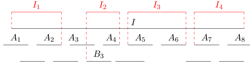
Figure 4.: L'intervalle I intersecte 8 intervalles disjoints. En rouge, le 4-intervalle retourné par l'algorithme.
