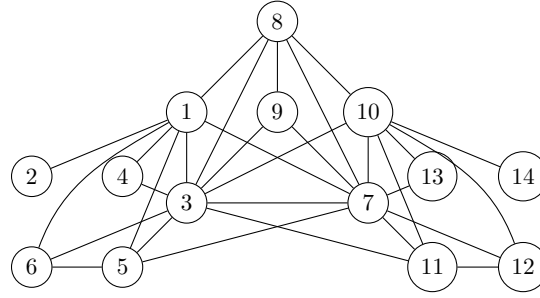
Figure 5.: Un graphe d'intervalles qui est sans K_{1,5} mais pas un graphe de 2-intervalles disjoints unitaire.
