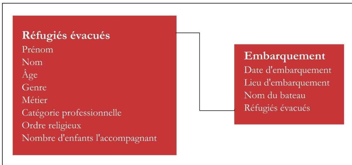
Schéma 55 : Schéma relationnel de la base de données sur les réfugiés évacués par voie maritime par les consulats français en Espagne.
