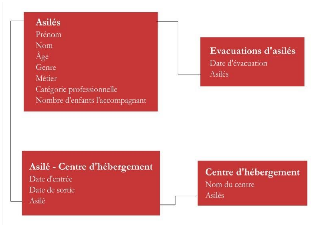
Schéma 56 : Schéma relationnel de la base de données sur les asilés de l'ambassade de France à Madrid.
