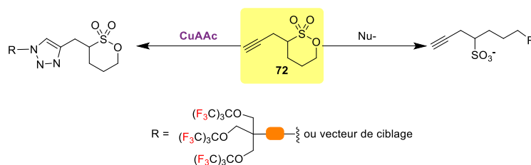
Schéma 50: Modularité de la sultone propargylique 72 pour le développement de sondes IRM ^{19}\text{F}
