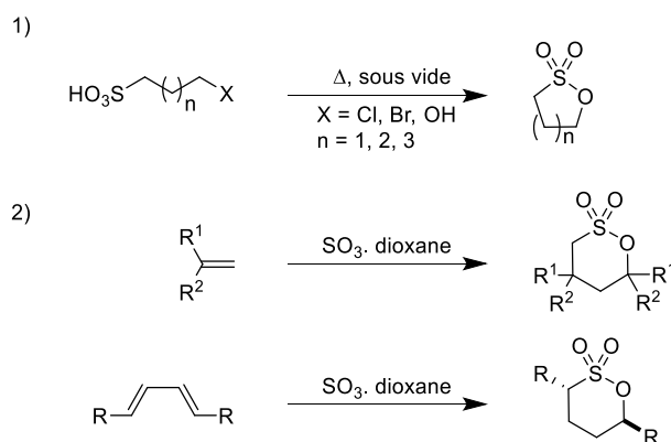
Schéma 20: Stratégies de synthèse classique de sultones
