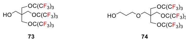
Schéma 22 : Structure des deux alcools polyfluoro-tert-butoxylés
