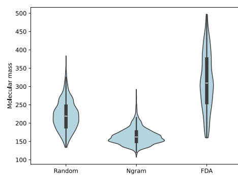
(d) g/mol
