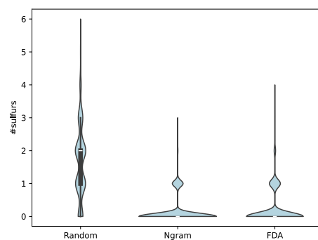
(p) #sulfurs
