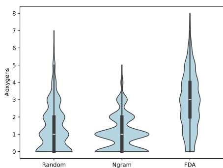
(o) #oxygens
