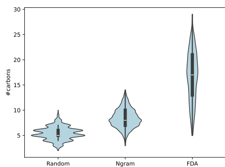
(g) #carbons
