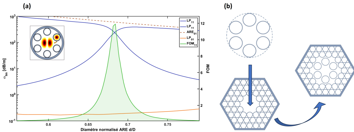
Figure 3.12 – (a) Accord de phase entre le mode LP_{11} du cœur d'air et LP_{01} des tubes [82]. (insert) Illustration schématique du couplage de ces modes. (b) Représentation de l'insertion d'une maille tubulaire dans une maille Kagomé donnant une fibre dite hybride.
