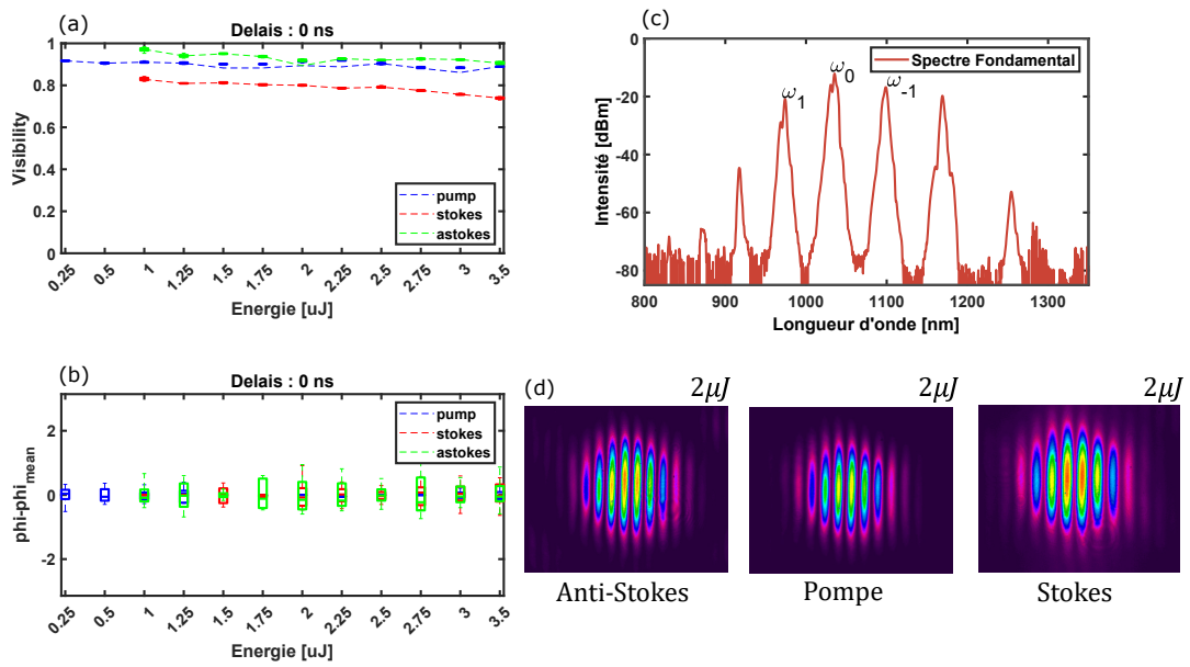
Figure 5.3 – (a-b) Visibilité et phase relative extraite des franges d’interférence à délai nul (référence) obtenue en fonction de l’énergie des deux impulsions de 3 ps. (c) Spectres Raman utilisé pour faire les mesures sur la visibilité (première raie Stokes \omega_{-1} , première raie anti-Sotkes \omega_1 et la pompe \omega_0 ). (d) Exemples de Franges d’interférence obtenues à la caméra infrarouge.
