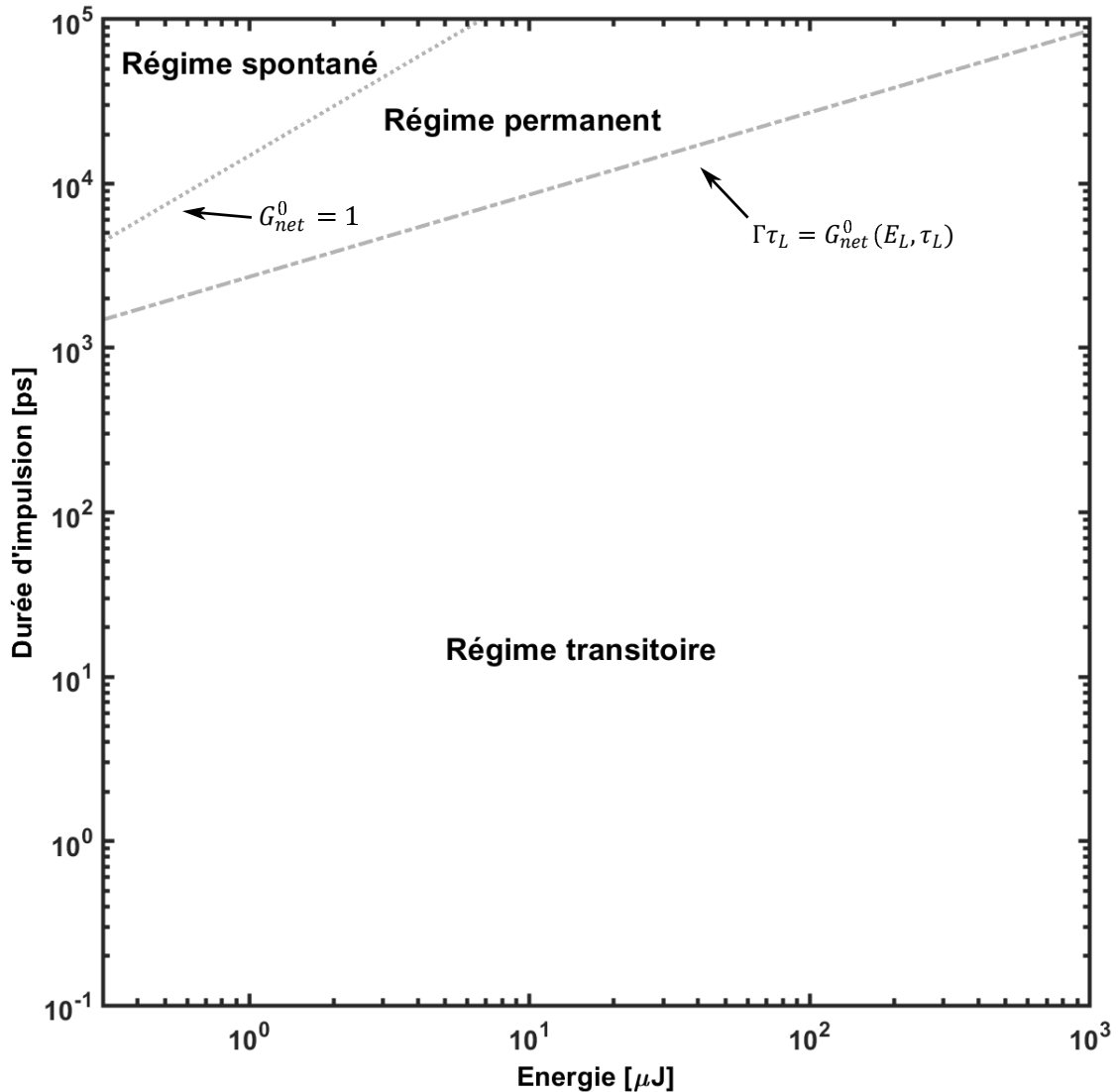
Figure 2.7 – Tracé des 3 régimes de diffusion Raman stimulée dans l'espace \tau_L et \epsilon_L déterminés pour les paramètres expérimentaux L = 3 m, R = 19,5 \mu\text{m} , g_R = 1,3 \times 10^{-11} m/W et \Gamma = 2 GHz . La ligne noire solide montre la transition entre les régimes de diffusion Raman spontanée et stimulée ( G_{net}^0 = 1 ). La ligne noire en pointillées met en évidence, dans le régime stimulé, la transition entre les régimes transitoire et permanent ( G_{net}^0 = \Gamma\tau_L ) .
