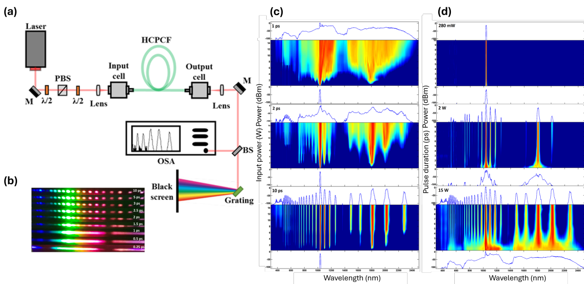
Figure 4.6 – (a) Rappel du schéma du dispositif expérimental et spectre Raman généré dans la HCPCF à CI envoyé vers un écran noir positionné après un réseau de diffraction. (b) La structure spectrale passe d'un peigne de fréquences à un supercontinuum, ici pour une puissance fixe de la pompe de 10 W. (c) Graphiques montrant la puissance spectrale mesurée en fonction de la puissance moyenne de la pompe à l'entrée de la fibre, pour des durées d'impulsion de pompe de 1 ps, 2 ps et 10 ps. (d) Graphiques montrant la puissance spectrale en fonction de la durée de l'impulsion de la pompe, avec une puissance moyenne de 280 mW, 2 W et 15 W à l'entrée de la fibre.
