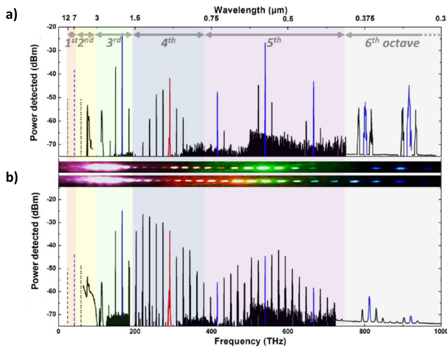
Figure 1.6 – Peigne Raman généré sur plus de 5 octaves en régime ps [37], (a) dans le cas d'une polarisation de pompe linéaire et (b) avec une polarisation de pompe circulaire. La pompe en rouge, les raies vibrationnelles Stokes et anti-Stokes en bleu, et les raies rotationnelles Stokes et anti-Stokes en noir.
