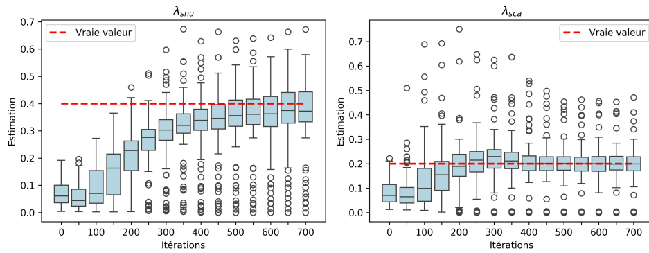
Figure 4.16 – Evolution de la valeur des paramètres d'échelle \lambda_\nu, \nu \in \Omega_{indiv} pendant la procédure d'inférence, sous l'hypothèse nulle \lambda_{R\_RGRmax}, \lambda_{LA\_RERmax} = 0 , au cours des itérations. Les boxplots sont affichés toutes les 50 itérations, la ligne rouge en pointillés représente la vraie valeur utilisée pour simuler les données. Les résultats ont été obtenus sur 100 répétitions.
