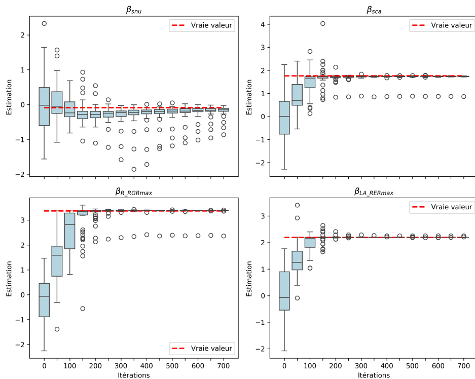
Figure 4.21 – Evolution de la valeur des paramètres de localisation \beta_\nu, \nu \in \Omega_{indiv} pendant la procédure d'inférence, au cours des itérations. Les boxplots sont affichés toutes les 50 itérations, la ligne rouge en pointillés représente la vraie valeur utilisée pour simuler les données. Les résultats ont été obtenus sur 100 répétitions, réalisées sur un même jeu de données.
