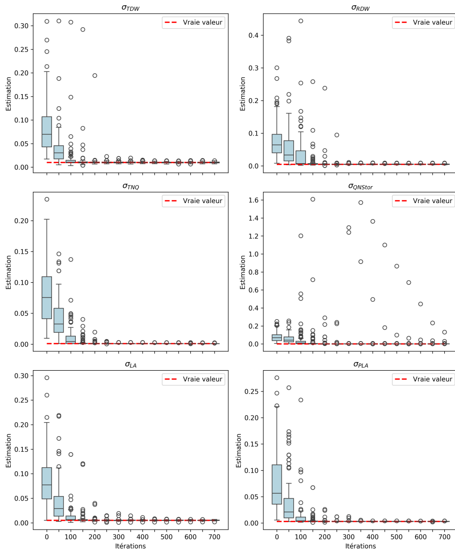
Figure 4.8 – Evolution de la valeur des paramètres de variance des résidus \sigma_\nu, \nu \in \Omega_{output} pendant la procédure d'inférence, au cours des itérations. Les boxplots sont affichés toutes les 50 itérations, la ligne rouge en pointillés représente la vraie valeur utilisée pour simuler les données. Les résultats ont été obtenus sur 100 jeux de données simulés.
