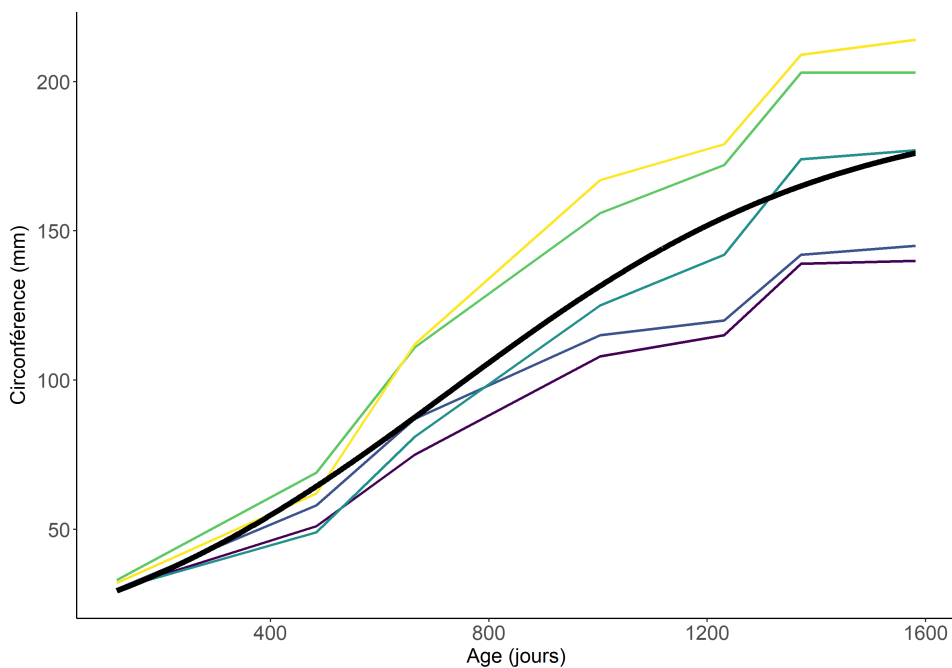
Figure 1.2 – Evolution au cours du temps (en jours) de la circonférence (en mm) du tronc de cinq orangers. La courbe noire épaisse correspond à une courbe de croissance logistique ajustée sur les données.
