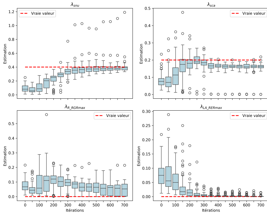
Figure 4.22 – Evolution de la valeur des paramètres d'échelle \lambda_\nu, \nu \in \Omega_{indiv} pendant la procédure d'inférence, au cours des itérations. Les boxplots sont affichés toutes les 50 itérations, la ligne rouge en pointillés représente la vraie valeur utilisée pour simuler les données. Les résultats ont été obtenus sur 100 répétitions, réalisées sur un même jeu de données.
