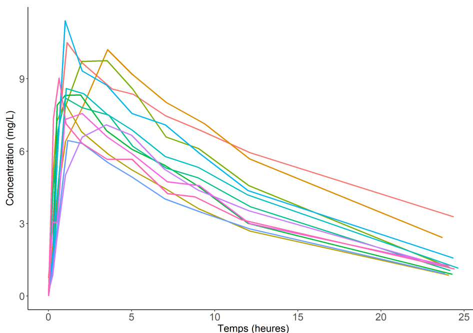
Figure 1.1 – Concentration de théophylline mesurée au cours du temps chez 12 sujets d'une étude pharmacologique
