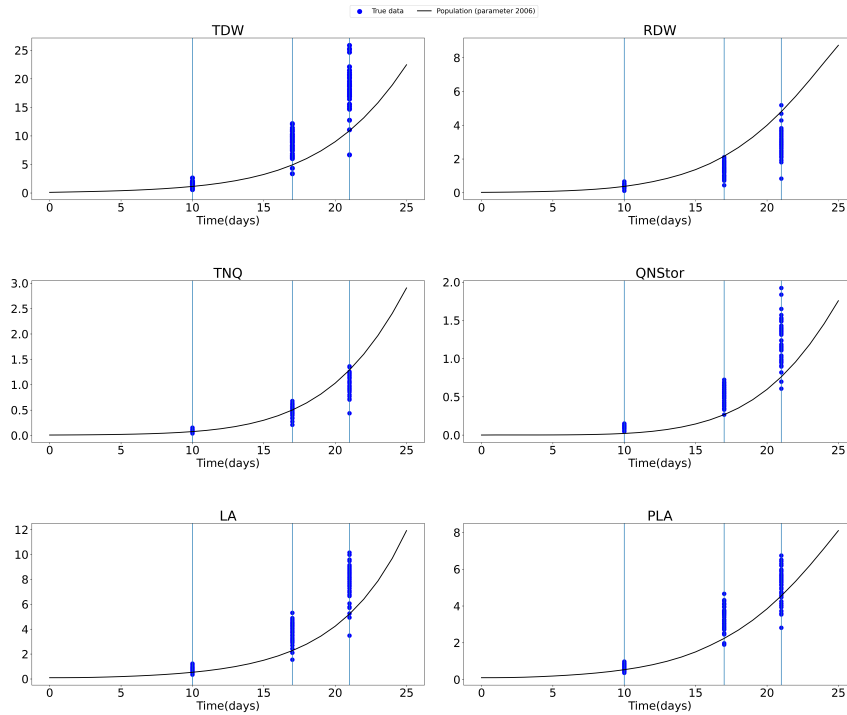
Figure 4.4 – Comparaison des données réelles d' Arabidopsis thaliana (points bleus) et des réponses simulées avec le modèle ARNICA, à partir des paramètres \varphi^{ref} (ligne noire).
