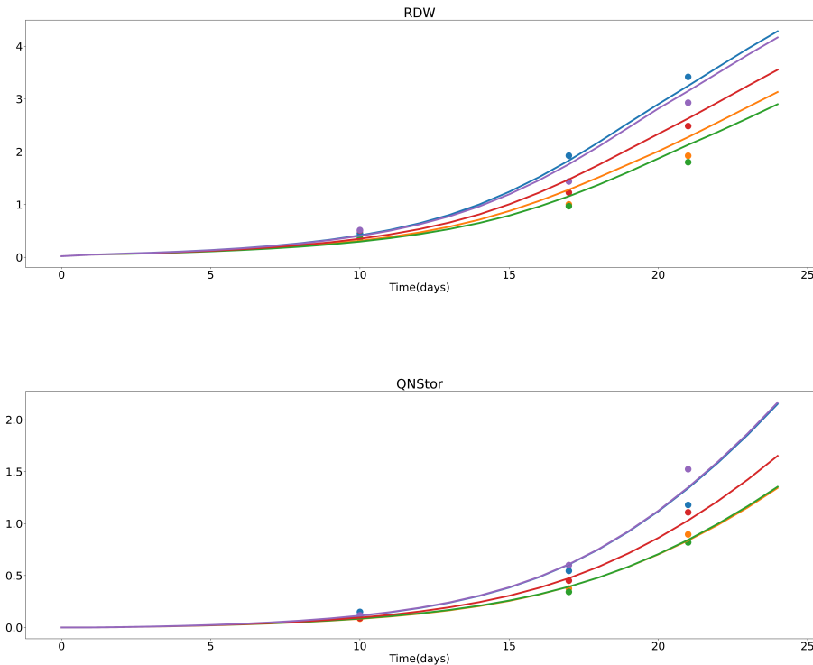
Figure 4.10 – Différentes courbes d’ajustement individuel pour 5 individus, et les données réelles correspondantes (les points) associées par couleur. Les courbes sont obtenues comme des sorties du modèle ARNICA à partir d’un paramètre individuel estimé.
