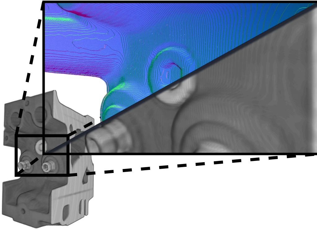
FIGURE 3.3 – Artéfacts typiques causés par le tracé de rayon volumique et leur impact sur les surfaces TROA. Quadrant haut : Vecteurs normaux à une surface TROA, ici choisie de telle sorte à ce qu'elle corresponde à la silhouette du moteur. Quadrant bas : Zoom sur le rendu volumique.
