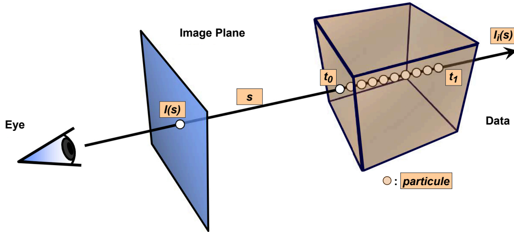
FIGURE 2.2 – Schéma de principe de lancer de rayon volumique. Copyright Siemens Healthcare GmbH , les annotations ont ajoutées pour ce manuscrit. Les notations sont détaillées ci-après.
