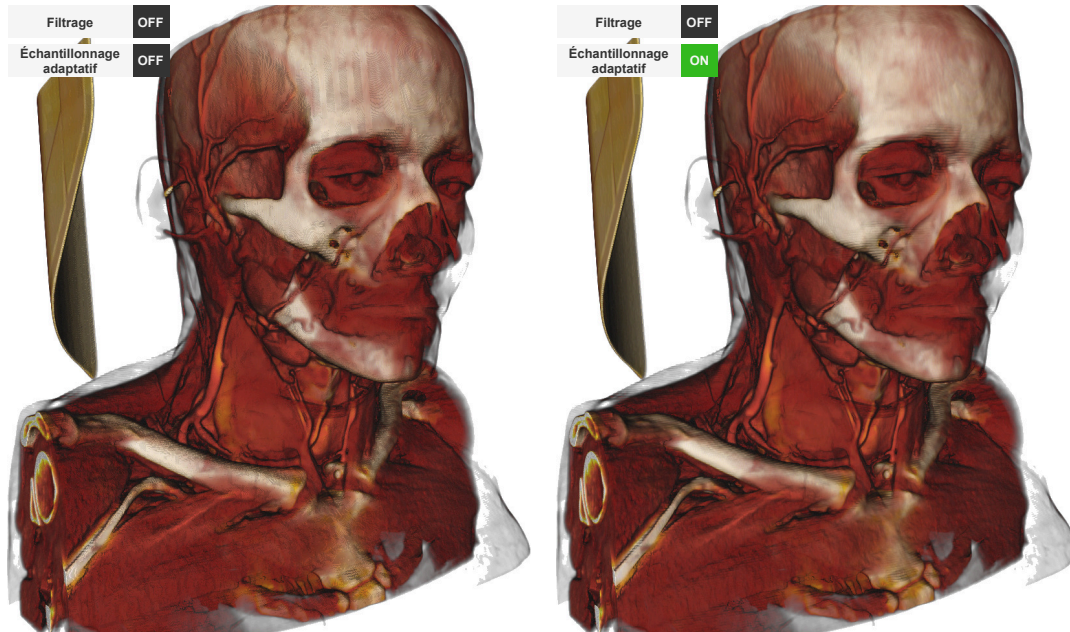
FIGURE B.2 – Influence de l'échantillonnage adaptatif sur les surfaces TROA, illustrée sur une image de scanner CT.
