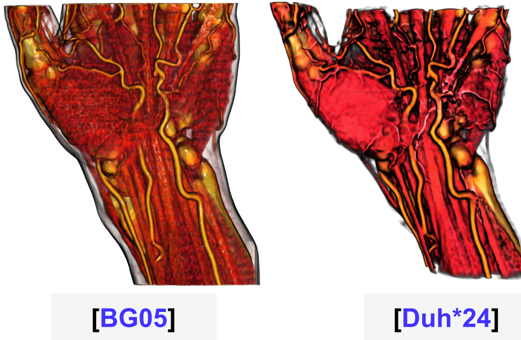
FIGURE 3.31 – Comparaison de notre effet de cel-shading basé sur les surfaces TROA à celui proposé par [BG05]. L’illustration pour [BG05] a été réalisée dans une version du logiciel dont nous avons modifié les shaders pour qu’ils soient supportés par les GPUs contemporains.
