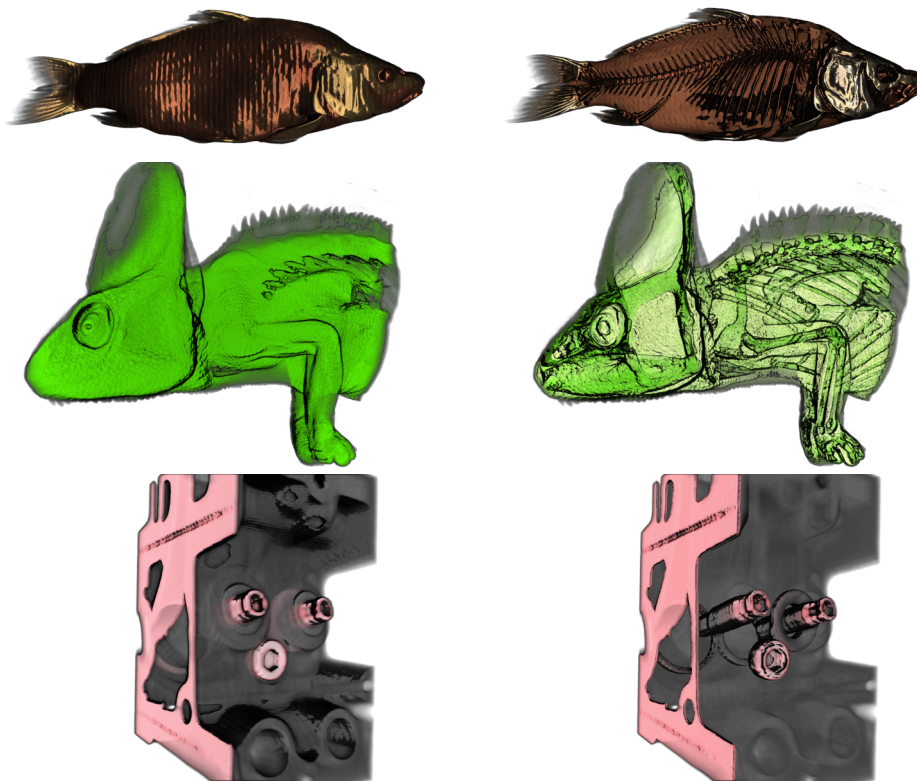
FIGURE A.2 – Notre méthode de rendu volumique en utilisant deux fonctions de transfert sur divers jeux de données, utilisés dans l'étude de la robustesse des surfaces TROA décrite dans la sous-section 3.6.2 . Les seuils d'opacité restent identiques.
