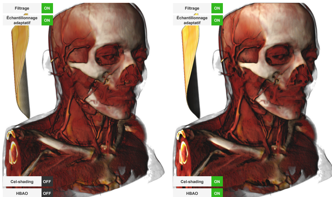
FIGURE B.6 – Combinaison du cel-shading et de l’HBAO sur une image par rendu volumique direct basé TROA, illustrée sur un scanner CT.
