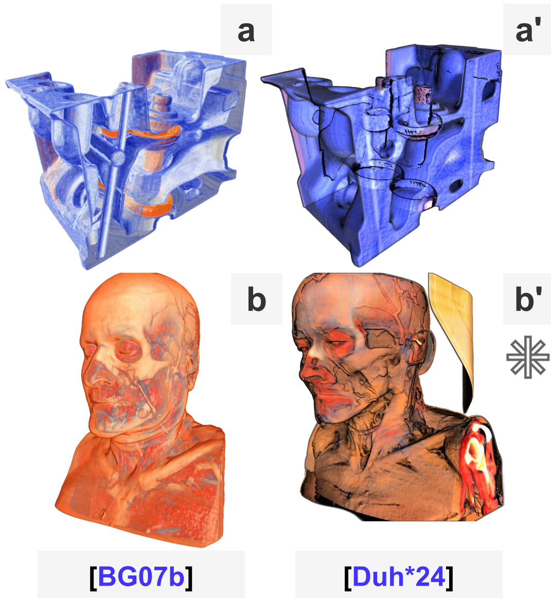
FIGURE 3.32 – Comparaison du rendu illustratif proposé par [BG07a] à notre rendu. L’illustration pour [BG07a] est extraite du travail original, Figure 7, dernière colonne (Illustration Copyright Computer Graphics Forum )
