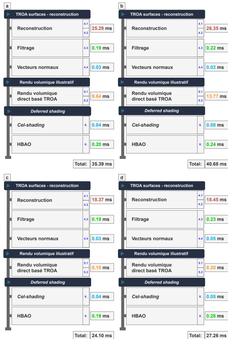
FIGURE 3.37 – Performances de notre rendu volumique basé TROA, estimé sur les jeux de données a, b, c et d. Chaque total représente le temps nécessaire à la réalisation d’une image affichée à l’écran.
