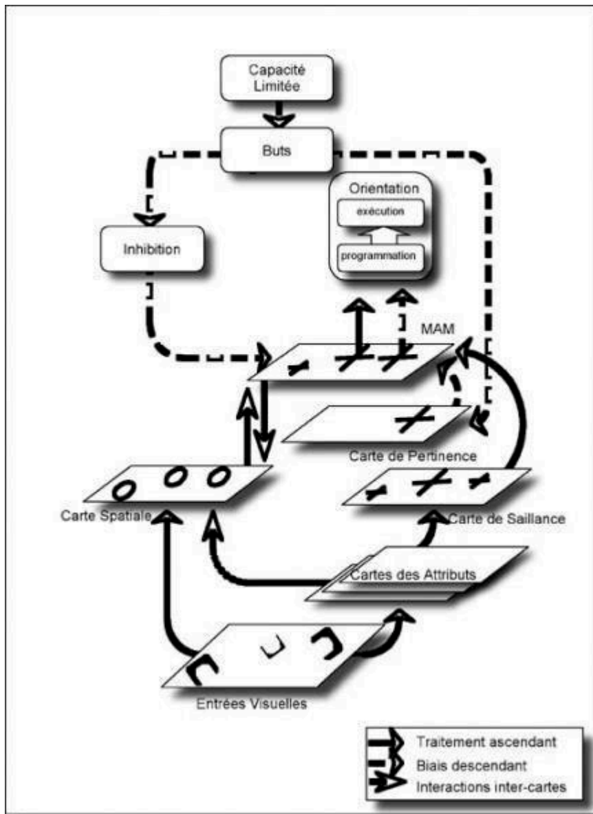
Figure 4 : Schéma du modèle MAM
