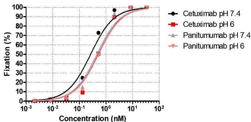
Figure 22 : Évaluation de la capacité dose réponse des anticorps de contrôle positif le Cetuximab et le Panitumumab aux pH physiologique (7,4) et acide (6) sur la protéine hEGFR-hFc.
