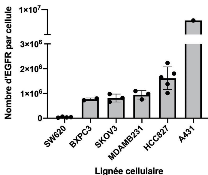
Figure 26 : Quantification du nombre de récepteurs EGFR humain par cellules pour les six lignées étudiées. Cette quantification est basée sur le Quantum Simply Cellular kit (Bangs Laboratories). Toutes les lignées ont été quantifiées au moins trois fois sauf A 431 (n=1) et BxPC3 (n=2).
