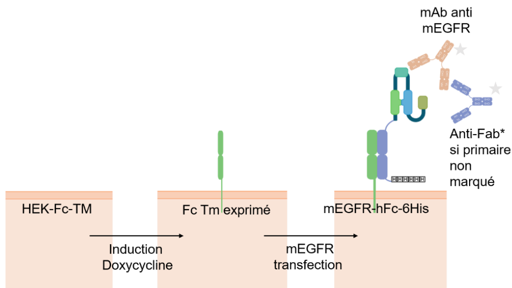
Figure 35 : Schéma explicatif de l'expression transmembranaire induite par la doxycycline du Fc couplé au domaine extracellulaire de l'EGFR murin sur la lignée stable HEK-FcTM. Un anticorps primaire marqué ne nécessite pas d'anticorps secondaire marqué mais si l'anticorps primaire n'est pas marqué, l'anticorps secondaire marqué est indispensable.
