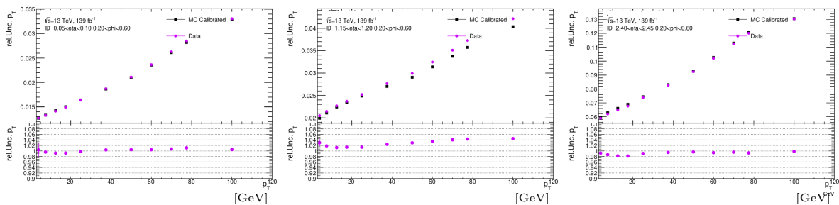
(a) 0.05 < \eta < 0.10
