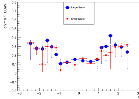
(d) dr_2 as a function of \eta
