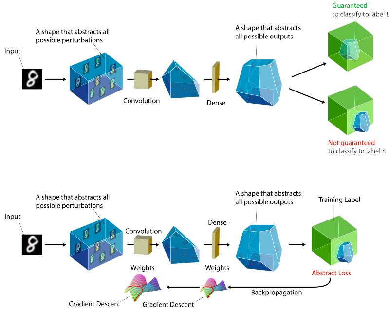
Figure A.2: Sur-approximation des sorties de réseaux de neurones pour la vérification et l'entraînement. Crédit : ETH Zurich SRI Lab.
