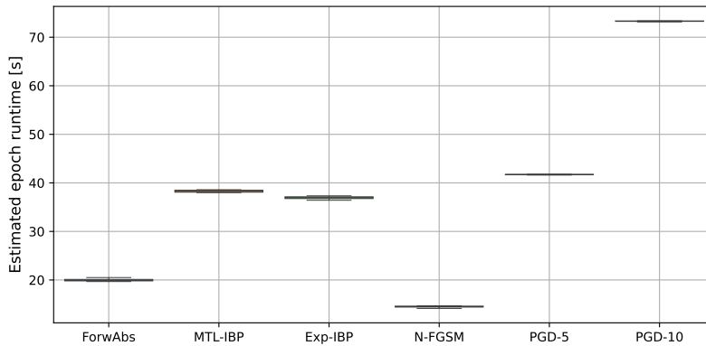
(b) CNN-5.
