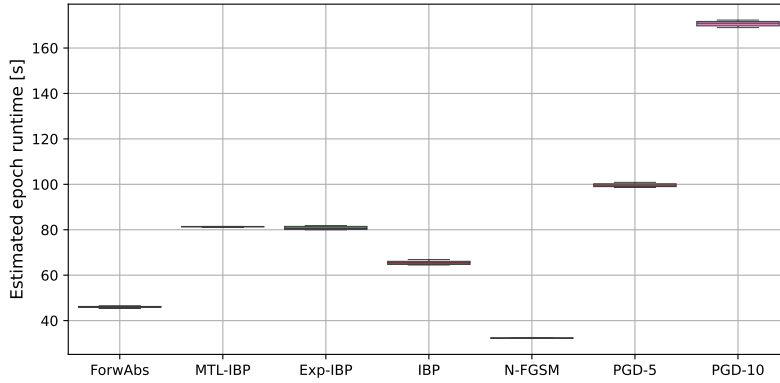
(a) CNN-7.
