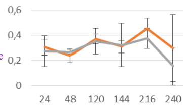
Tyrosine
