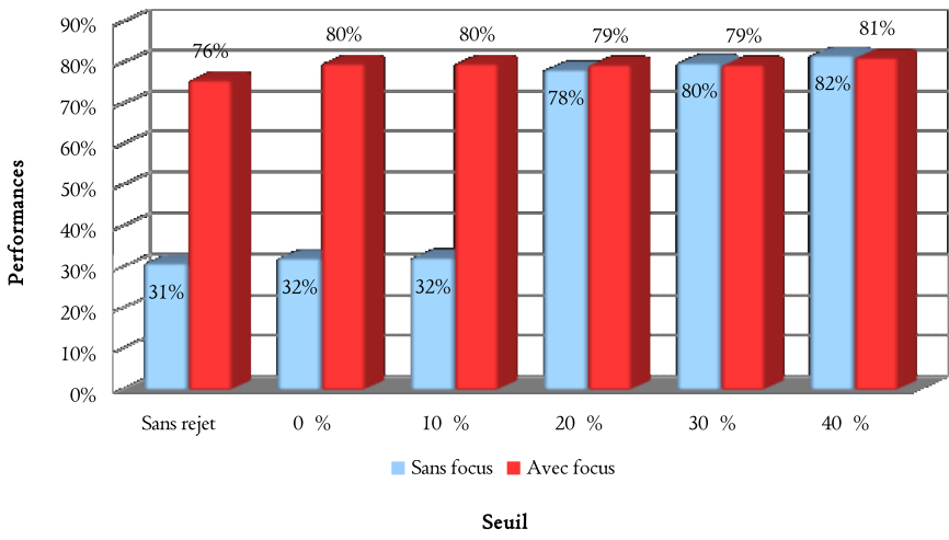
Figure 7.5. Évolution de la précision du système en fonction de la contrainte de seuil.
