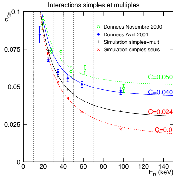
FIG. VI.8: Résolutions \sigma_{Q_n} expérimentales de novembre 2000 (cercles vides) et avril 2001 (cercles pleins) comparées aux écarts-types \sigma_{D^s} avec ( \times ) et sans ( + ) sélection des interactions simples. Sont aussi représentées les lois \sigma_{Q_n}(E) (cf équation VI.2) pour C=0,050 , C=0,040 (valeur moyenne des données expérimentales), C=0,024 (ajustant au mieux les valeurs \sigma_{D^s} sans sélection des interactions simples) et C=0,0 (ajustant au mieux les valeurs \sigma_{D^s} avec sélection des interactions simples).
