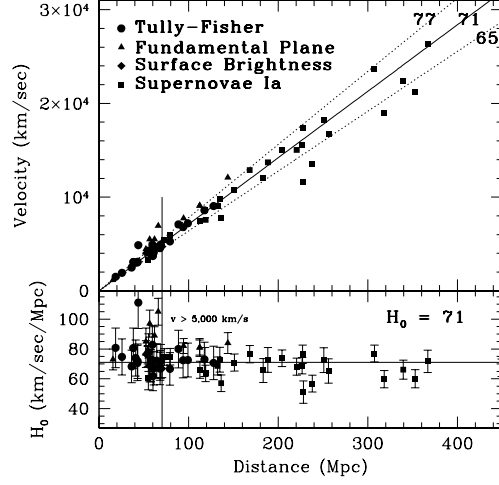
FIG. I.1: Figure du haut : diagramme des vitesses de récession en fonction des distances à la Terre pour un certains nombres d'objets servant d'indicateurs de distance. Une pente H_0 = 71 \text{ km/s/Mpc} est représentée, ainsi que les lignes à \pm 10\% autour de cette valeur. Figure du bas : Pente H_0 en fonction de la distance. Extrait de [4].
