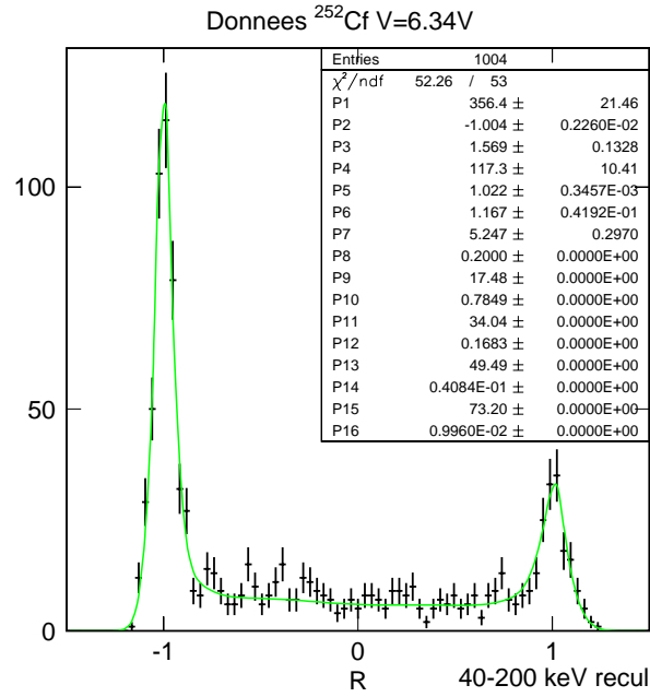
FIG. V.24: Ajustement par la fonction CORNUD des données de calibration 252 Cf sous +6,34 V de polarisation.
