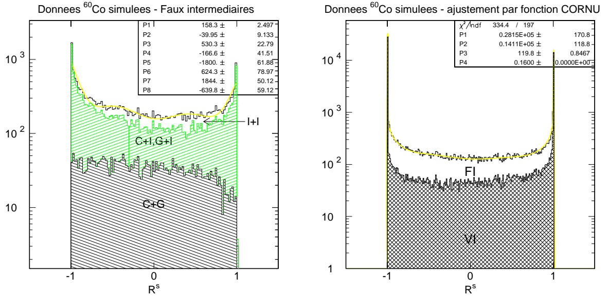
FIG. V.15: Figure de gauche : ajustement de R^s pour la population FI par la fonction polynômiale \mathfrak{Z}(R) . Figure de droite : ajustement de R^s par la fonction CORNU. La population de vrais intermédiaires (VI) est représentée en hachurée.
