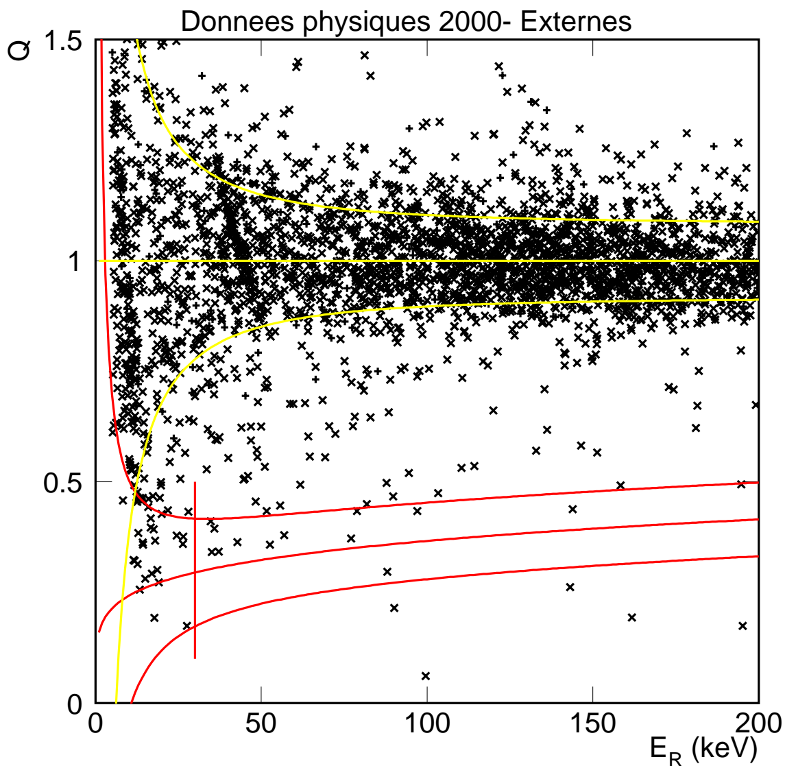
FIG. VI.14: Bi-plot ( E_R, Q ) des événements externes pour les enregistrements de l'année 2001. Les événements pour lesquels E_i > E_g sont représentés par le symbole +.
