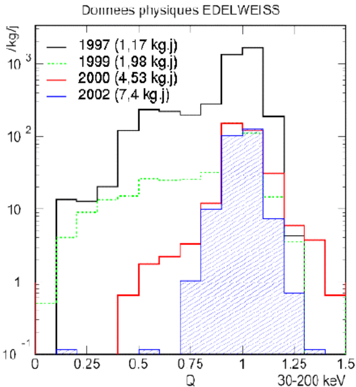
FIG. VI.20: Histogramme normalisé en \text{kg}^{-1}\cdot\text{j}^{-1} de la variable Q pour les données physiques enregistrées par l'expérience EDELWEISS au cours des campagnes 1997 [131], 1999 [159], 2000 [188] et 2002 [161].
