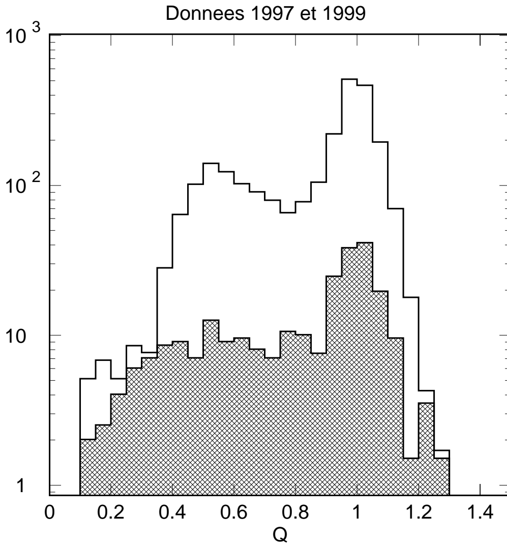
FIG. III.18: Histogramme du facteur de quenching Q normalisé en \text{kg}^{-1}\cdot\text{jour}^{-1} pour les données enregistrées avec les détecteurs Ge4 en 1997 et Ge7 en 1999 (hachuré) sur la plage d'énergie de recul 20-100 keV.
