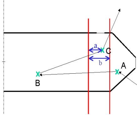
FIG. V.10: Illustration de la construction des signaux E_g^s et E_i^s avec une particule interagissant successivement dans les volumes V_C , V_G et V_I . On obtient pour l'événement associé : E_i^s = 0 + E_t^s(B) + P_C \cdot E_t^s(C) et E_g^s = E_t^s(A) + 0 + (1 - P_C) \cdot E_t^s(C) , avec P_C = \frac{(b-a)}{b} .
