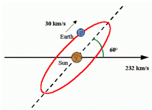
FIG. II.5: Schéma illustrant la rotation de la Terre et déplacement du Soleil dans un référentiel associé au halo.
