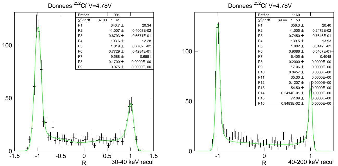
FIG. V.25: Ajustement par la fonction CORNUD des données de calibration 252 Cf sous +4,78 V de polarisation.
