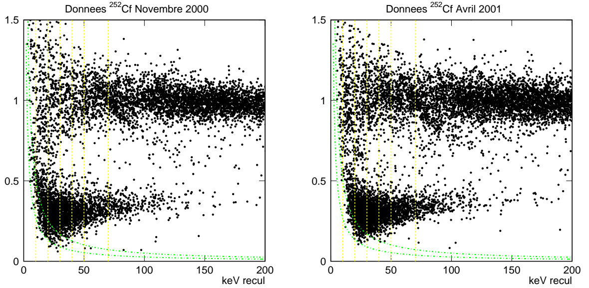
FIG. VI.1: Bi-plot (E_R, Q) pour les données de calibration ^{252}\text{Cf} de novembre 2000 et avril 2001. Sont représentés les seuils centre ( E_i = 5,1 \text{ keV} ) et garde ( E_g = 2,7 \text{ keV} ) (tirets). On a également tracé en pointillés les limites des intervalles d'étude 10-20, 20-30, 40-50, 50-70 et 70-200 keV.
