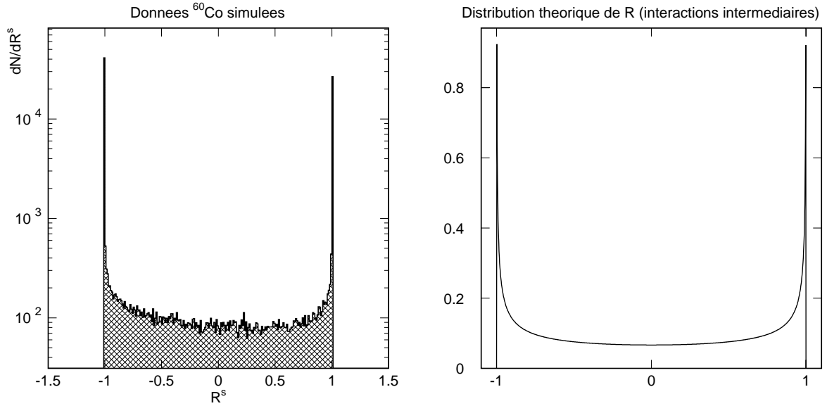
FIG. V.8: figure de gauche : distribution R^s pour la simulation ^{60}\text{Co} pour E_{\text{recoil}} > 30 \text{ keV} , avec un choix arbitraire r_b = 1 \text{ mm} et R_c = 2,4 \text{ cm} . figure de droite : distribution attendue de la variable R d'après le modèle en boule pour une répartition uniforme d'interactions dans le volume intermédiaire V_I .
