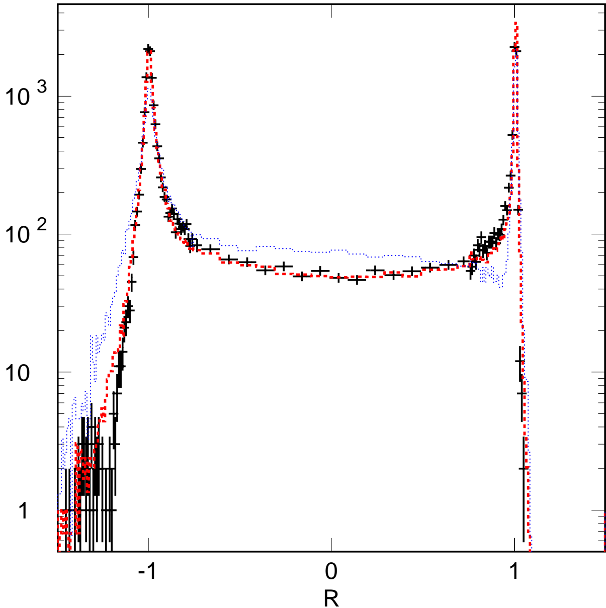
FIG. V.14: Superposition des variables R et R^{sd} pour les données ^{60}\text{Co} expérimentales ( V=+6,34V ) (croix) et simulées d'après le modèle linéaire ( R_{Ce}=21,0 mm, R_G=28,0 mm, pointillées) et le modèle en boule ( r_b = 3,5 mm et R_c = 24,50 mm, tirets). La plage d'étude est ici fixée à l'intervalle 30-1400 keV.
