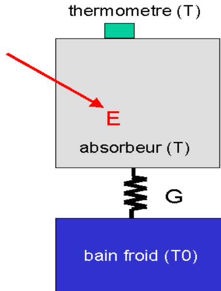
FIG. III.3: Schéma du système bolomètre + bain froid permettant une modélisation du principe de détection d'un dépôt d'énergie E dans l'absorbeur (représenté ici par la flèche).
