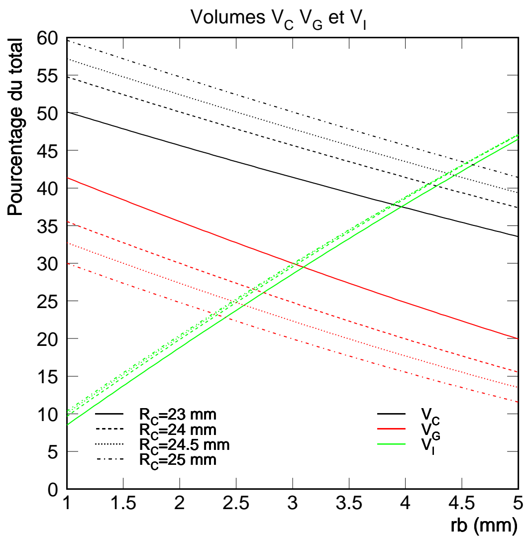
FIG. C.3: Volumes V_C , V_G et V_I en fonction de r_b sur la plage [1,0, 5,0 \text{ mm}] pour R_C=23,0, 24,0, 24,5 et 25,0 \text{ mm} .
