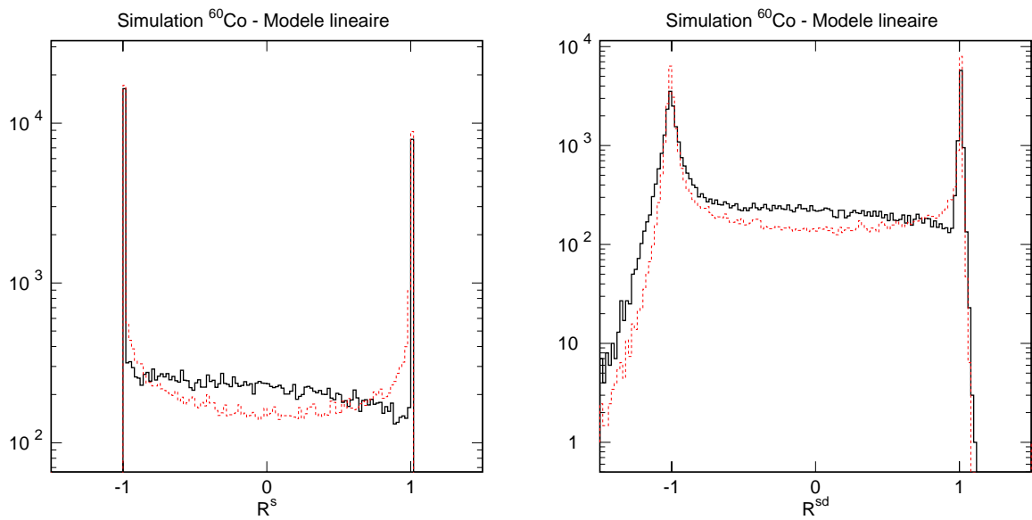
FIG. V.11: figure de gauche : distribution R^s pour la simulation ^{60}\text{Co} construites par simulation pour E_{\text{recul}} > 30 \text{ keV} pour un choix arbitraire R_{C_e} = 21,0 \text{ mm} et R_G = 28,0 \text{ mm} . Est aussi représenté en pointillés la distribution associée au modèle en boule pour r_b = 3,5 \text{ mm} et R_C = 24,5 \text{ mm} donnant les mêmes valeurs R_{C_e} et R_G . figure de droite : distribution R^{sd} : dégradation des distributions R^s par la résolution expérimentale (trait plein : pour le modèle linéaire, pointillés : pour le modèle en boule).
