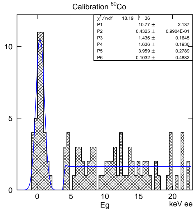
FIG. IV.13: Spectres des voies centre et garde pour une calibration avec source ^{60}\text{Co} . Le pic de bruit gaussien et le plateau correspondant aux événements de ^{60}\text{Co} sont clairement résolus. La distribution est ajustée par une fonction SEUIL s'écrivant comme la somme d'une fonction gaussienne (pour le pic de bruit) et d'une fonction erreur. Le seuil correspondant à une efficacité de 50% de détection est donné par le paramètre P5.
