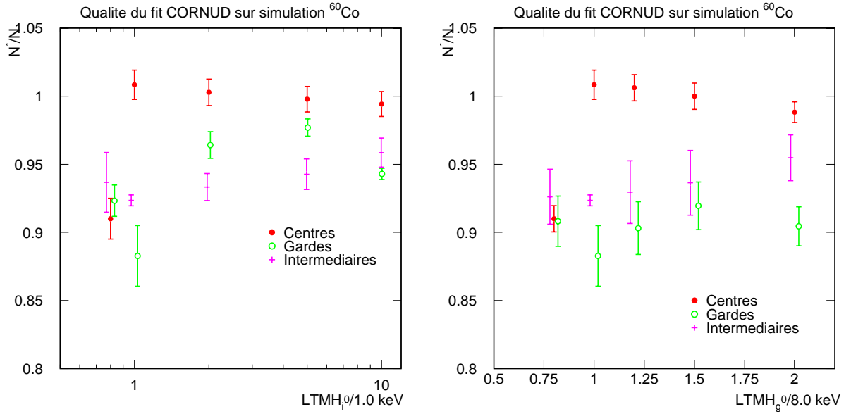
FIG. V.18: Evolution des rapports N_{C^*}/N_C , N_{G^*}/N_G et N_{I^*}/N_I en fonction du rapport LTMH_i^0/1,0 , avec LTMH_g^0 fixé à 8,0 \text{ keV} (à gauche) et en fonction de LTMH_i^0/8,0 , avec LTMH_g^0 fixé à 1,0 \text{ keV} (à droite).
