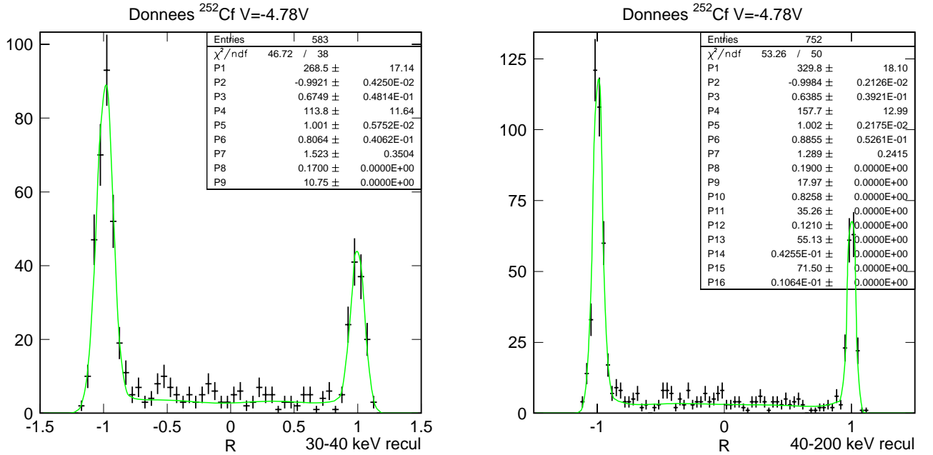
FIG. V.26: Ajustement par la fonction CORNUD des données de calibration 252 Cf sous -4,78 V de polarisation.
