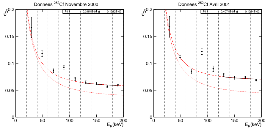
FIG. VI.4: Représentation des \sigma_{Q_\gamma}^i en fonction de l'énergie de recul pour les calibrations ^{252}\text{Cf} de novembre 2000 (à gauche) et avril 2001 (à droite). Ajustement de la distribution sur la plage 120-200 keV par la loi VI.5 avec b_c paramètre libre. On trouve b_c = 0,032 \pm 0,01 pour novembre 2000 et b_c = 0,041 \pm 0,01 pour avril 2001. On représente (tirets) la loi \sigma_{Q_\gamma} pour ces valeurs, ainsi que pour b_c=0 (pointillés). Les tranches d'énergie inférieures à 120 keV ne sont pas considérées pour l'ajustement en raison du biais induit par la bavure de la distribution en Q (visible sur la figure VI.1) due aux interactions inélastiques (cf chapitre III.2.2).
