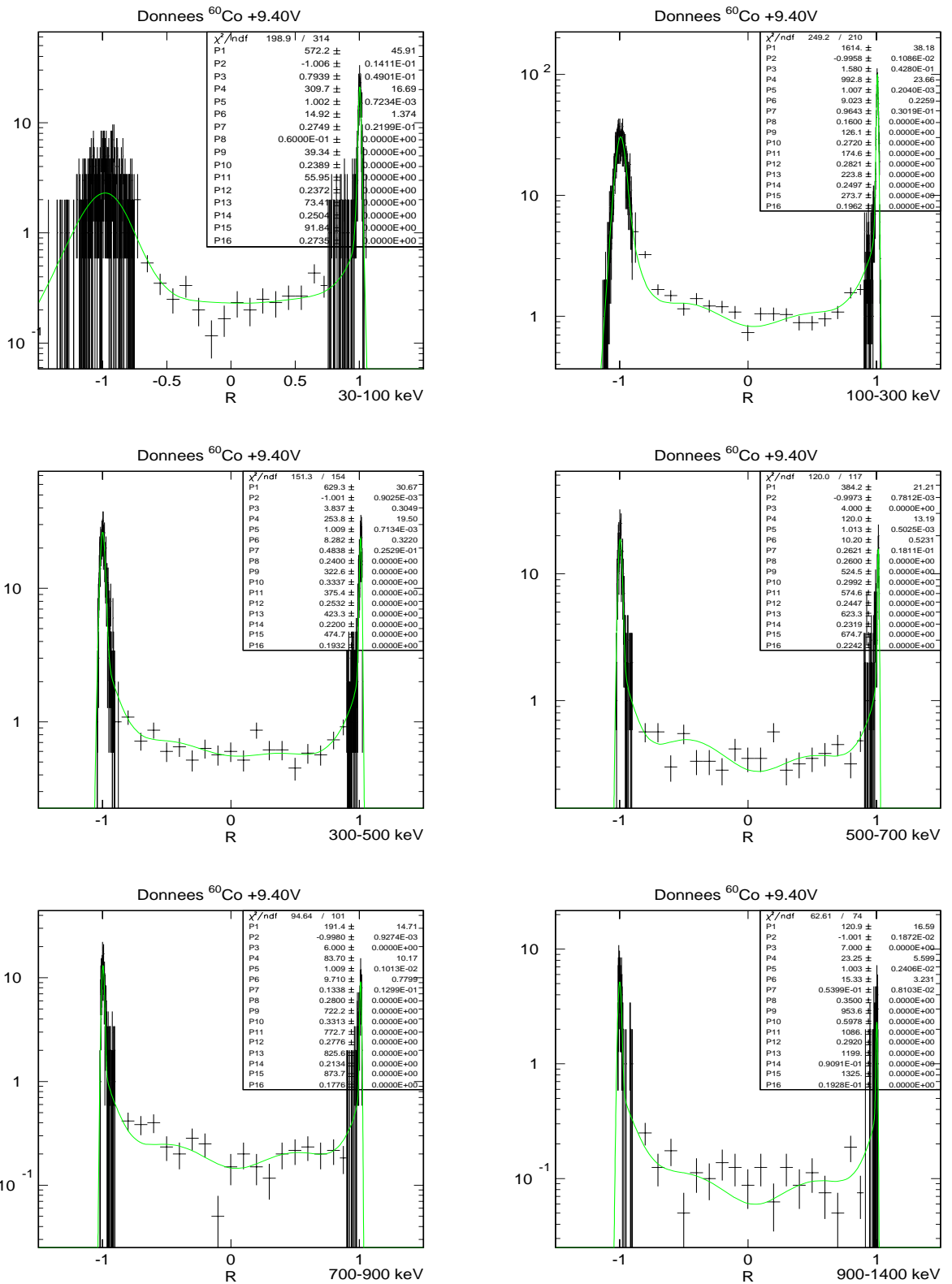
FIG. D.1: Ajustement des données expérimentales de calibration ^{60}\text{Co} pour V = +9.40\text{ V} .
