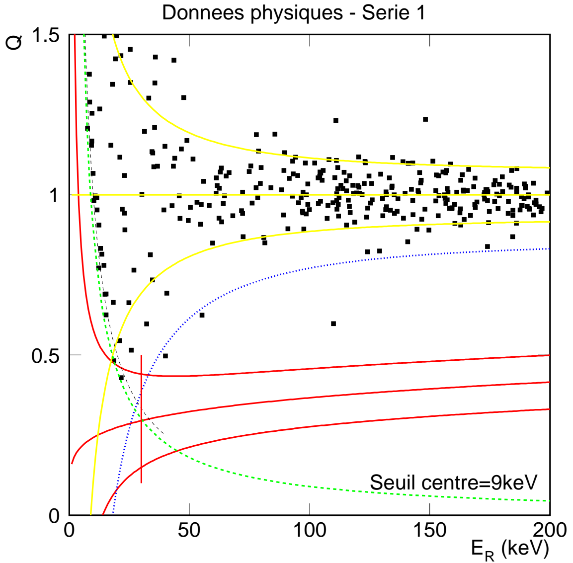
FIG. VI.11: Bi-plot (E_R, Q) des données internes de la série 1. On a tracé les lignes \gamma ( Q=1 ) et neutrons ( Q = 0,16E_R^{0,18} ) et les zones à \pm 1,645\sigma_Q autour de ces lignes (traits pleins). Sont aussi représentées la ligne correspondant à 99,9% d'efficacité sur la zone \gamma (pointillés), les hyperboles E_t=9,0 keV (seuil de la voie centre, tirets) et E_t=10,4 keV (tirets fins, jusqu'à E_R=40 keV).
