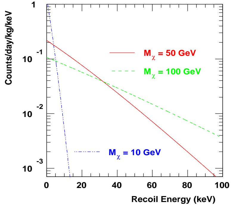
FIG. II.4: Spectres de reculs attendus dans une cible de germanium pour des WIMPs du halo ( \rho_0 = 0,3 \text{ GeV/cm}^3 et \bar{v} = 270 \text{ km}\cdot\text{s}^{-1} ) de différentes masses et ayant une section efficace de diffusion sur proton \sigma_{\omega-p} = 7 \times 10^{-6} \text{ pb} .
