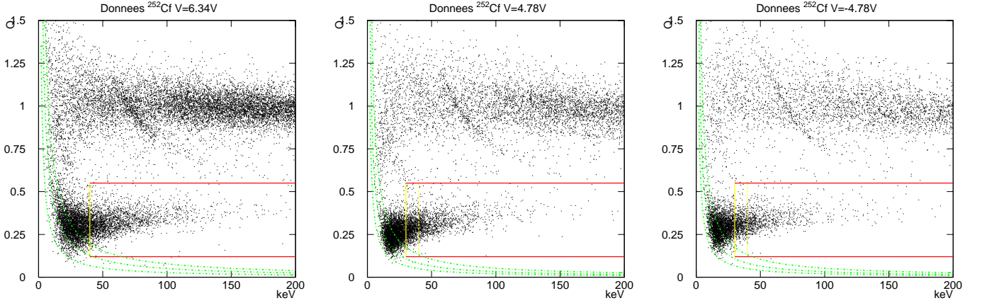
FIG. V.23: Bi-plot (E_R, Q) pour les trois séries de prises de données ^{252}\text{Cf} à +6,34 , +4,78 et -4,78 V. Les données sélectionnées pour l'analyse de la variable R correspondent à 0,15 < Q < 0,55 (rectangle). Sont également représentées les hyperboles E_i = \text{seuil}_{\text{centre}} , E_g = \text{seuil}_{\text{garde}} et E_i = \text{seuil}_{\text{centre}} + \text{seuil}_{\text{garde}} correspondant aux efficacités de 100% pour le déclenchement d'un événement centre, garde et intermédiaire.
