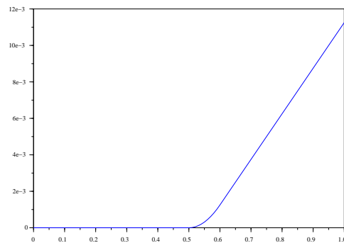
Fig 4. Graphes de la fonction phi.
