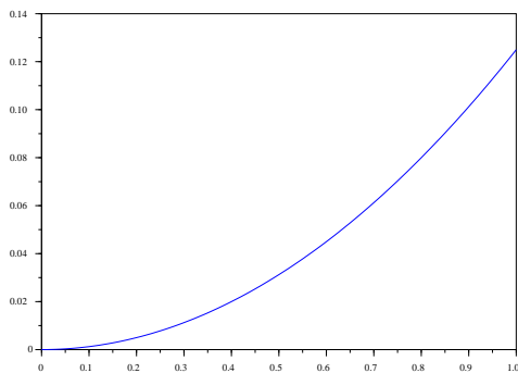
Fig 3. Graphes de la fonction f.
