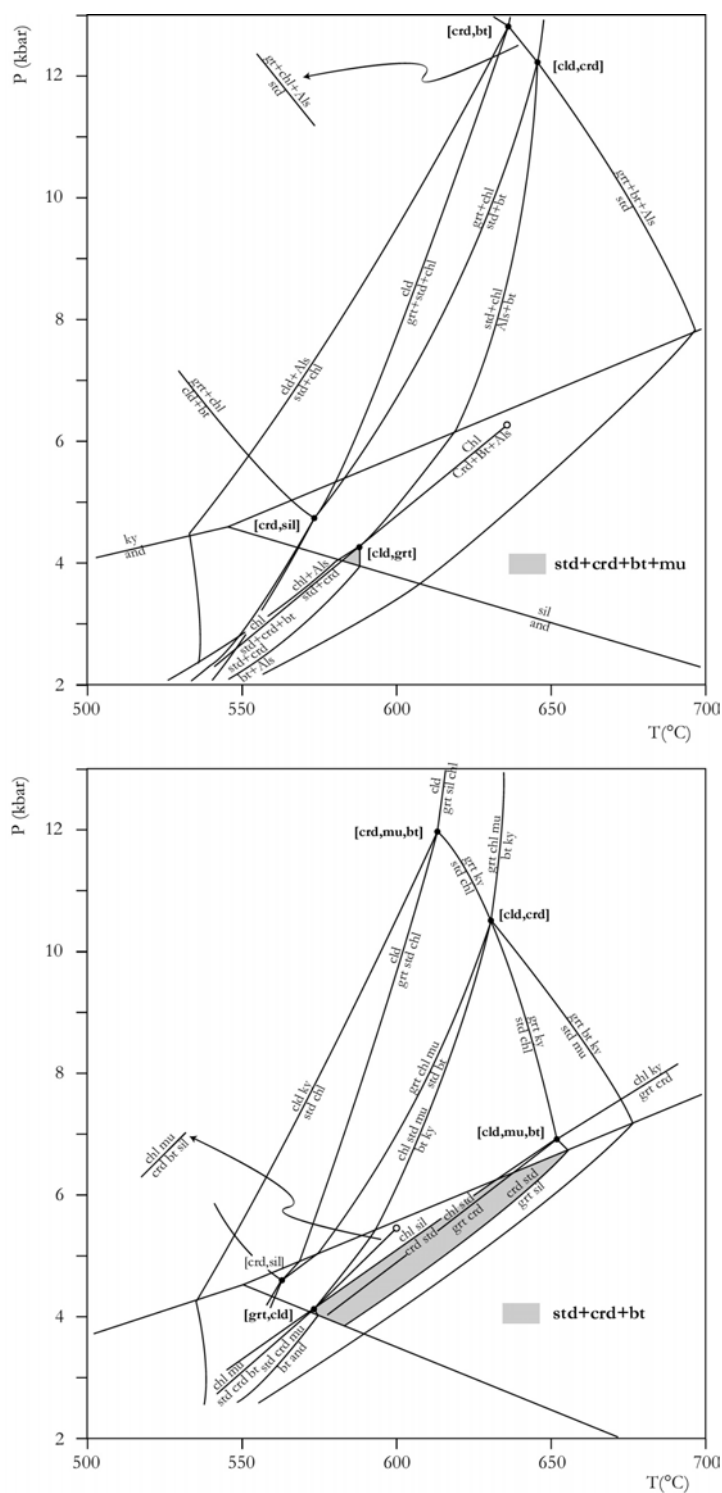
Fig. II-11: (a) Grille pétrogénétique dans le système KFMASH montrant la position des réactions univariantes (Spear, 1999). Quartz, muscovite et H 2 O sont excès. Les points noirs correspondent aux points invariants et le point blanc à l'extrémité de la réaction chl+mu+qtz=crd+bt+sil , correspond à un point invariant dans le système KFMASH. Dans cette grille, l'assemblage crd+std+bt+mu n'est stable que dans un champ PT très restreint dans le domaine PT de la sillimanite (zone grisée). (b) Grille pétrogénétique dans le système KFMASH, modifié d'après Zeh (2001). Quartz et H 2 O en excès. La différence majeure est la présence d'un point invariant supplémentaire [cld,mu,bt]. Ce point invariant permet d'expliquer la stabilité de l'assemblage std+crd+bt dans le champ de la sillimanite (zone grisée).
