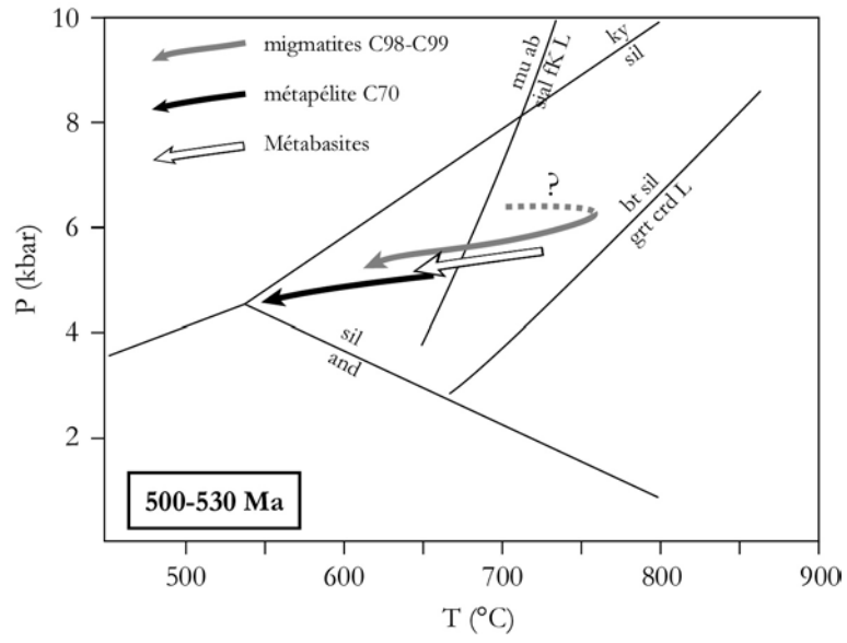
Fig. II-16: Compilation des conditions PT et trajets PT associés à la déformation Cambrienne (500-530 Ma) obtenus sur les migmatites C98-99, la métapélite C70 et les métabasites.
