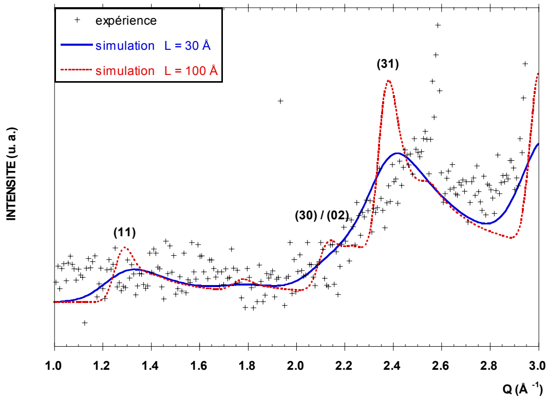
Figure IV.15 : Simulation du spectre de poudre pour la phase p(3 \times 2) issue des calculs ab initio à T = 0 \text{ K} , influence de la longueur de cohérence L ( L = 30 \text{ \AA} et L = 100 \text{ \AA} )
