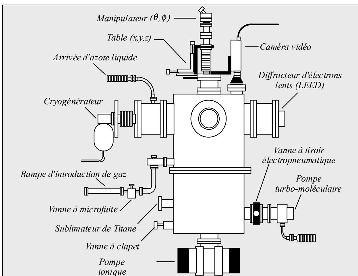
Figure II.1 : L'enceinte ultravide
