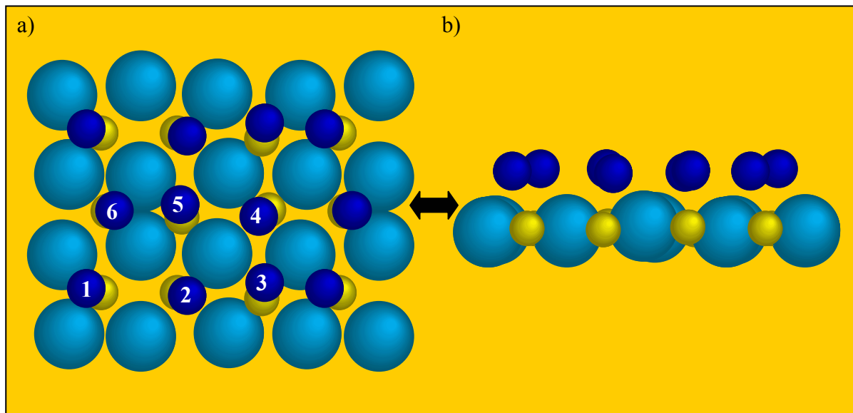
Figure IV.10 : Nouvelle structure générée par le programme TENSOR LEED, la structure de départ est issue des calculs ab-initio à T \approx 200 K. a) vue de dessus, b) vue de côté.
