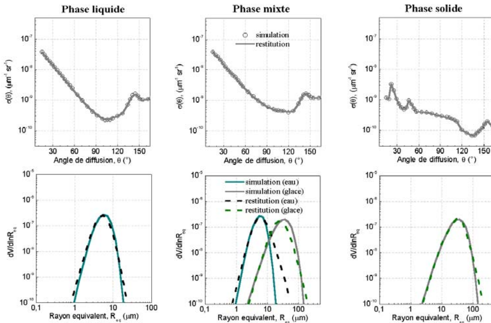
Figure I-3.3. Inversion de sections efficaces de diffusion volumique simulées pour trois granulométries types caractéristiques de la composition microphysique des nuages
