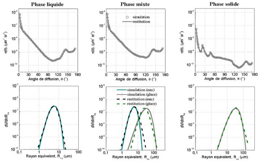
Figure I-3.2. Inversion de sections efficaces de diffusion volumique simulées pour trois granulométries types caractéristiques de la composition microphysique des nuages
