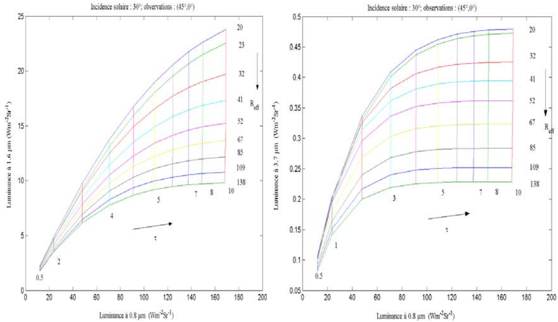
Figure III-3.1. Tables d'interpolation obtenues associées à une incidence solaire de 30° et des angles d'observations du satellite de (45°,0°). Relations obtenues entre les luminances à 0.8 μm et 1.6 μm (à gauche) et entre les luminances à 0.8 μm et 3.7 μm (à droite) pour 9 rayons effectifs ( R_{\text{eff}} ) et 14 épaisseurs optiques ( \tau ).
