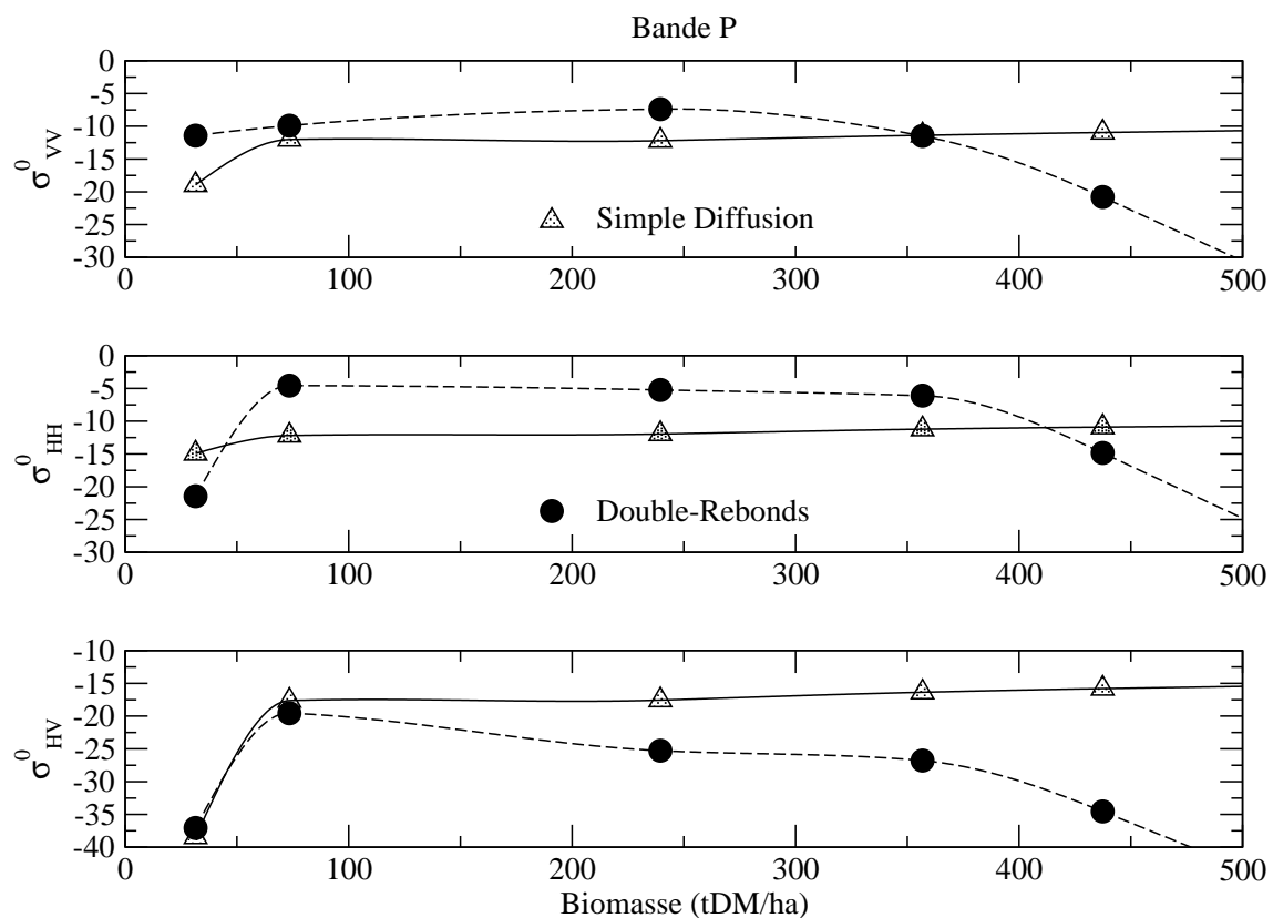
FIG. II.19 – Simulations du coefficient de rétrodiffusion des doubles-rebonds (cercles) et de la simple diffusion (triangle) en fonction de la biomasse en tDM/ha pour toutes les polarisations et avec \theta_i = 35^\circ et f = 0.44\text{GHz} .
