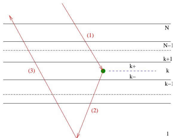
FIG. II.8 – Trajet d'une onde incidente et diffusée, dans le cas du mécanisme de rebond diffuseur-sol, pour un élément placé dans la couche k .
