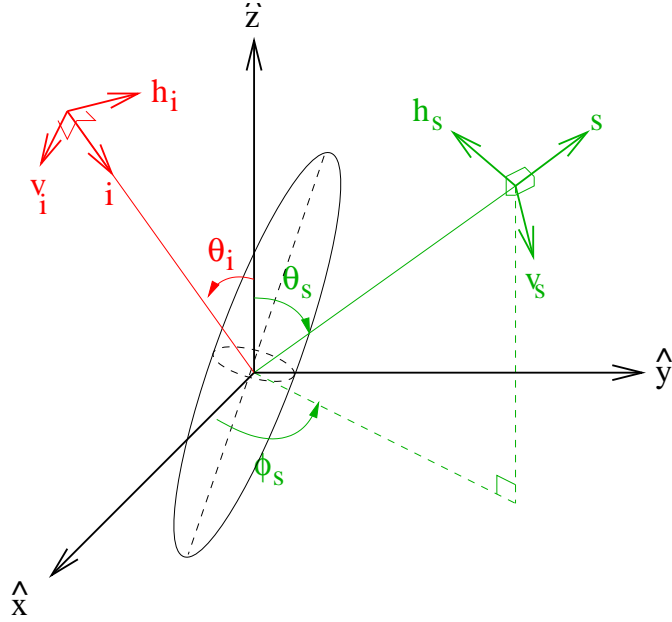
FIG. IV.1 – Définition dans le repère global des vecteurs incidents et diffusés sur un ellipsoïde orienté aléatoirement dans le cas de la convention FSA (Forward Scattering Alignment).
