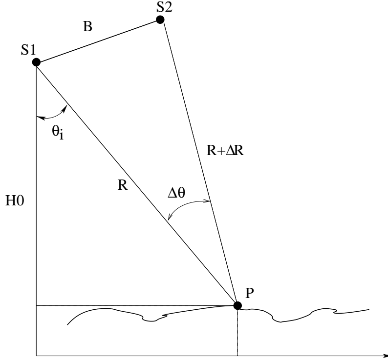
FIG. II.9 – Configuration géométrique pour l'interférométrie.
