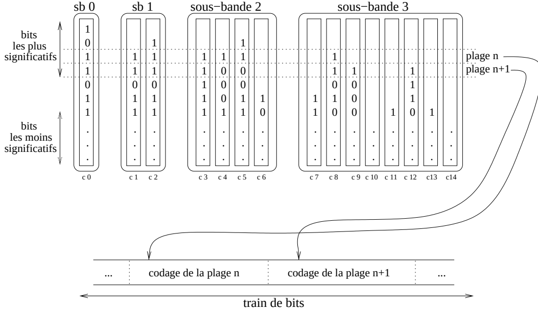
FIG. 2.15 – Illustration du codage en plan de bits
