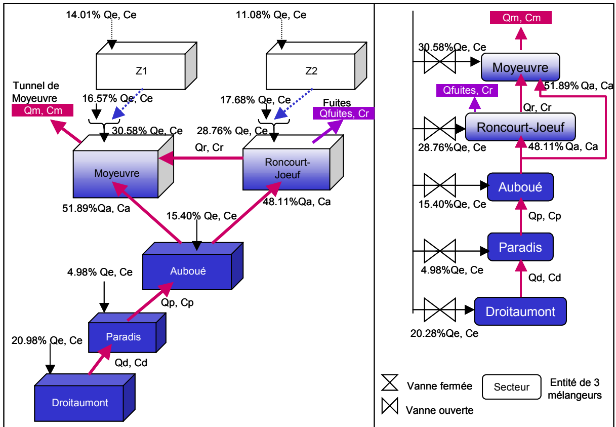
Figure 5.10. Quatrième phase de fonctionnement du bassin Sud : Remplissage de Roncourt-Joeuf et de Moyeuvre
