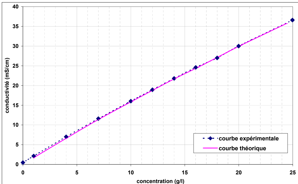
Figure 2.16. Courbe d'étalonnage
