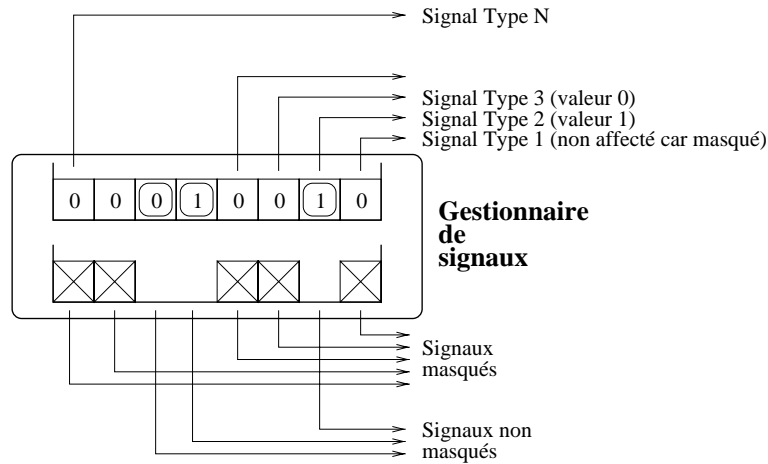
FIG. 3.9: Le gestionnaire de signaux.
