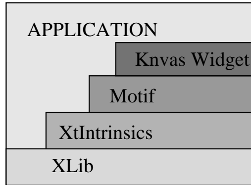
FIG. 4.3: Les niveaux d'abstraction de l'application.
