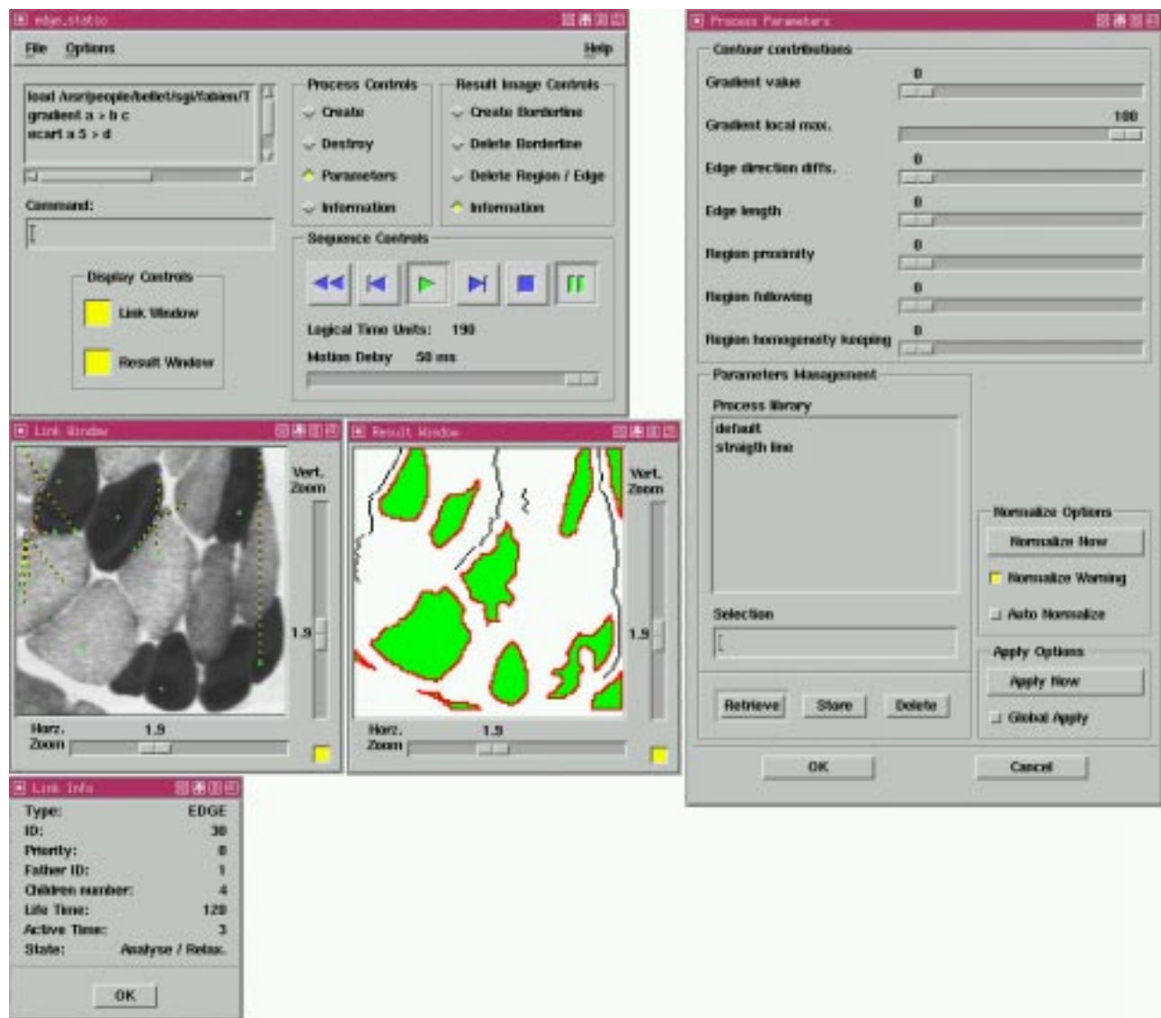
FIG. 4.1: Vue globale du système de segmentation : la fenêtre principale est edge.static , elle contient les contrôles de séquençement ; Link Window présente les relations de parenté entre les processus ; Result Window montre les résultats courants de la segmentation ; Link Info indique les caractéristiques d'un certain processus qui a été sélectionné par l'utilisateur et Process Parameters offre un accès à un panneau permettant de contrôler les comportements d'un processus de segmentation.
