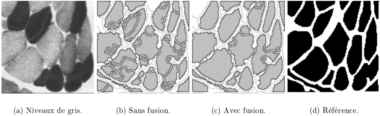
FIG. 5.42: Influence de la fusion des primitives région sur le résultat final. (a) L'image en niveaux de gris est une partie de l'image cellules256.gif . (b) Les primitives régions ne fusionnent pas entre elles. La mesure de Vinet de ce résultat vaut V_1 = 0.334 . (c) Les primitives régions fusionnent dynamiquement au cours de leur construction. La mesure de Vinet de ce résultat de ce résultat vaut V_2 = 0.184 . (d) La carte des régions de référence.
