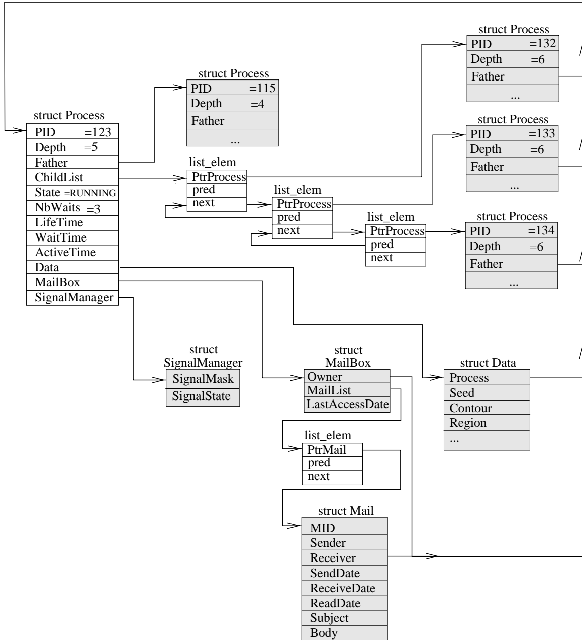
FIG. 3.2: Les données de séquençement d'un processus.
