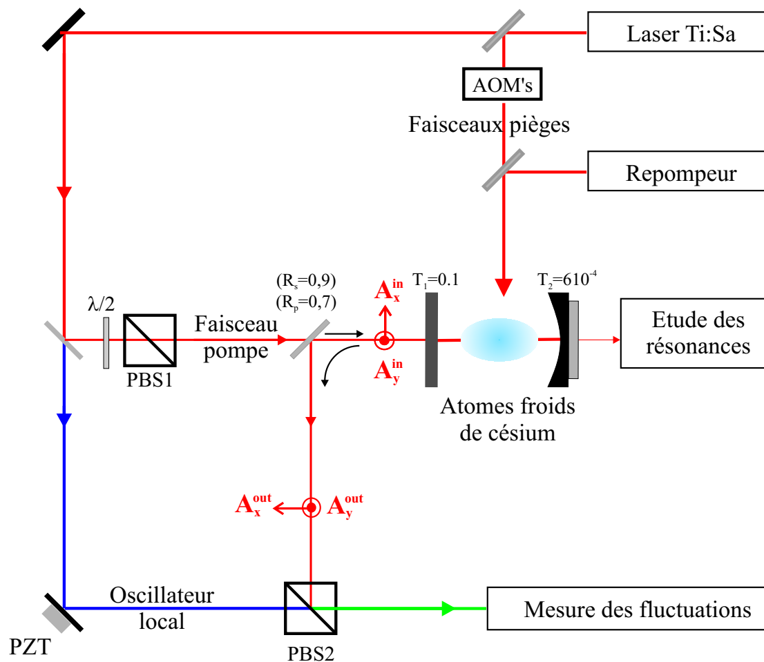
Fig. 2.6 – Schéma de principe de la configuration expérimentale.
