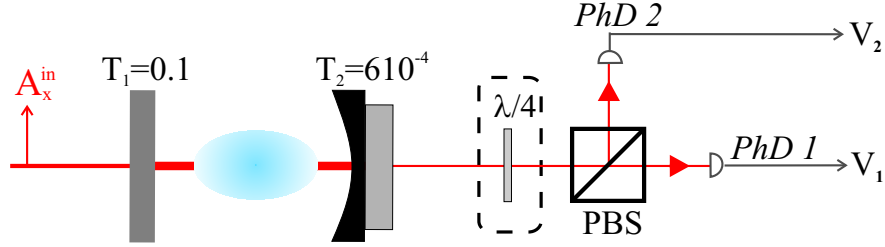
Fig. 2.7 – Dispositif expérimental pour l'analyse de la polarisation transmise par la cavité. Si la lame quart d'onde est enlevée, les photodiodes PhD 1 et PhD 2 mesurent les intensités des modes polarisés horizontalement et verticalement. Si la lame quart d'onde est tournée de 45^\circ , alors ces photodiodes mesurent les intensités des modes polarisés circulairement.
