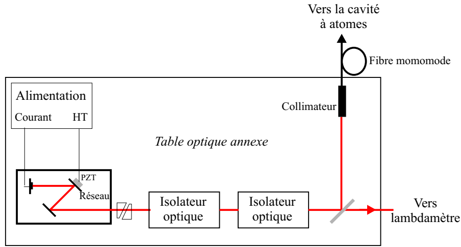
Fig. 3.9 – Montage de la diode laser auxiliaire sur réseau. Le faisceau est envoyé vers la cavité à l'aide d'une fibre monomode.
