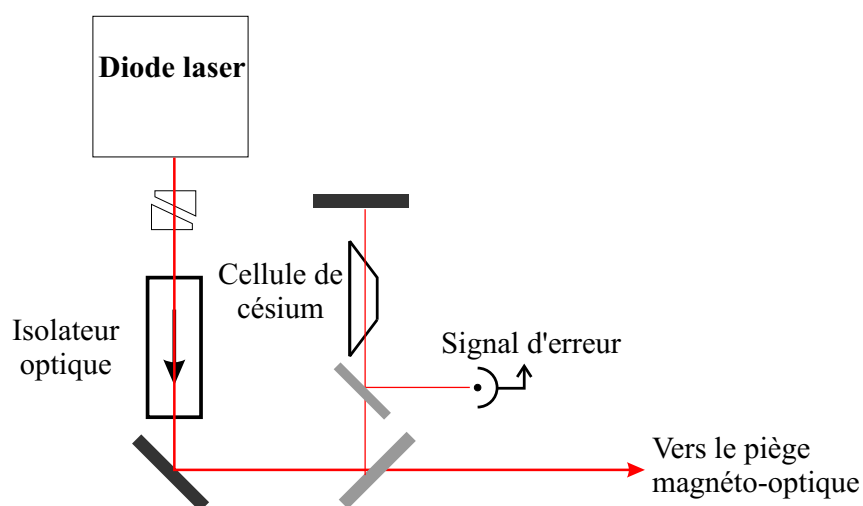
Fig. 2.5 – Asservissement de la diode de repompage par absorption saturée.
