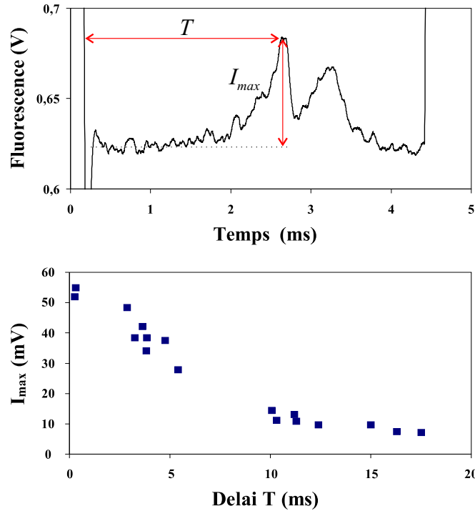
Fig. 3.4 – Fluorescence du nuage atomique due au faisceau pompe. Courbe (a): résonance de la cavité. Courbe (b): évolution de l'intensité maximale de fluorescence de la pompe en fonction du temps T , compté à partir de la coupure des faisceaux pièges.
