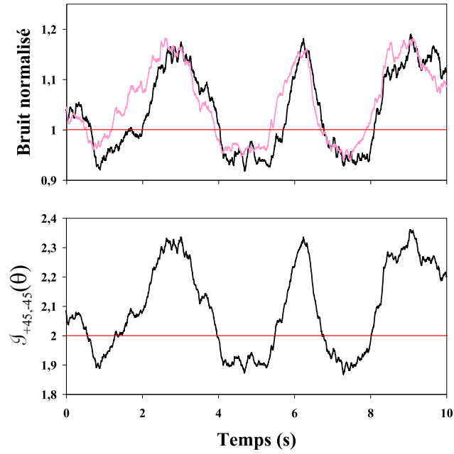
Fig. 5.11 – Mesure de l'intrication des modes polarisés à 45^\circ . La courbe (a) donne les spectres de bruit des modes x et iy . La somme de ces bruits correspond à \mathcal{J}_{+45,-45}(\theta) (courbe (b)). La fréquence d'analyse vaut 5\text{ MHz} et la puissance incidente 7\text{ }\mu\text{W} .
