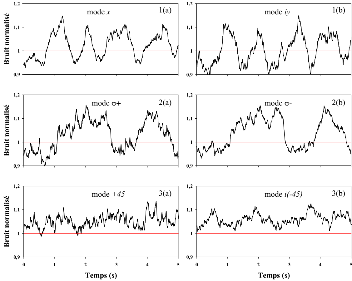
Fig. 5.13 – Bruits normalisées à la fréquence d'analyse de 5 MHz. La cale piézo-électrique de l'oscillateur local est modulée dans la temps, ce qui balaie la phase des quadratures de bruit mesurées. La vitesse de balayage est différente pour les enregistrements 1, 2 et 3. Courbes 1(a) et (b): modes A_x et A_y . Courbes 2(a) et (b): modes A_{\sigma_+} et A_{\sigma_-} . Courbes 3(a) et (b): modes A_{+45^\circ} et A_{-45^\circ} . Les modes x , y , \sigma_+ , \sigma_- sont comprimés tandis que les modes à 45^\circ présentent un excès de bruit. Les spectres de bruits (a) et (b) sont enregistrés en même temps: à chaque instant, la quadrature mesurée sur les deux spectres est la même.
