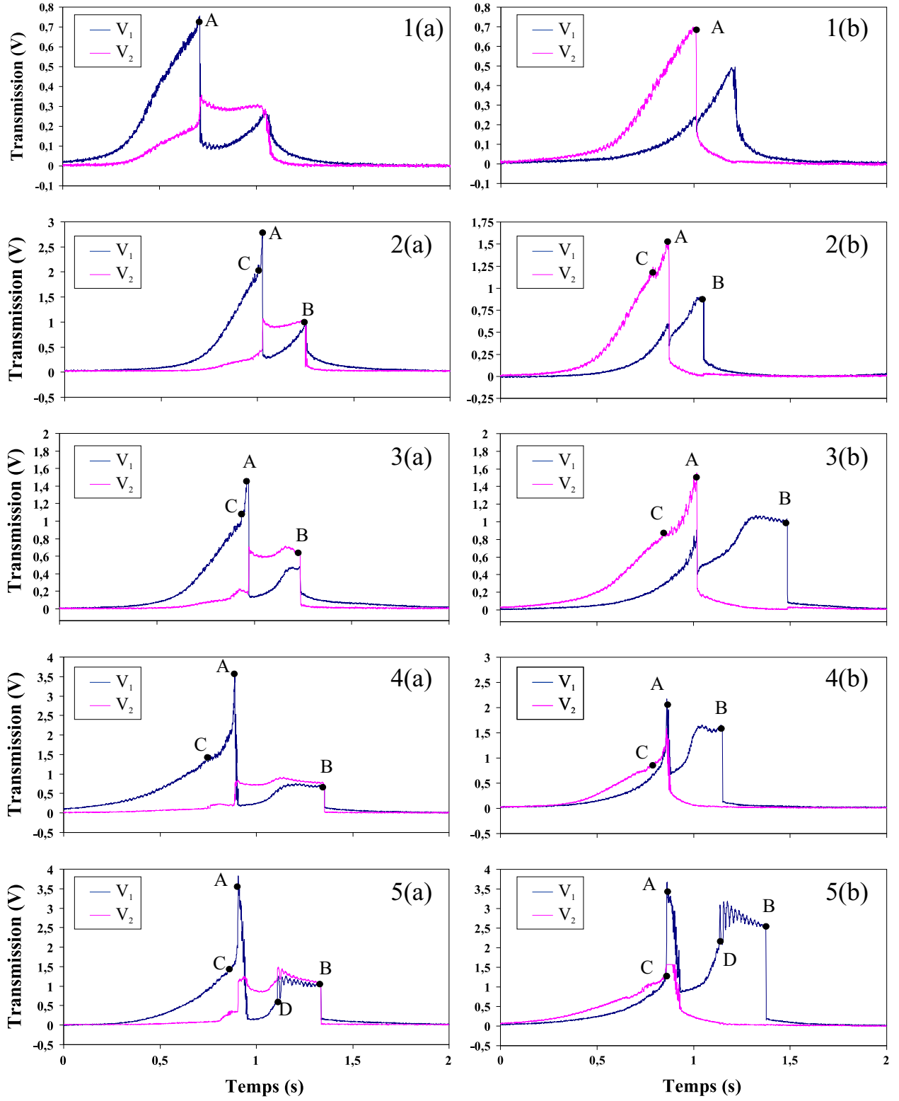
Fig. 2.13 – Evolution des courbes de résonance en fonction de l'intensité. Les courbes (a) et (b) représentent l'analyse linéaire et circulaire respectivement. La puissance des pièges vaut P_{\text{pièges}} = 10 \text{ mW} et le paramètre de saturation est s_{\text{pièges}} \simeq 2 . Courbes 1): P_{\text{in}} = 7 \text{ } \mu\text{W} , s_{\text{pompe}}^{\text{max}} \simeq 0.3 ; 2): P_{\text{in}} = 14 \text{ } \mu\text{W} , s_{\text{pompe}}^{\text{max}} = 0.6 ; 3): P_{\text{in}} = 21 \text{ } \mu\text{W} , s_{\text{pompe}}^{\text{max}} = 0.9 ; 4): P_{\text{in}} = 28 \text{ } \mu\text{W} , s_{\text{pompe}}^{\text{max}} = 1.2 ; 5): P_{\text{in}} = 42 \text{ } \mu\text{W} , s_{\text{pompe}}^{\text{max}} = 0.35 .
