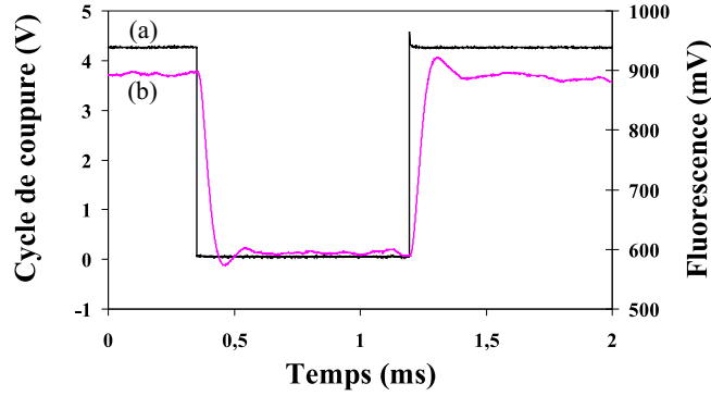
Fig. 3.3 – Fluorescence du nuage atomique due aux faisceaux pièges. Courbe (a): tension de commande de la coupure des faisceaux pièges: V_{cycle} . Courbe (b): tension de sortie de la photodiode enregistrant la fluorescence des atomes. La puissance totale des faisceaux pièges est de l'ordre de 5 mW. résonance de la cavité. Courbe (b): évolution de l'intensité maximale de fluorescence de la pompe en fonction du temps T , compté à partir de la coupure des faisceaux pièges.
