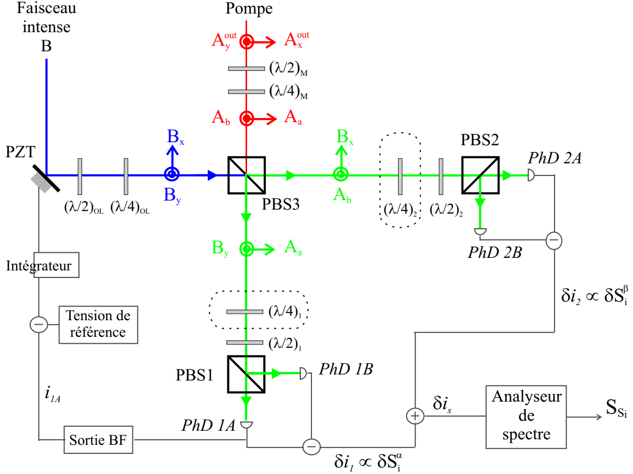
Fig. 5.21 – Dispositif de mesure de l'intrication en polarisation. Les lames quart d'onde (\lambda/4)_{1,2} et demi-onde (\lambda/2)_{1,2} sont ajustées pour mesurer les paramètres de Stokes S_2^{\alpha,\beta} et S_3^{\alpha,\beta} . Le signal d'interférence de la photodiode 1A est utilisé pour asservir la phase du faisceau B.
