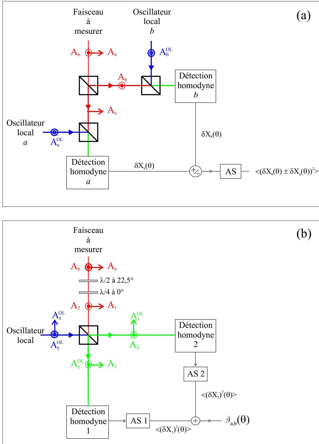
Fig. 5.8 – En haut: principe de mesure des corrélations en séparant spatialement les modes a et b dont on veut estimer \mathcal{I}_{a,b} . Cette méthode suppose deux mesures successives. En bas: mesure directe du critère de non-séparabilité selon la méthode décrite dans le texte.
