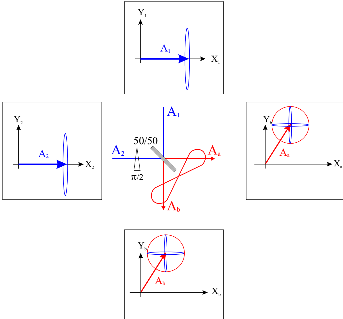
Fig. 5.2 – Génération de faisceaux intriqués en combinant deux faisceaux 1 et 2 comprimés sur une lame séparatrice 50/50. Ces faisceaux sont comprimés en amplitude (quadrature X ). Si on introduit un déphasage de \pi/2 entre les deux bras, alors les faisceaux sortant sont intriqués.
