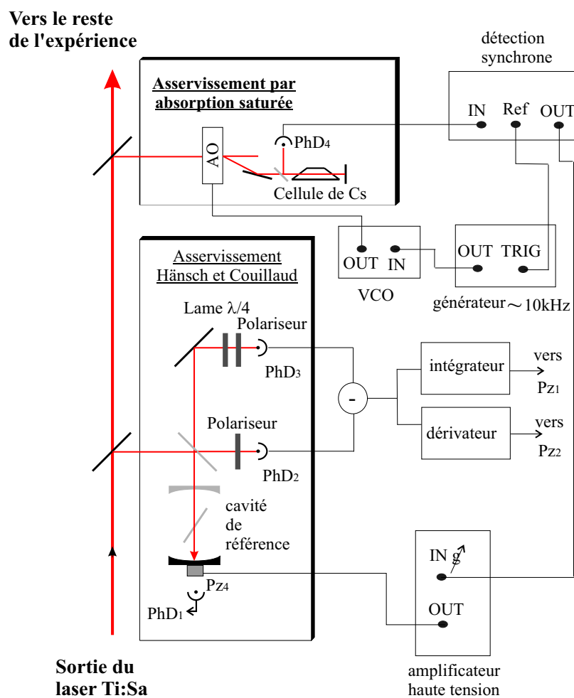
Fig. 2.2 – Asservissement du laser Titane:saphir sur une cavité de référence et asservissement de cette cavité d'absorption saturée.
