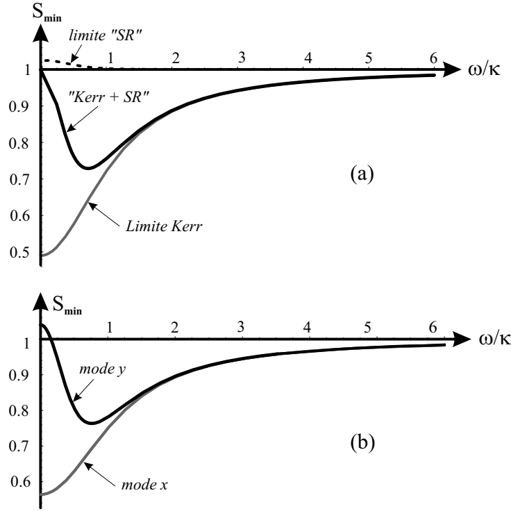
Fig. 4.9 – Figure (a): spectre de bruit minimal du mode vide A_y^{\text{out}} donné par les termes basse fréquence "SR" (trait pointillé), par les termes hautes fréquences Kerr (trait grisé) et par les deux effets combinés (trait noir). D'apparence négligeable sur cette figure, puisque l'on a représenté le spectre de bruit minimal, les termes "SR" sont en fait associés à un important excès de bruit sur les autres quadratures. Cet excès de bruit provoque une remontée du bruit à basse fréquence. Par ailleurs, on note que le spectre de bruit minimal donné par la limite Kerr (trait grisé) correspond également au spectre de bruit minimal du champ moyen A_x^{\text{out}} . Figure (b): spectre de bruit des modes A_y^{\text{out}} (trait noir) et A_x^{\text{out}} (trait grisé) calculés par un traitement numérique complet des fluctuations. Les paramètres valent: \delta_0 = 5 , \Delta = 20\gamma , \gamma/\gamma_{\perp} = 3 , \kappa = 2\gamma , s_{\max} = 0.1 , \delta_{\text{cav}} = 4.6 . Le point de fonctionnement est proche du seuil de bascule de la polarisation et correspond au point A représenté sur la figure 4.11.
