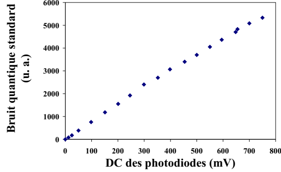
Fig. 2.18 – Evolution du bruit quantique standard à la fréquence de 4 MHz en fonction de la puissance de l'oscillateur local.
