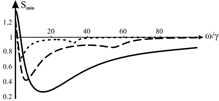
Fig. 4.13 – Spectres de bruit minimal pour différentes valeurs du rapport \rho = \kappa/\gamma (pointillé: \rho = 2 , tireté: \rho = 10 , plein: \rho = 50 ). Pour chaque valeur de \rho , le paramètre de saturation s_{max} est optimisé. Les paramètres correspondent à: \delta_0 = 5 , \Delta = 20\gamma , \gamma/\gamma_\perp = 3 .
