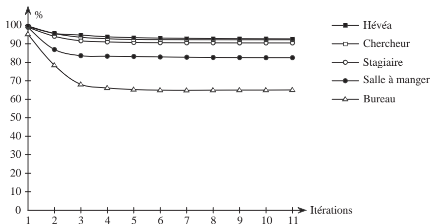
FIG. 3.3 – Proportion des liens pour lesquels BF ne d passe pas \epsilon .
