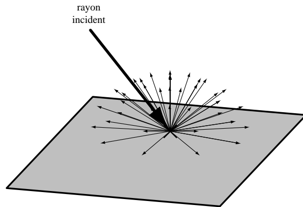
FIG. 2.2 – Loi de réflexion de Lambert : surfaces diffuses.
