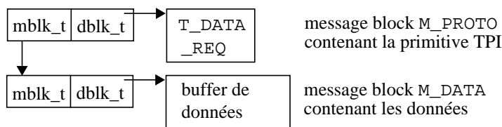
Figure 9: Message TPI contenant une requête de transmission de données.
