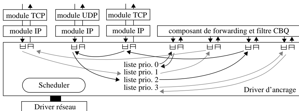
Figure 15: Extension QoS de la pile TCP/IP démultiplexée sous Streams.
