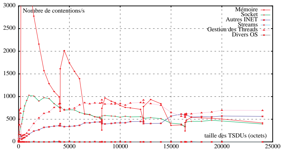
Figure 22: Contentions pour la pile BSD, 4 connexions, quadri-processeur.
