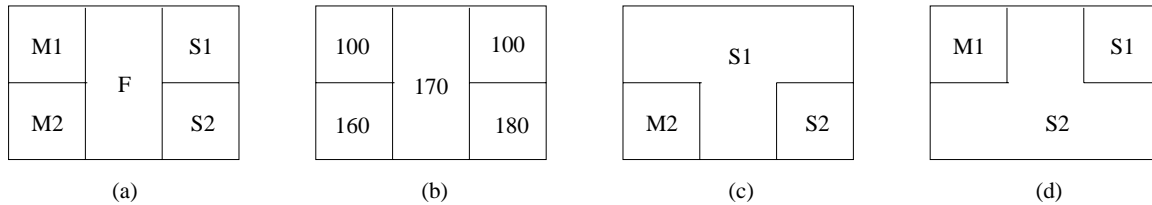
FIG. 5.6 - (a) Des régions \Gamma (b) leurs niveaux de gris et (c-d) deux configurations possibles résultant de la validation des arêtes floues.
