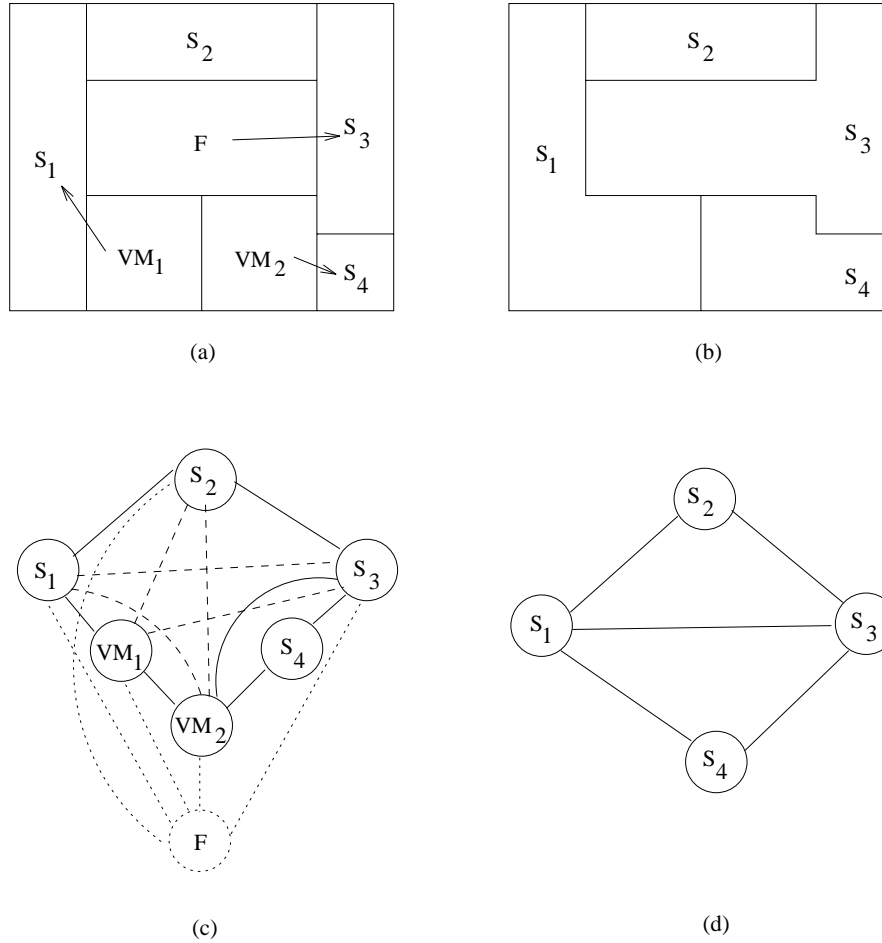
FIG. 5.23 - La configuration montrée en (b) résulte de celle de (a) après les fusions des sommets VM_1 avec S_1 , VM_2 avec S_4 et F avec S_3 . La clique floue d'ordre 5 de (c) donne lieu aux adjacences réelles montrées en (d).
