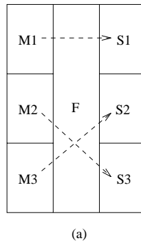
FIG. 5.9 - Trois arêtes floues qui s'interdisent mutuellement.
