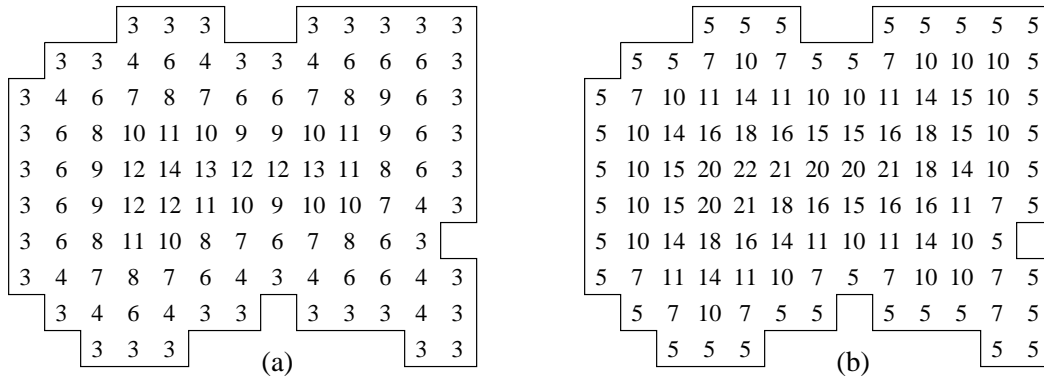
FIG. 10 - DM pour (a) d_{3,4} et (b) d_{5,7,11}
