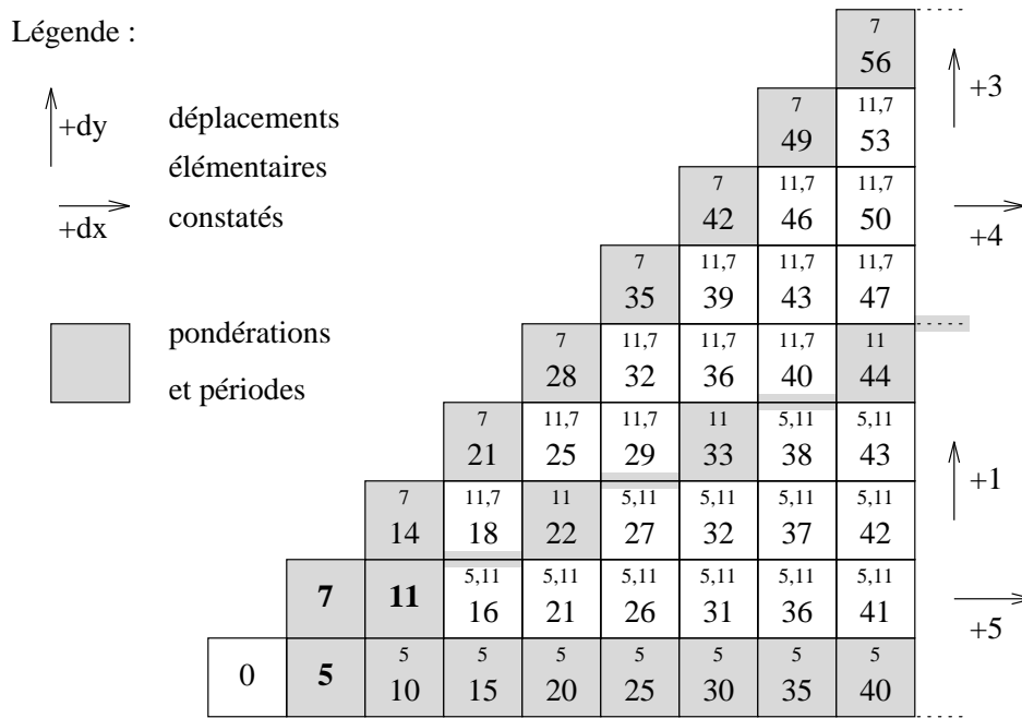
FIG. 21 - Cônes d'influence de chanfrein 5, 7, 11
