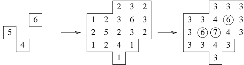
FIG. 51 - Image de poids, image reconstruite, DM et AM pour d_{3,4}
