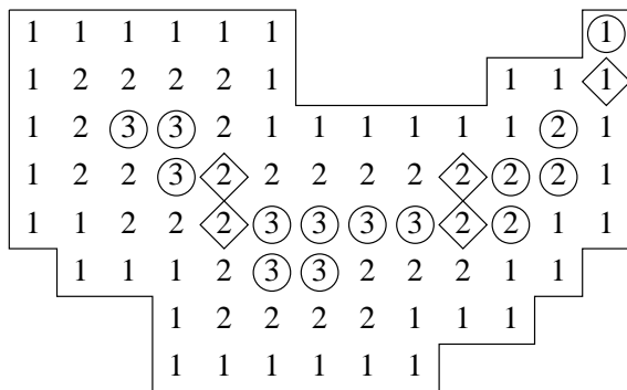
FIG. 55 - Carte de distance d_8 , axe médian (cercles) et points selle (losanges) de types 2, 3, 1 de gauche à droite
