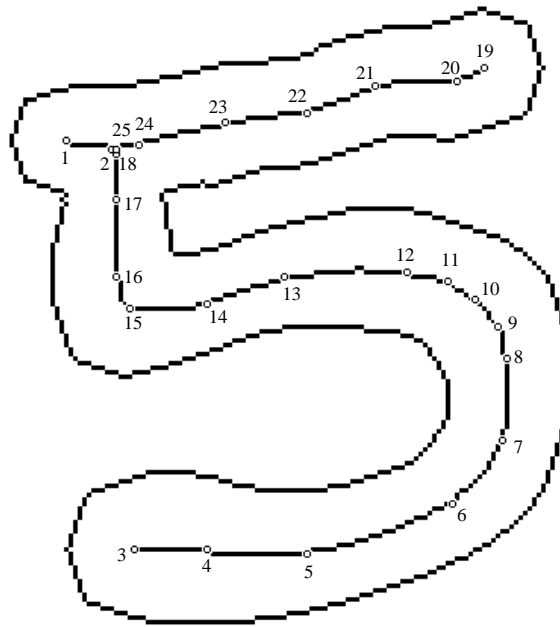
FIG. 64 - Partition du squelette pour d_{3,4} et \theta = 1.5 . Les sommets sont numérotés.
