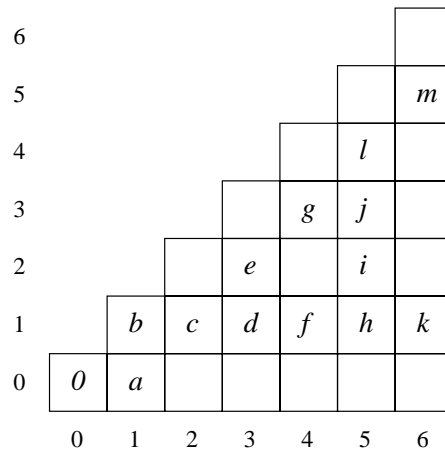
FIG. 19 - Noms des Points visibles (pour x \leq 6 )
