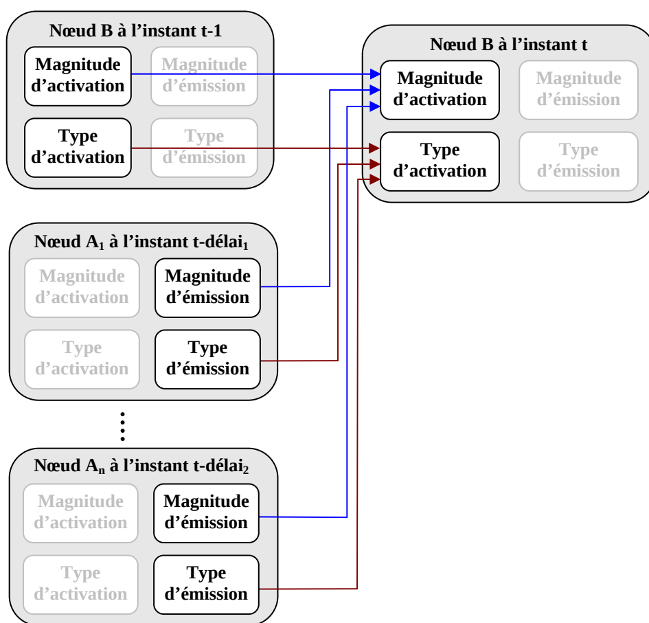
Figure IV.3.3 : Calcul des valeurs d'activation d'un nœud B possédant n parents A_1, \dots, A_n .
