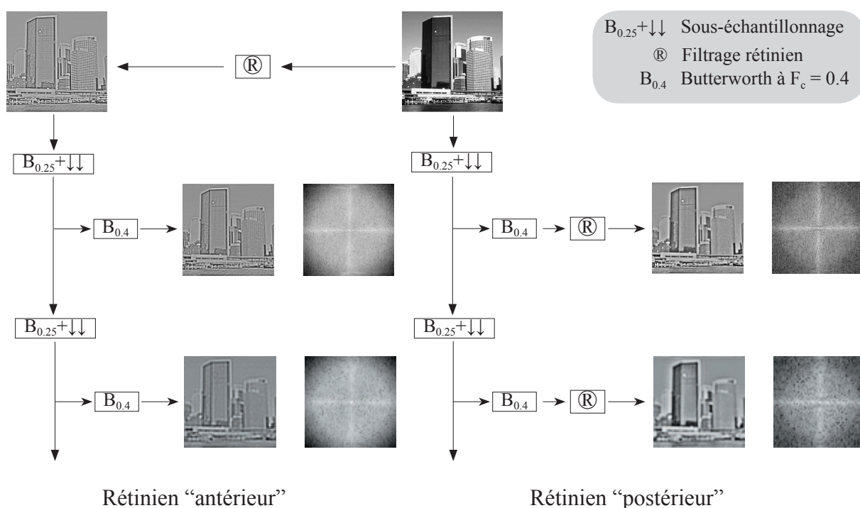
Figure 5.3 : Deux stratégies pour la pyramide incluant le prétraitement rétinien. A chaque niveau est représentée l'image et le logarithme des modules de leurs spectres. Le filtre anti-repliement d'un niveau de la pyramide au suivant est un filtre de Butterworth d'ordre 6 et de fréquence de coupure 0.25. Nous appliquons préférentiellement le "rétinien postérieur".
