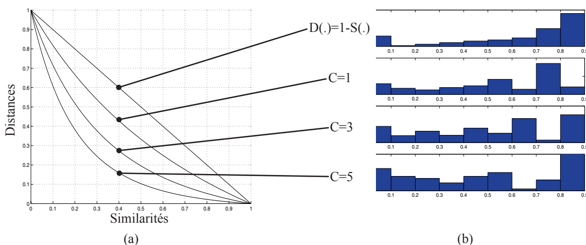
Figure 4.3 : Pour différentes valeurs de C (formule 4.4) (a) passage des similarités aux distances (avec normalisation). (b) Histogramme des distances les plus courtes
